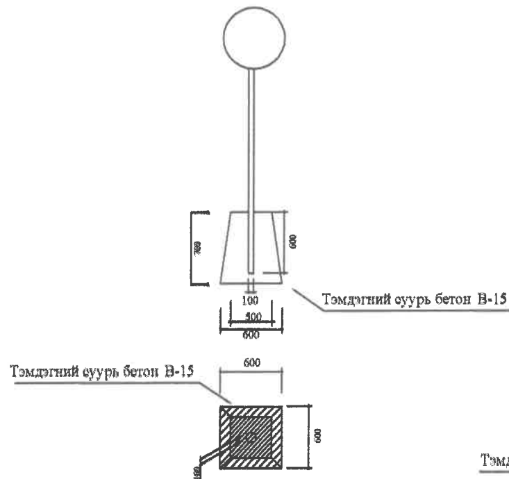
5.18 ХУРД СААРУУЛАГЧ
