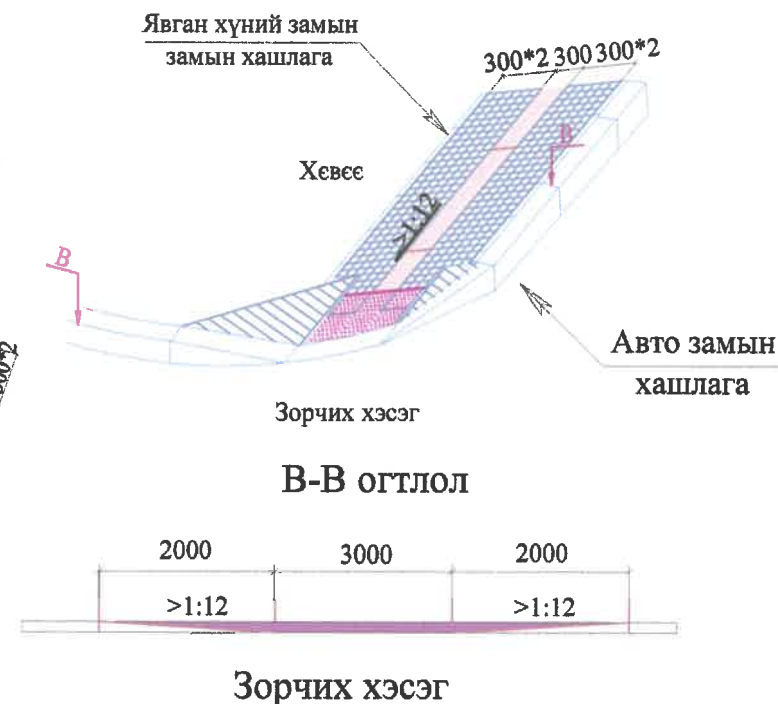
Хараагүй хүний хавтанцар хөтөч зам
