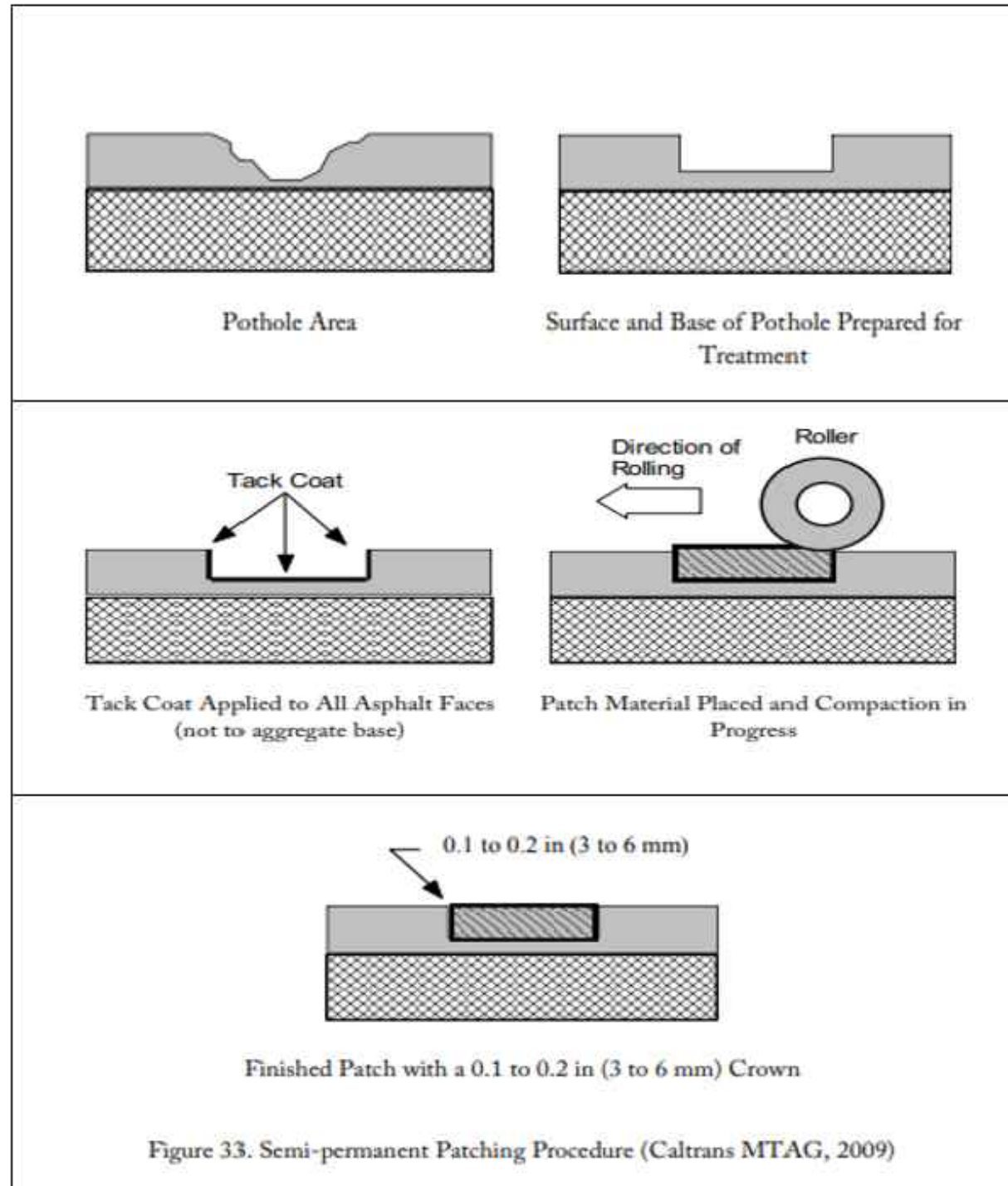
Зураг 1. Нөхөөс хийх схем зураг
