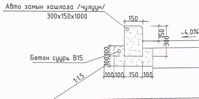
Авто замын хашлага Масштаб 1:20
