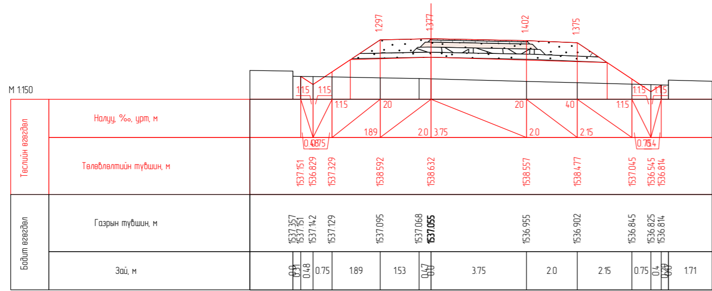
ПК 2-10.00
