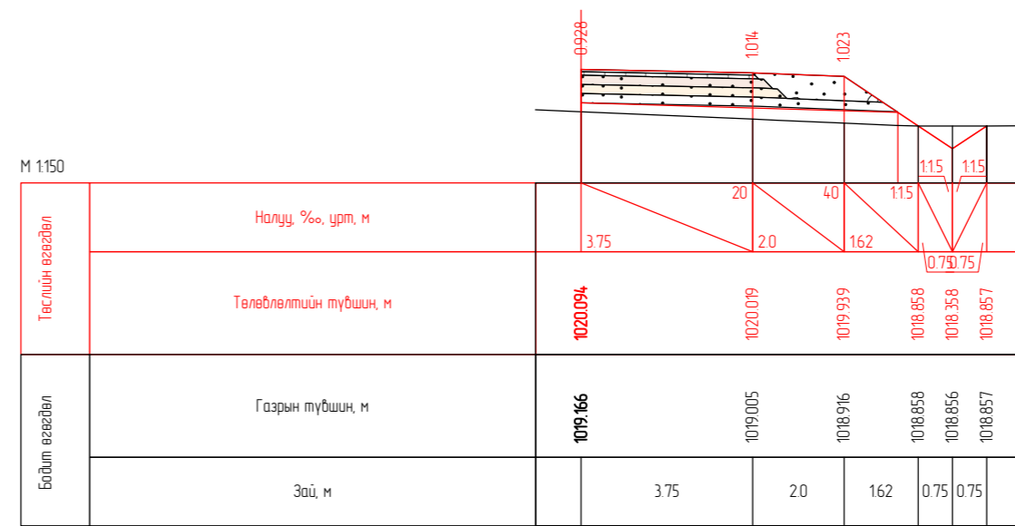
ПК 2+80.00
