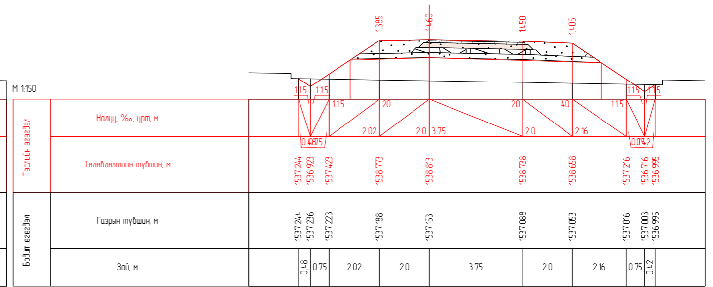
ПК 1-90.00
