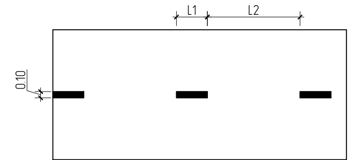
1.15 Тээврийн хэрэгслийн эсрэг урсгалыг тусгаарлах V > 60 \text{ km/h} , L1=3.00-4.00 , L2=9.00-12.00 L1:L2=1:3
