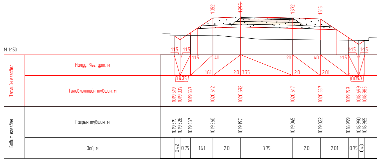
ПК 0+80.00
