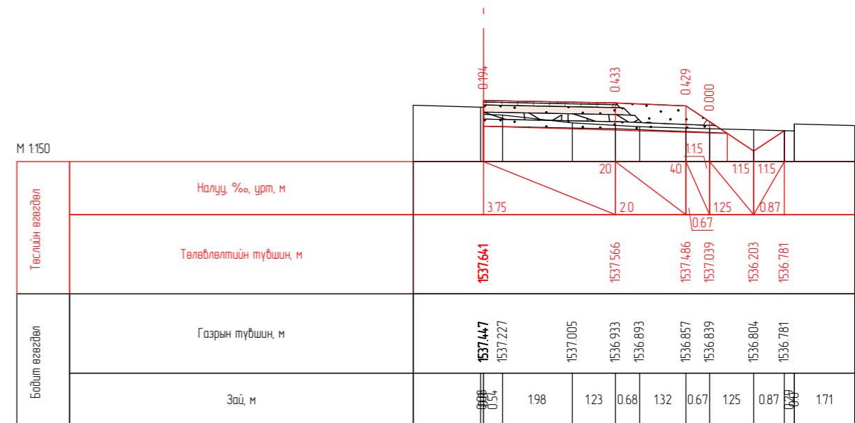
ПК 2-90.00
