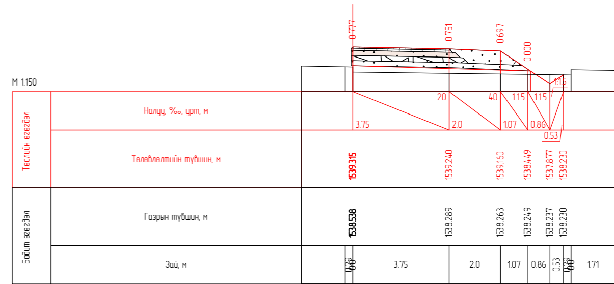
ПК 0+42.78
