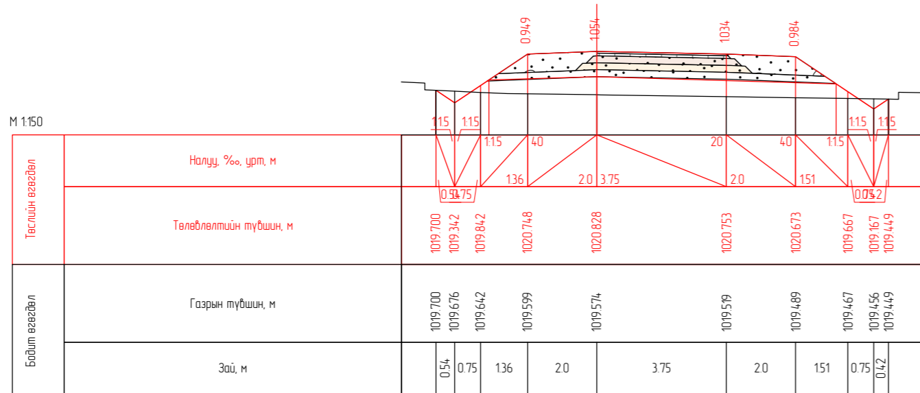
ПК 2+10.00
