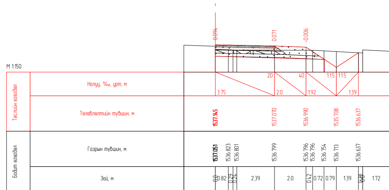
ПК 3+28.39
