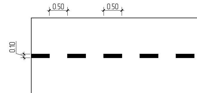
1.17 Чулувар дээрх хөдөлгөөний эгнээг тэмдэглэх
