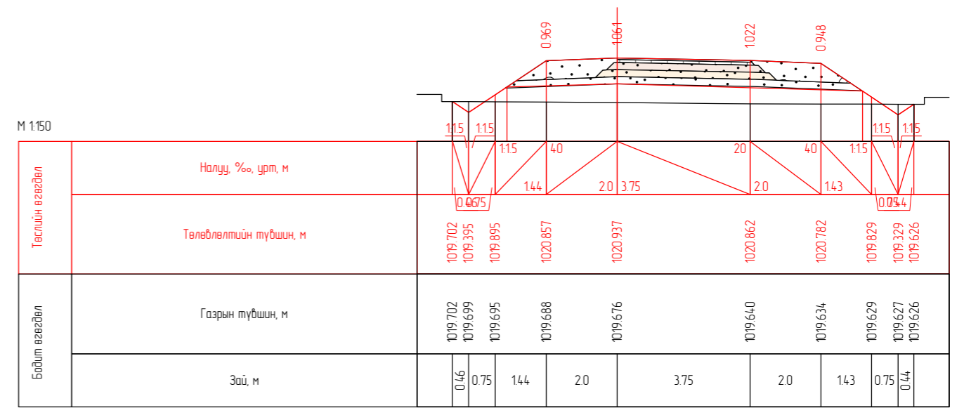
ПК 1+90.00
