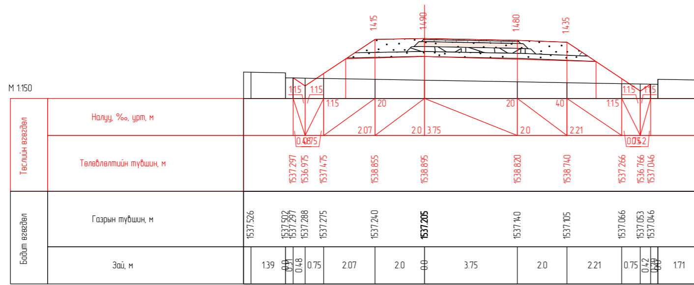
ПК 1-80.00
