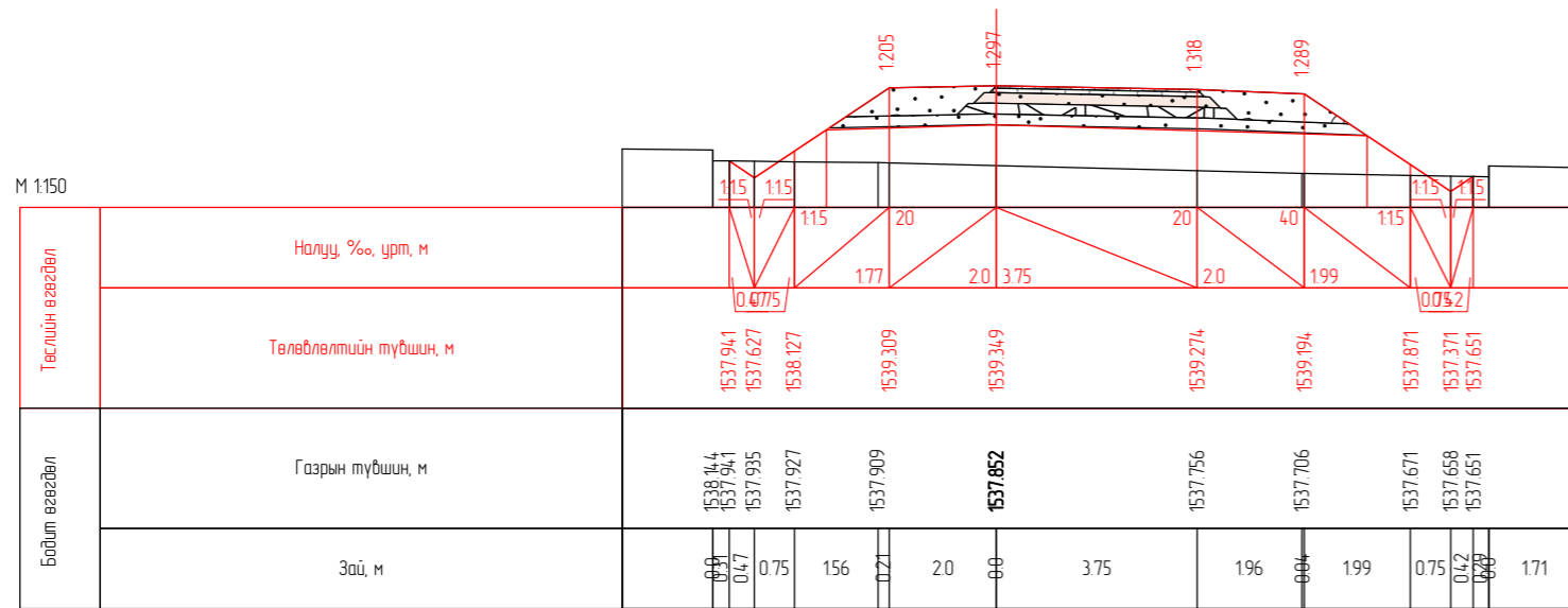
ПК 1+00.00
