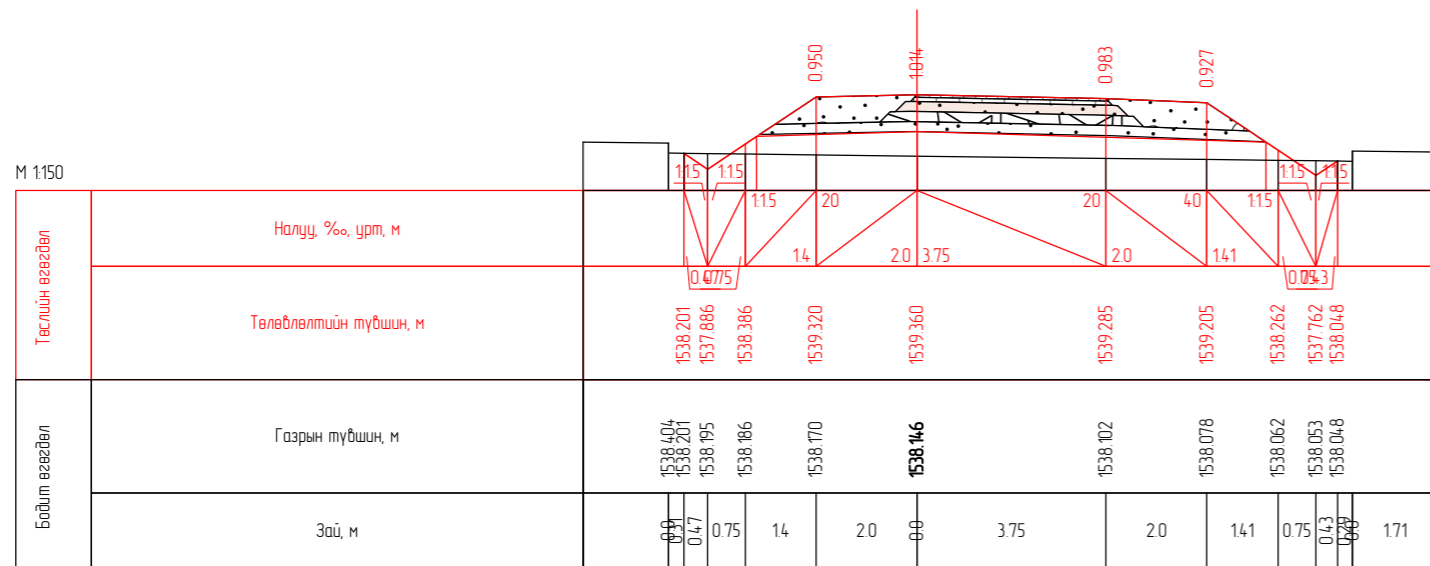
ПК 0+70.00
