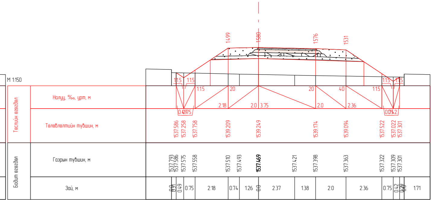
ПК 1+30.00
