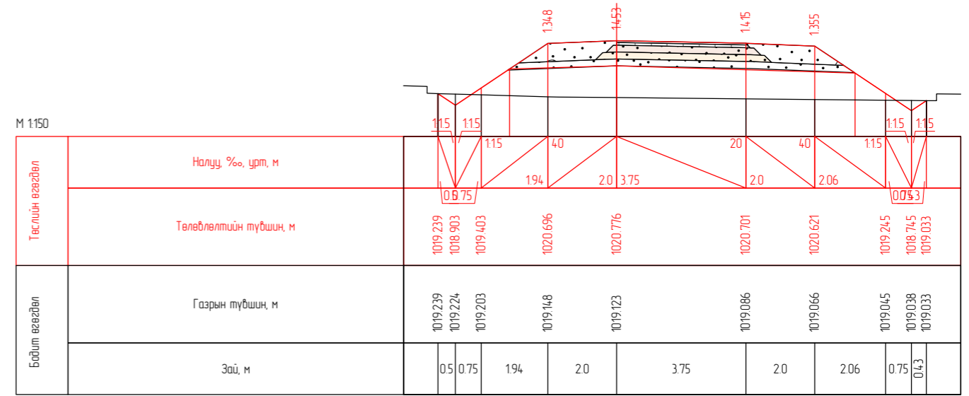
ПК 0+90.00
