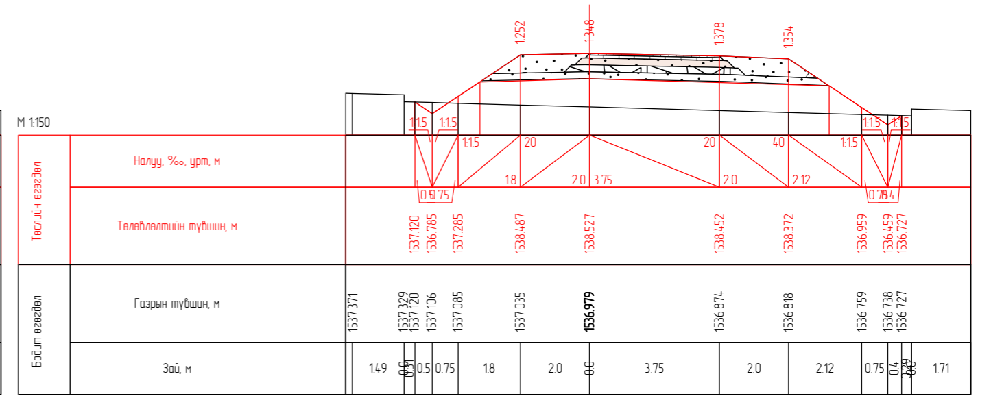
ПК 2-20.00
