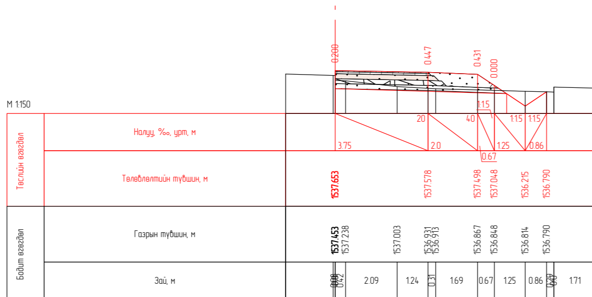
ПК 2-89.11
