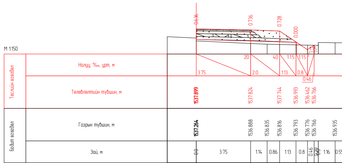
ПК 2-70.00
