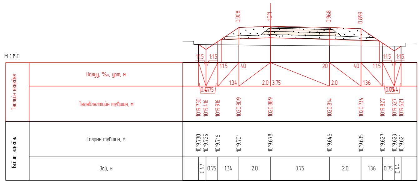
ПК 2+00.00
