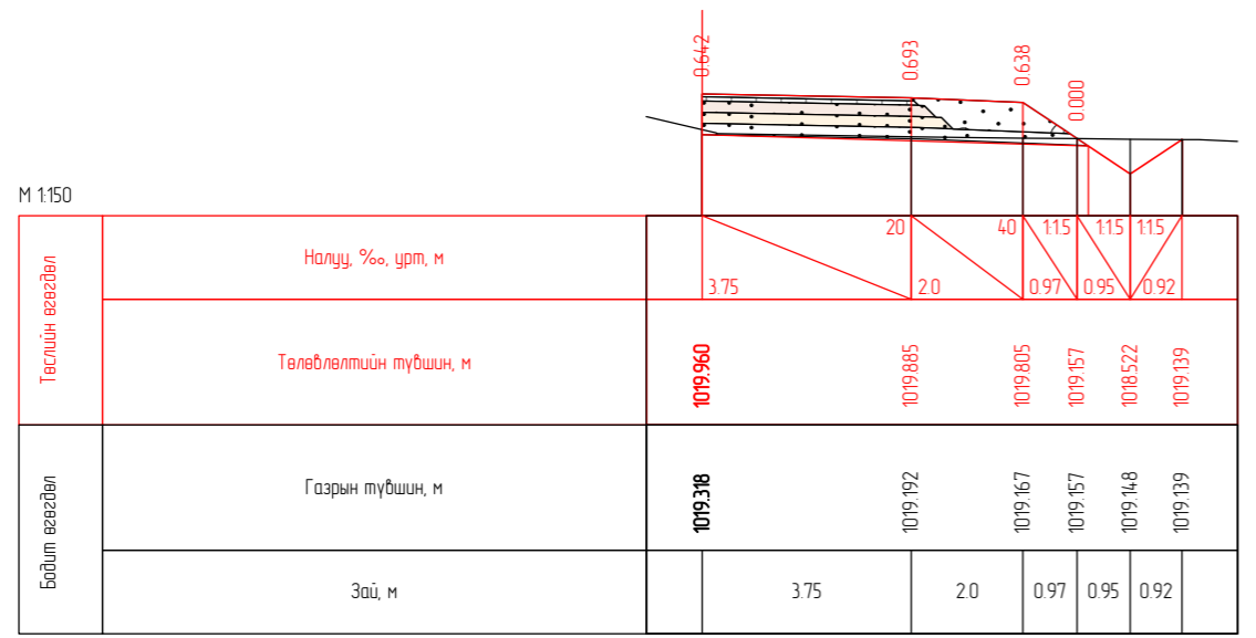
ПК 2+90.84
