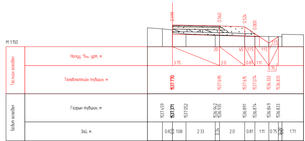
ПК 2-80.00
