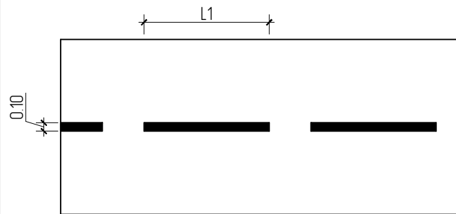
1.16 Үргэлжилсэн шугам ойртож байгааг тэмдэглэх V < 60 \text{ km/h} , L1=3.00-6.00 , L2=1.00-2.00 V > 60 \text{ km/h} , L1=6.00-9.00 , L2=2.00-3.00 L1:L2=3:1
