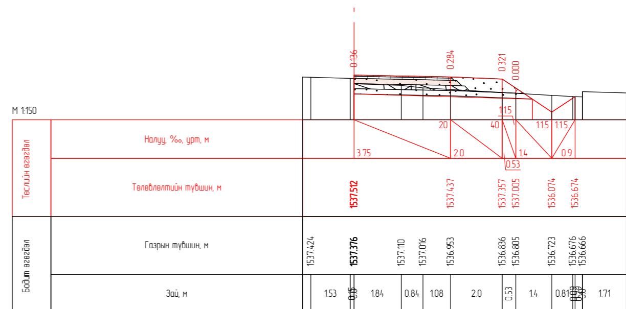
ПК 3+00.00
