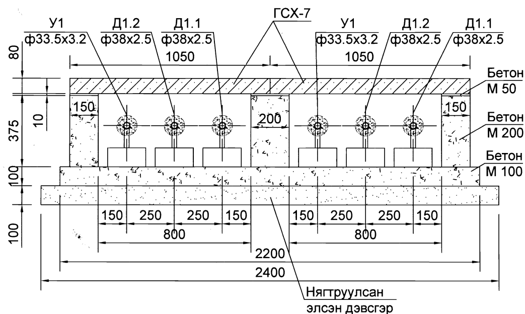
Сувгийн огтлол 19-19 масштаб 1:20
