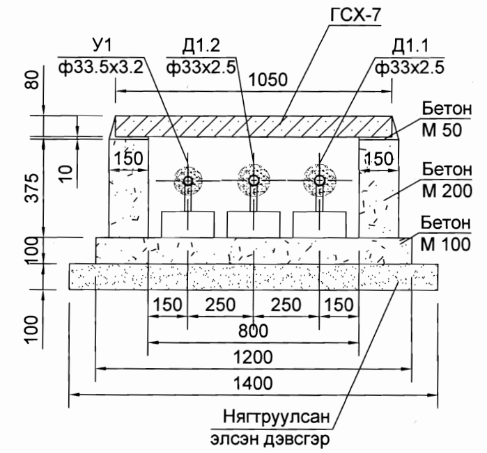
Сувгийн огтлол 16-16 масштаб 1:20
