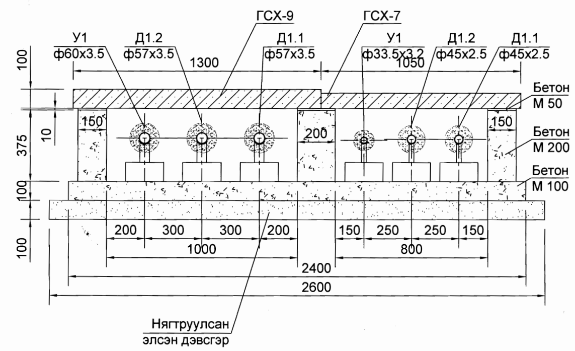
Сувгийн огтлол 17-17 масштаб 1:20
