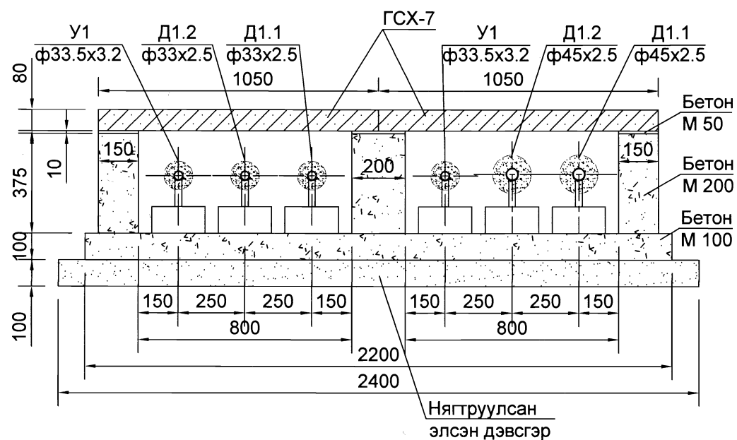
Сувгийн огтлол 18-18 масштаб 1:20
