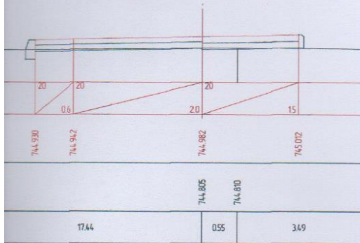
ПК 1+200.00
