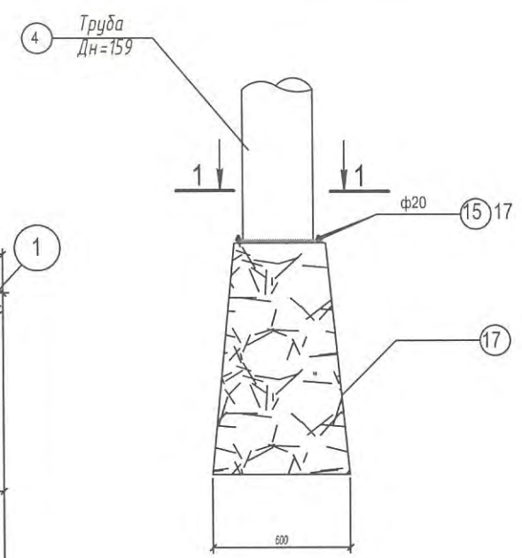
ШОНГИЙН СУУРЬ М 1:10
