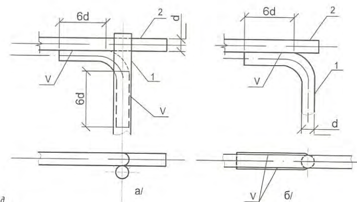
Хэвтээ газардуулагч ба газардуулагч утсыг гагнуураар холбох
