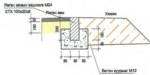
Бүтээц-2 Явган замын хашлага
