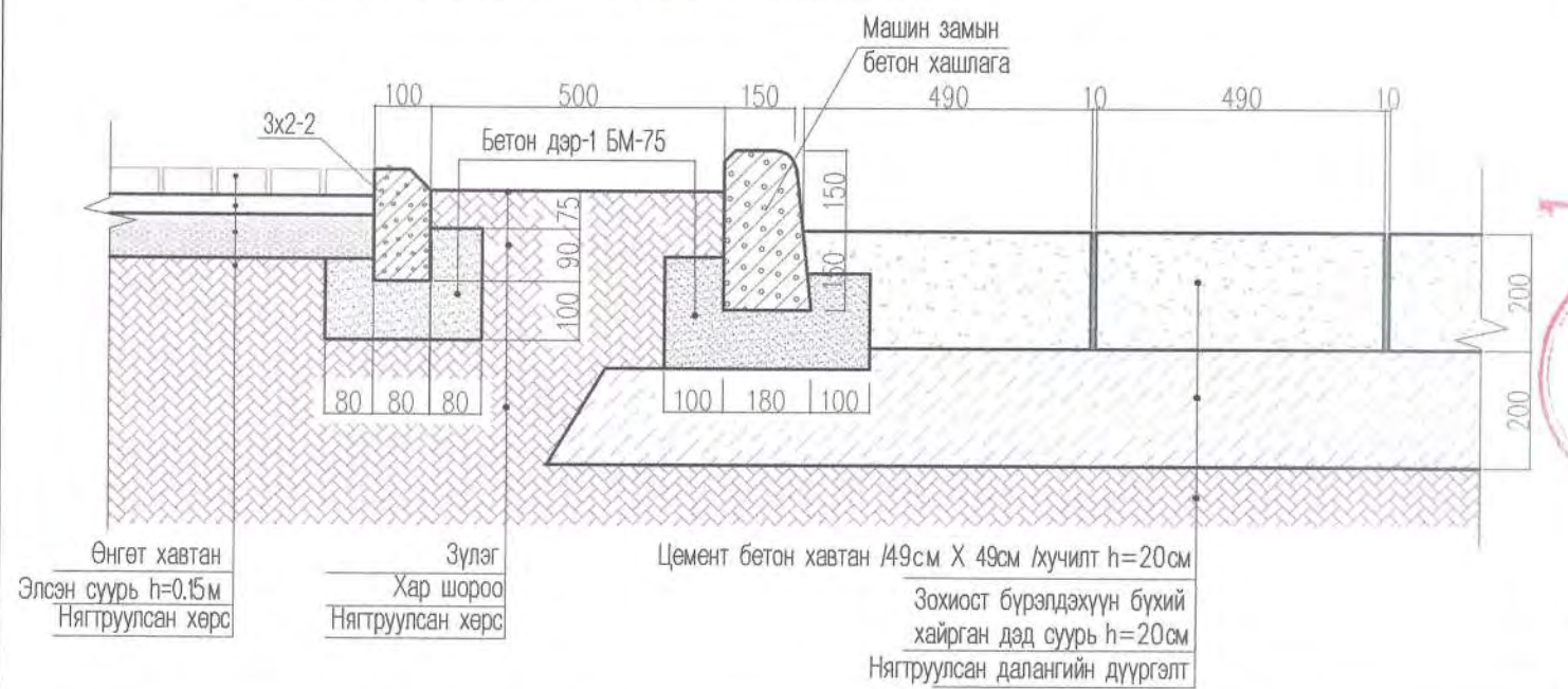
ЯВГАН ХҮНИЙ ЗАМ, ЗУЛЭГ, БЕТОН ХАВТАНТ ЗАМ ОГТЛОЛ 4-4 М1:20
