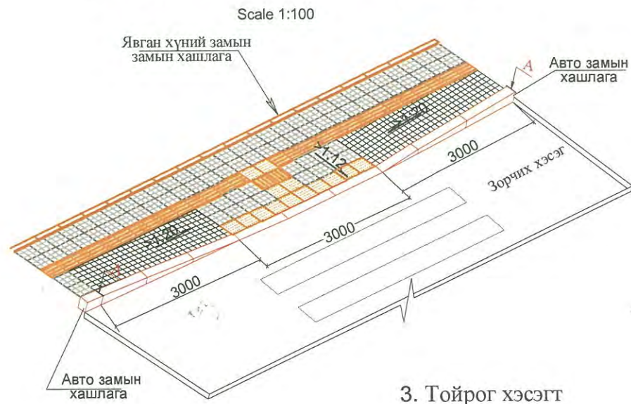
1. Шулуун хэсэгт ногоон байгууламжгүй
