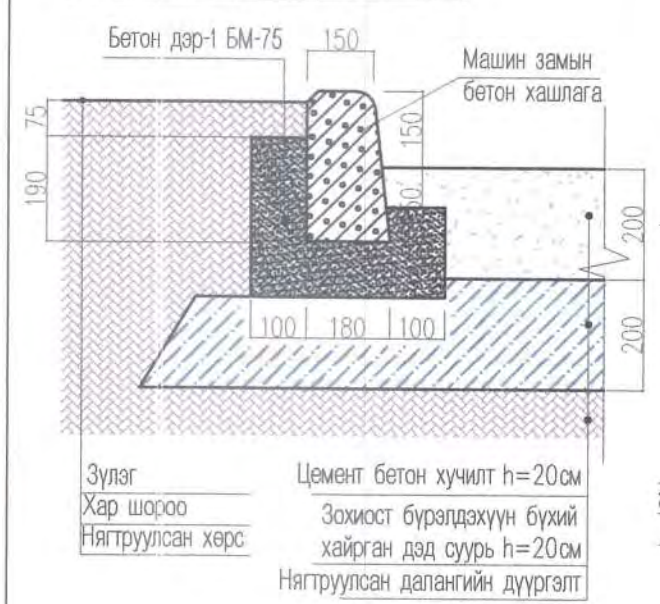
ЯВГАН ХҮНИЙ ЗАМ, ЗУЛЭГ, АВТО ЗАМЫН ОГТЛОЛ 3-3 М1:20
