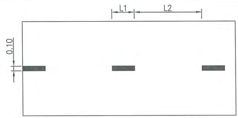
V > 60 \text{ Km/h} , L1 = 3.00 - 4.00 , L2 = 9.00 - 12.00 L1:L2 = 1:3 7.5 Эгнээний хилийг тэмдэглэх
