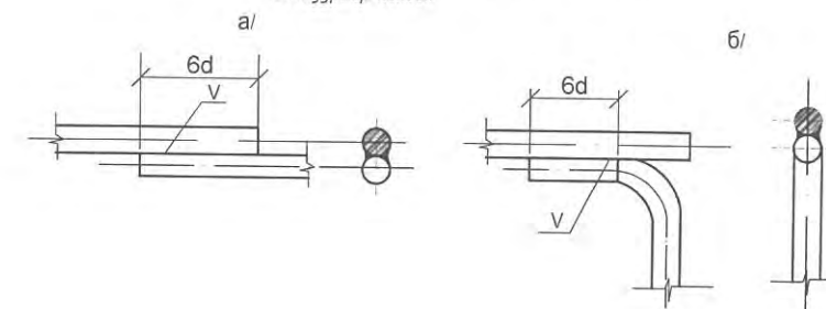
Хэвтээ газардуулагч ба газардуулагч утсыг гагнуураар холбох
