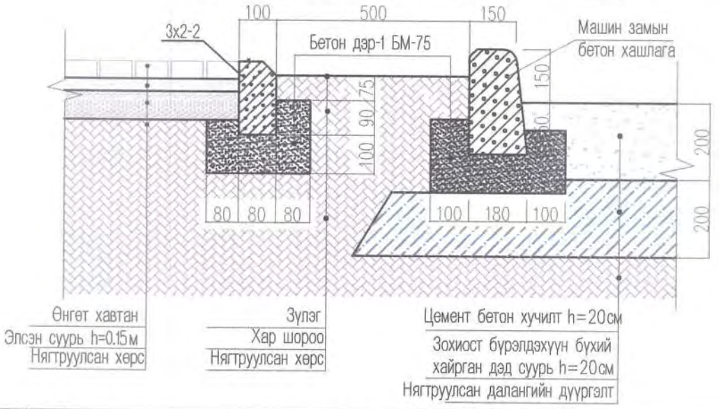
ЯВГАН ХҮНИЙ ЗАМ, ЗУЛЭГ, АВТО ЗАМЫН ОГТЛОЛ 3-3 М1:20
