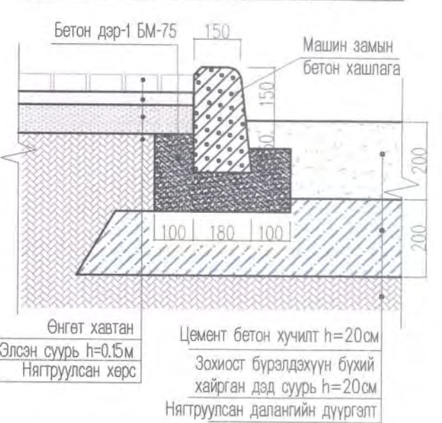
ЯВГАН ХҮНИЙ ЗАМ, ЗУЛЭГ, АВТО ЗАМЫН ОГТЛОЛ 3-3 М1:20
