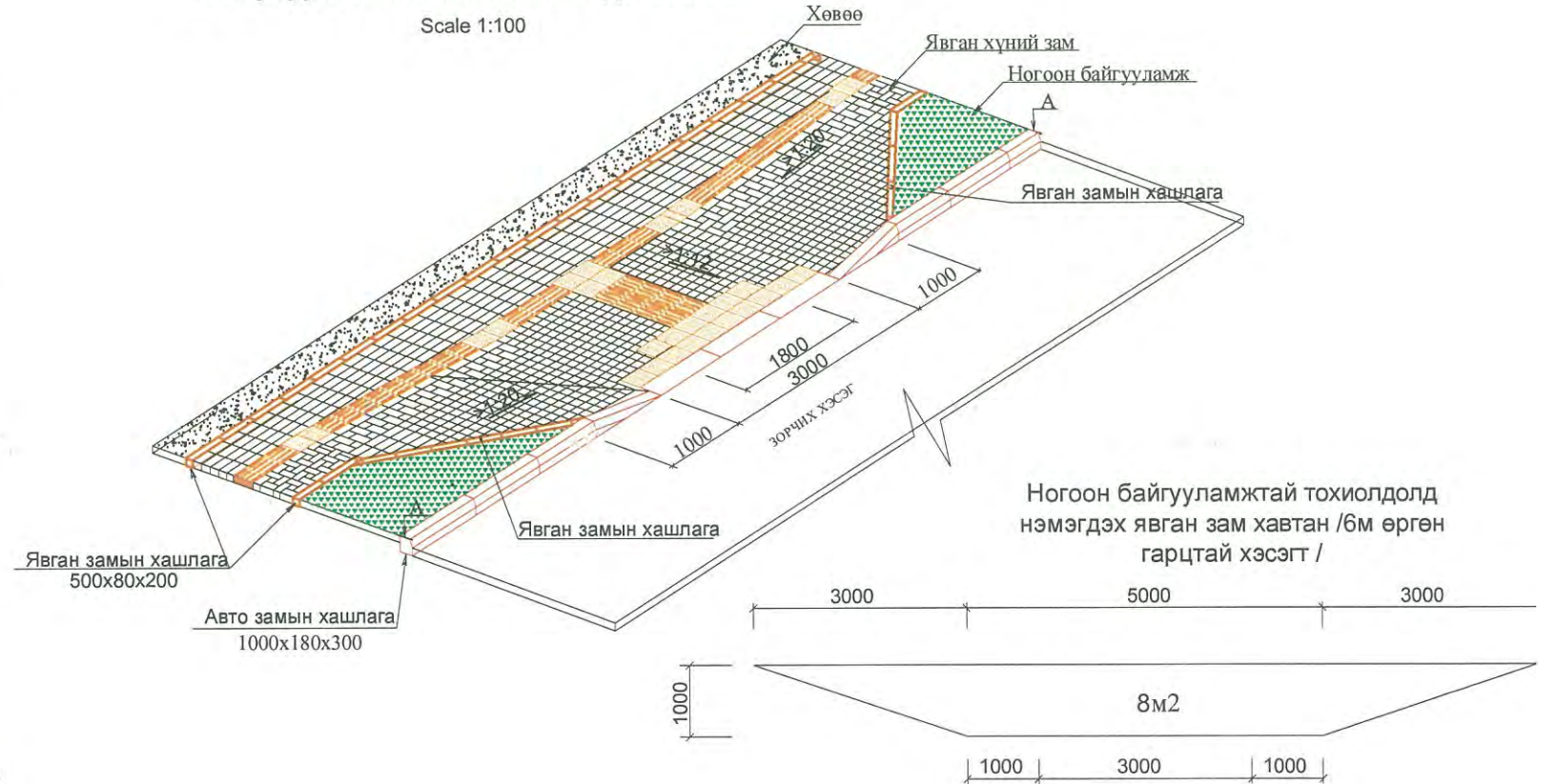
2. Шулуун хэсэгт ногоон байгууламжтай
