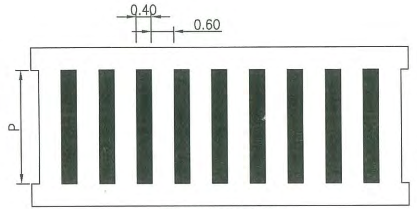
V < 60 \text{ Km/Hr} , P > 2,50 V > 60 \text{ Km/Hr} , P > 4,00 7.13a Явган хүний гарц (Явган хүний зохицуулдаггүй гарц)
