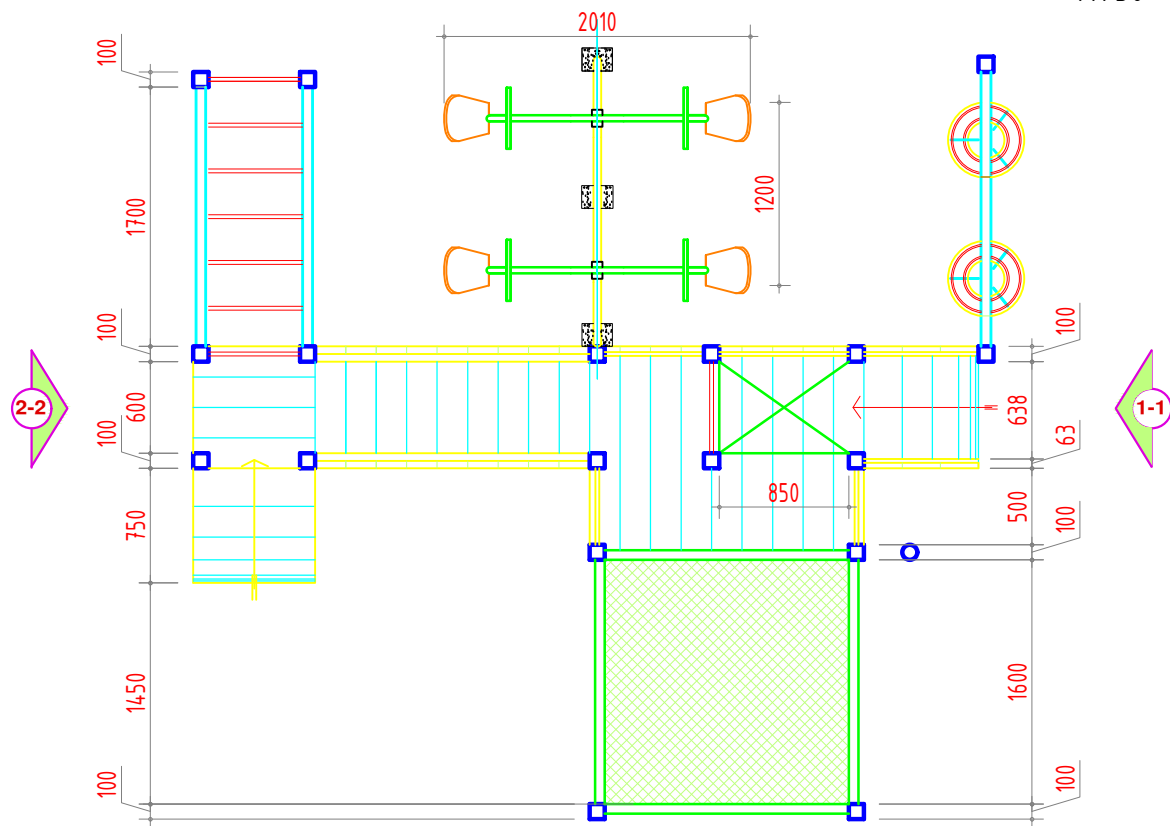
ТОГЛООМЫН БАЙГУУЛАЛТ M1:50
