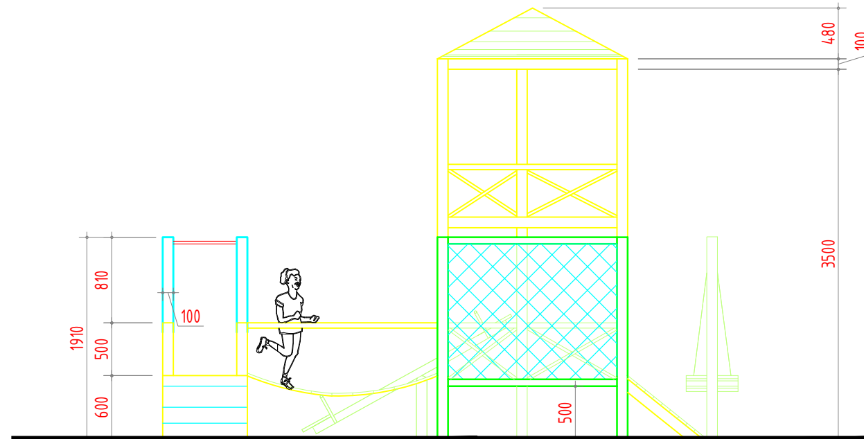
ХАЖУУ ТАЛ /3-3/ M1:50
