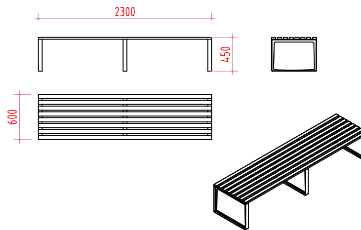
САНДАЛНЫ БАЙГУУЛАЛТ М1:50
