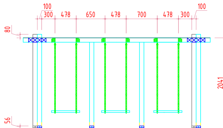
НҮҮР ТАЛ М1:50
