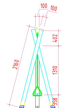
ХАЖУУ ТАЛ М1:50
