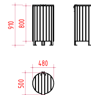
ХОГНЫ САВ БАЙГУУЛАЛТ М1:50
