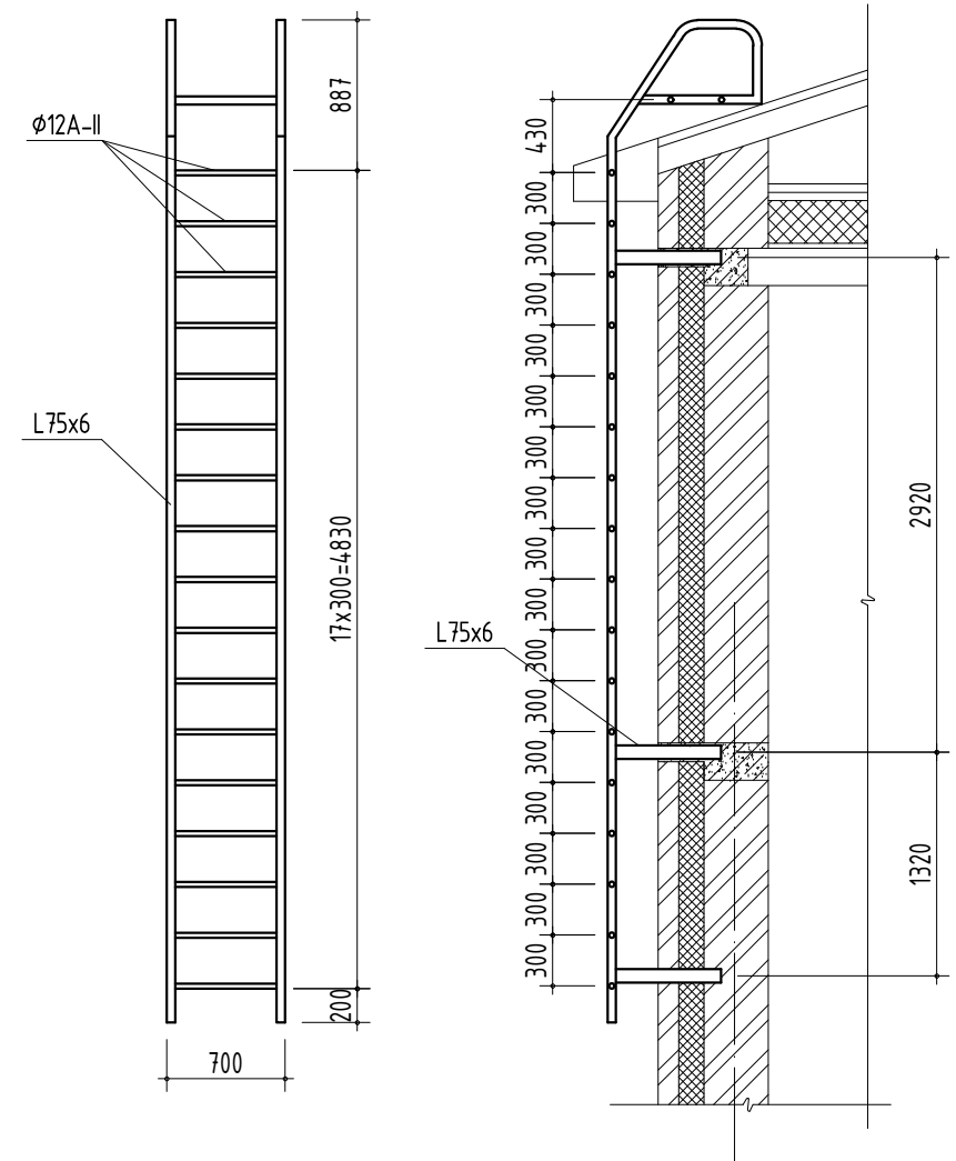
ДЭЭВЭРТ ГАРАХ ШАТНЫ БАЙГУУЛАЛТ М1:100
