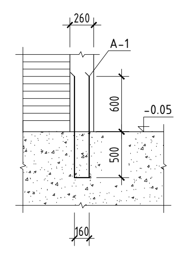
СУУРИНД АНКЕР А-1 СУУЛГАХ
