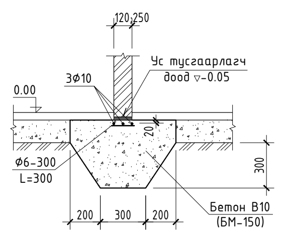
ХАМАР ХАНЫН ДООРХИ СУУРЬ
