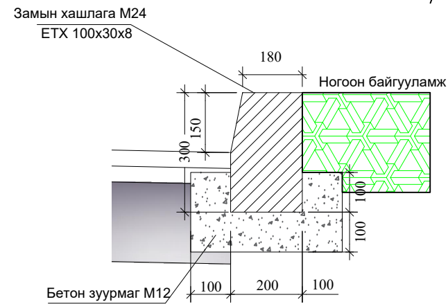
Бүтээц-1 Авто замын хашлага
