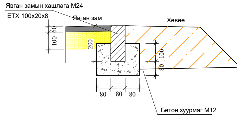
Бүтээц-2 Явган замын хашлага
