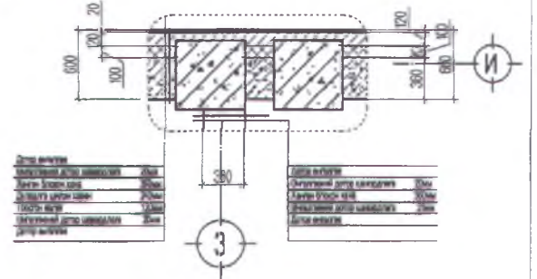
Хэсгэл-2 М1:30
