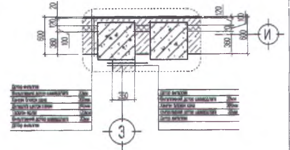
Хэсэглэл-2 М1:30
