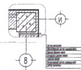
Хэсгэл-1 М1:30
