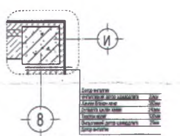
Хэсгэл-1 М1:30
