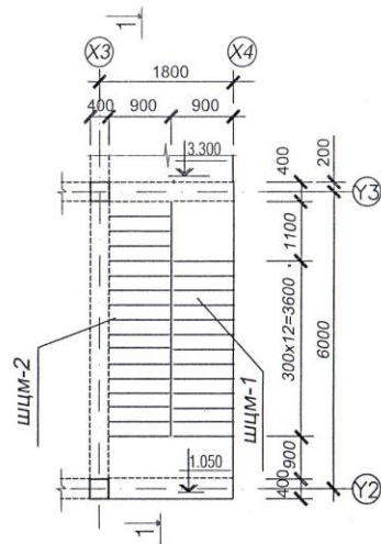
ГАДНА ШАТНЫ БАЙГУУЛАЛТ 1-1
