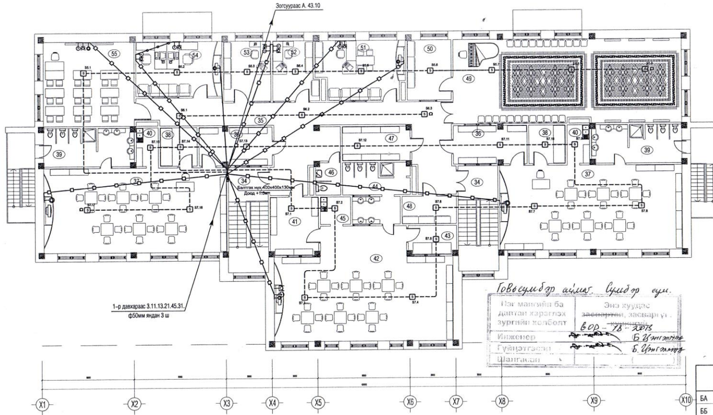
2-Р ДАВХРЫН ӨРӨӨНИЙ ТОДОРХОЙЛОЛТ
