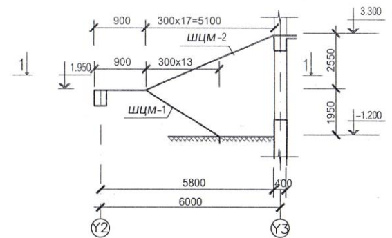
ОГТЛОЛ 1-1
