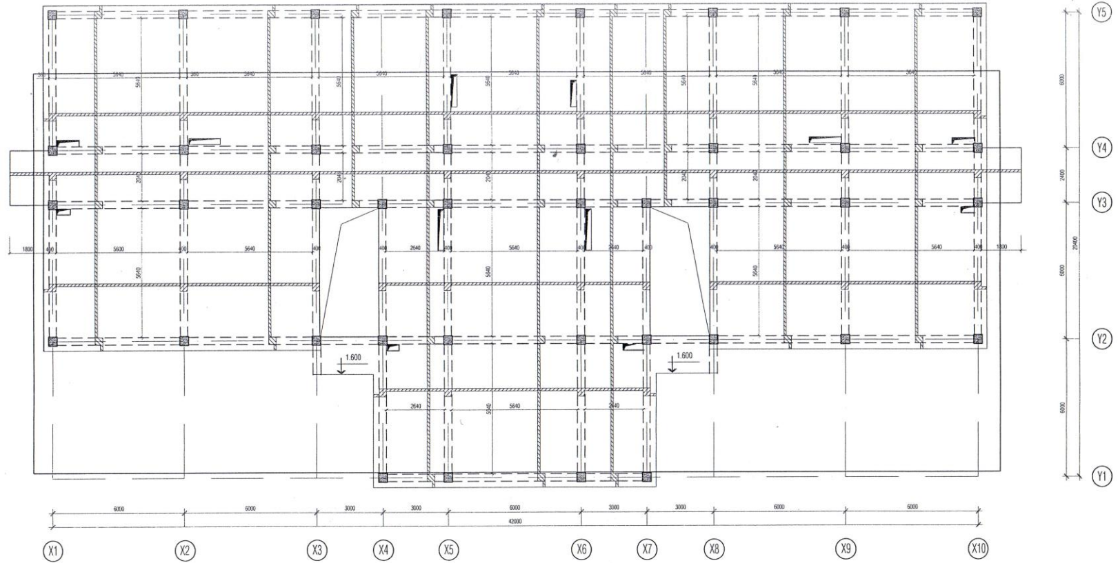
Салхиачийн нүхний нэмэлт арматурын байрлал
