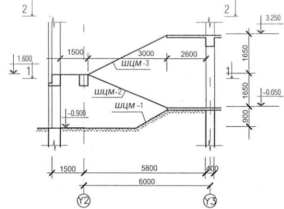
ОГТЛОЛ 1-1
