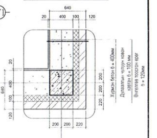
ГАДНА ХАНЫН ХЭСЭГЛЭЛ.
