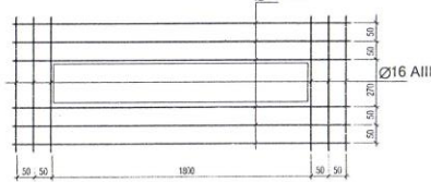
Салхиачийн нүхний нэмэлт арматурын байрлал
