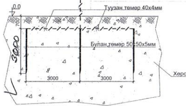
Хэсэглэл - 1 М1:100
