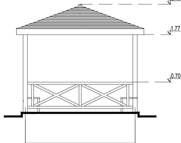
ХАЖУУ ТАЛ М1:50
