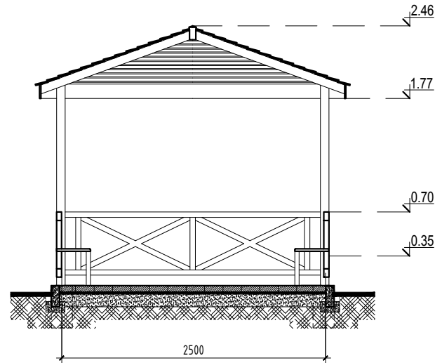
ОГТЛОЛ 1-1 М1:50
