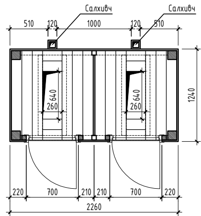
БАЙГУУЛАЛТ М1:50
