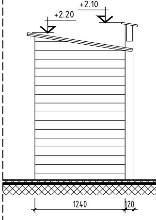
ЗҮҮН ТАЛ М1:50
