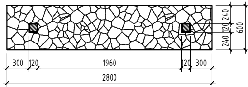
САРАВЧНЫ БАЙГУУЛАЛТ М1:50
