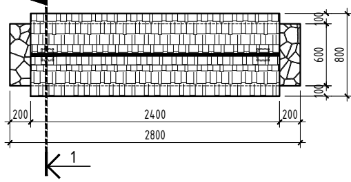
САРАВЧНЫ БАЙГУУЛАЛТ М1:50
