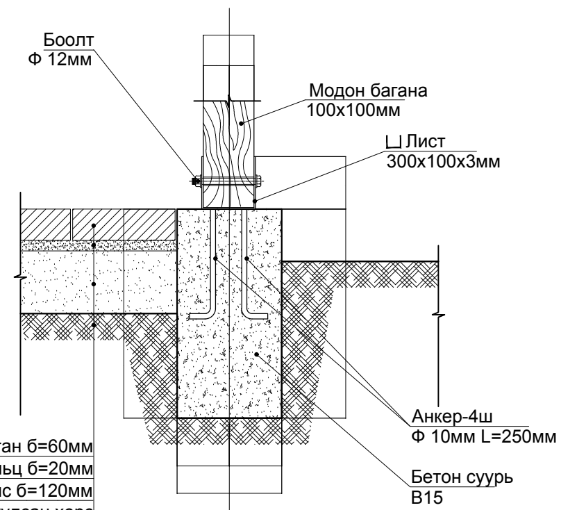
ХЭСЭГЛЭЛ-2 М1:20
