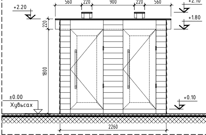
ЗҮҮН ТАЛ М1:50
