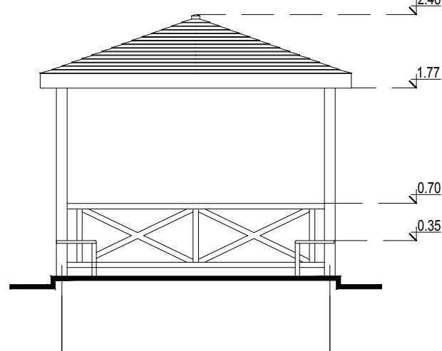
НҮҮР ТАЛ М1:50
