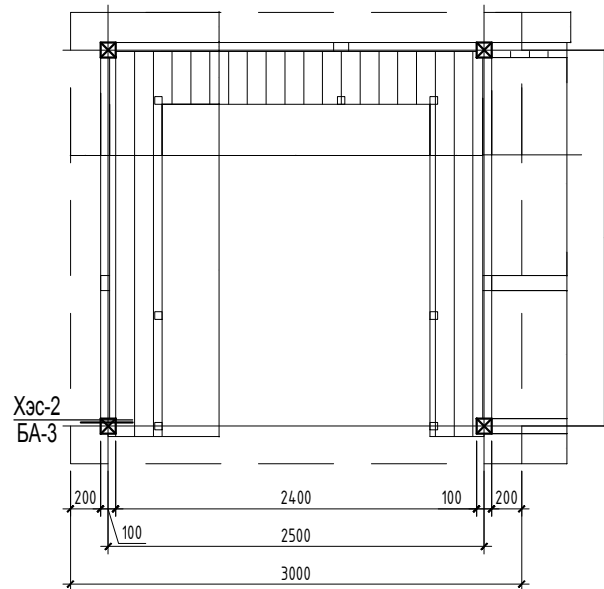
ДЭЭВРИЙН БАЙГУУЛАЛТ ТАЛ М1:50
