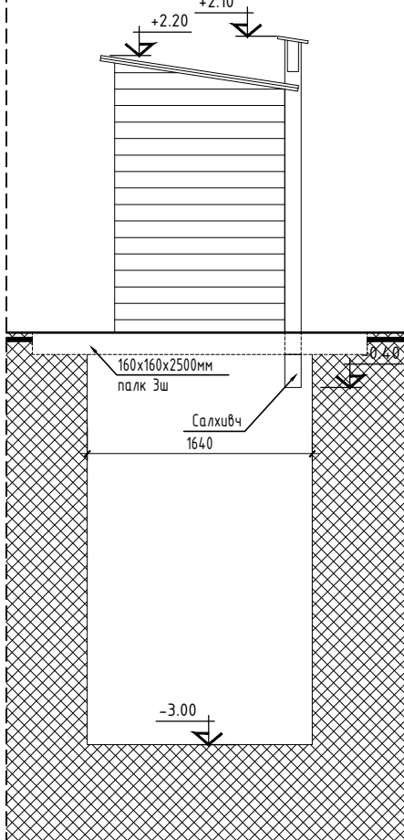
ОГТЛОЛ М1:50
