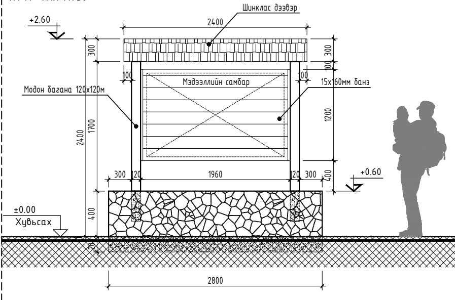
НҮҮР ТАЛ М1:50
