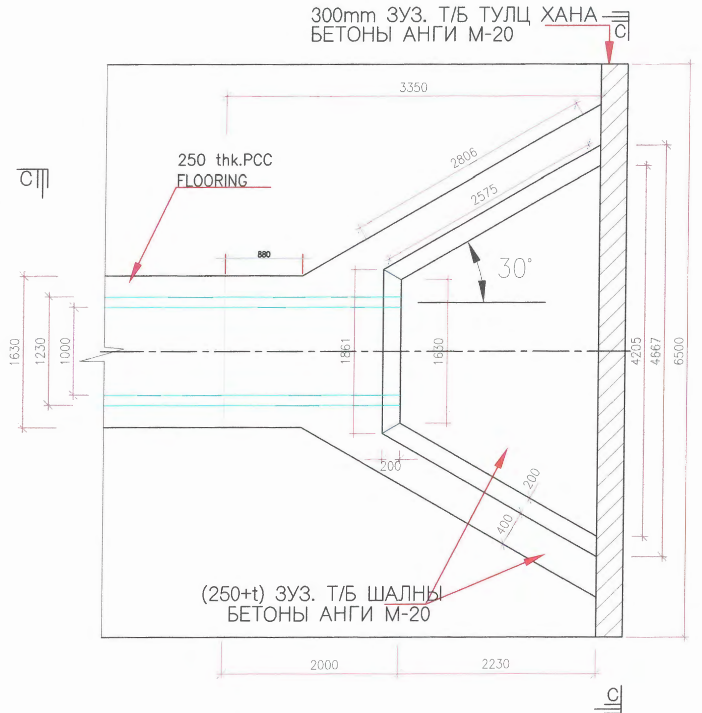
Т/Б ШАЛ, ТУЛЦ ХАНА, СУУРИЙН ДЭВСГЭР ЗУРАГ
