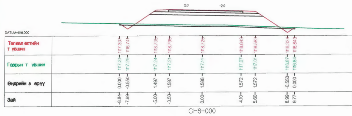
CH6+000
