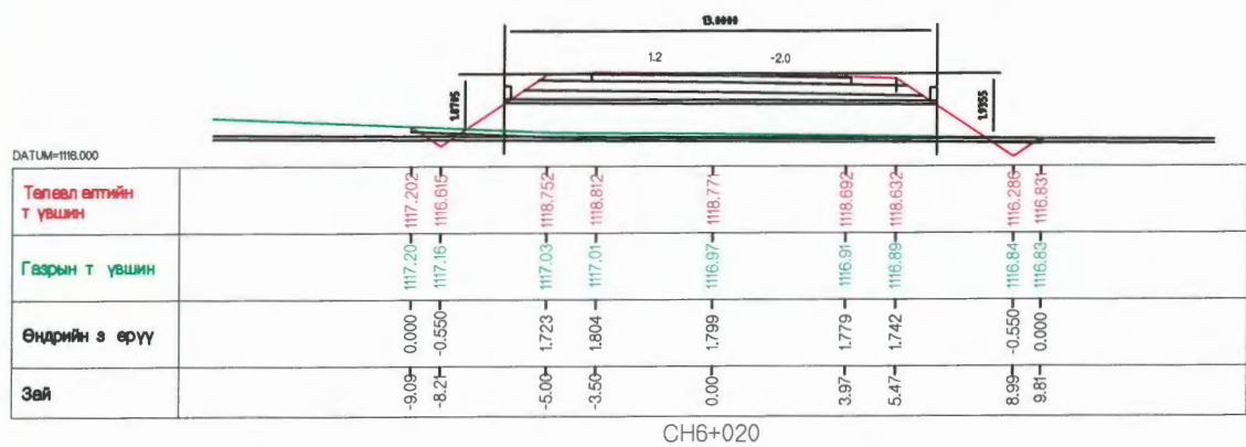
CH6+020
