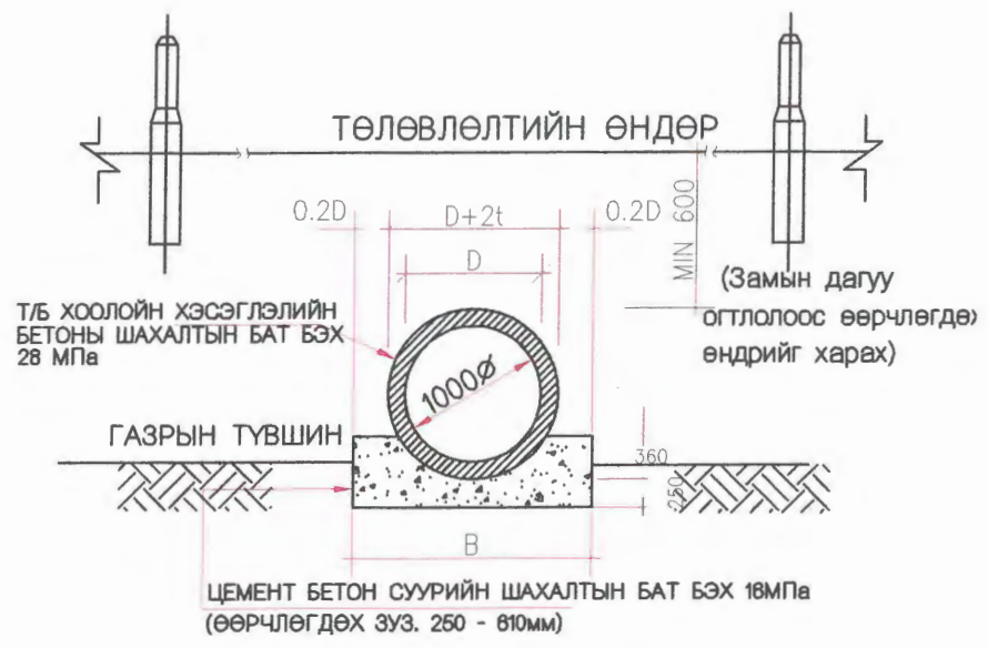
Огтлол В-В
