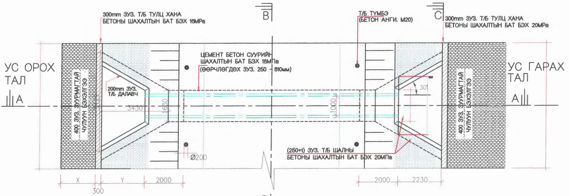
ПЛАН
