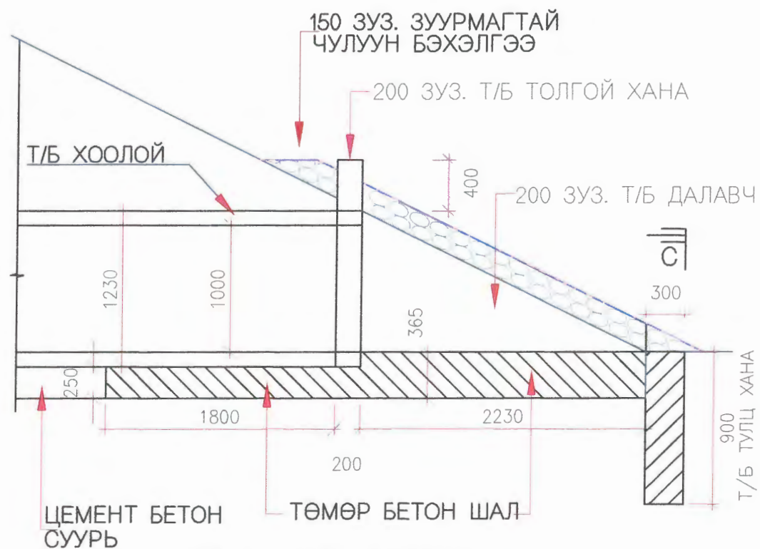
ХИЙЦҮҮДИЙН ХЭМЖЭЭ Т/Б ТОЛГОЙ, ДАЛАВЧ, ШАЛ, ТУЛЦ ХАНА
