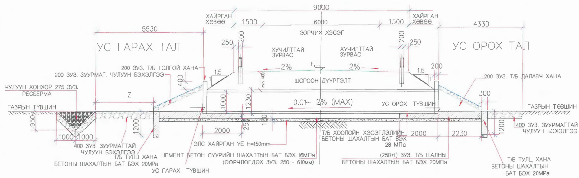
ОГТЛОЛ А-А
