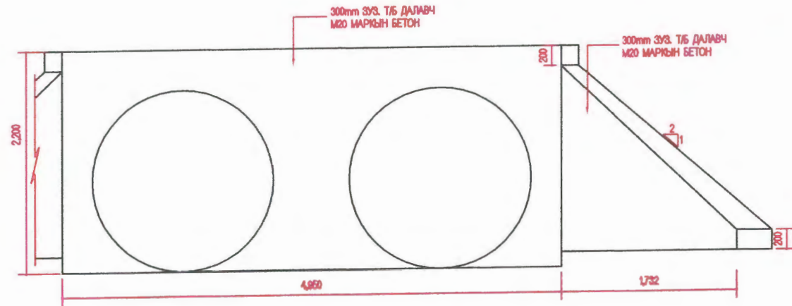
ХИЙЦҮҮДИЙН ХЭМЖЭЭ Т/Б ТОЛГОЙ, ДАЛАВЧ, ШАЛ, ТУЛЦ ХАНА
