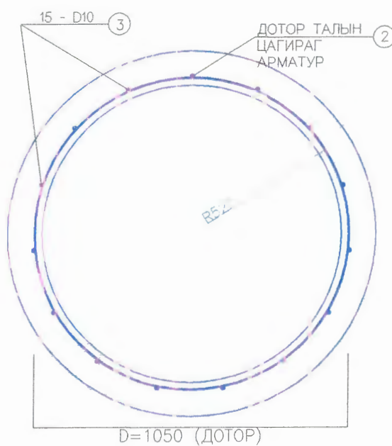
ДАВХАР АРМАТУРЫН ТОР
