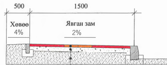
Явган зам SCALE 1:50
