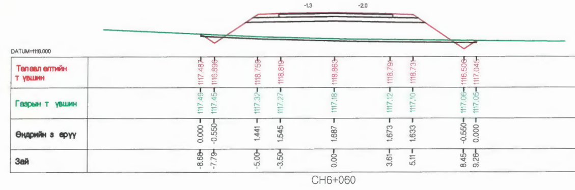
CH6+060
