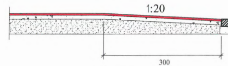
Б-Б огтлол
