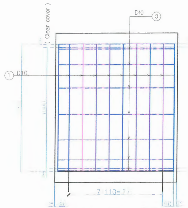
ДОТОР ТАЛЫН ТОР
