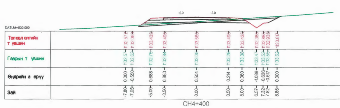
CH4+400
