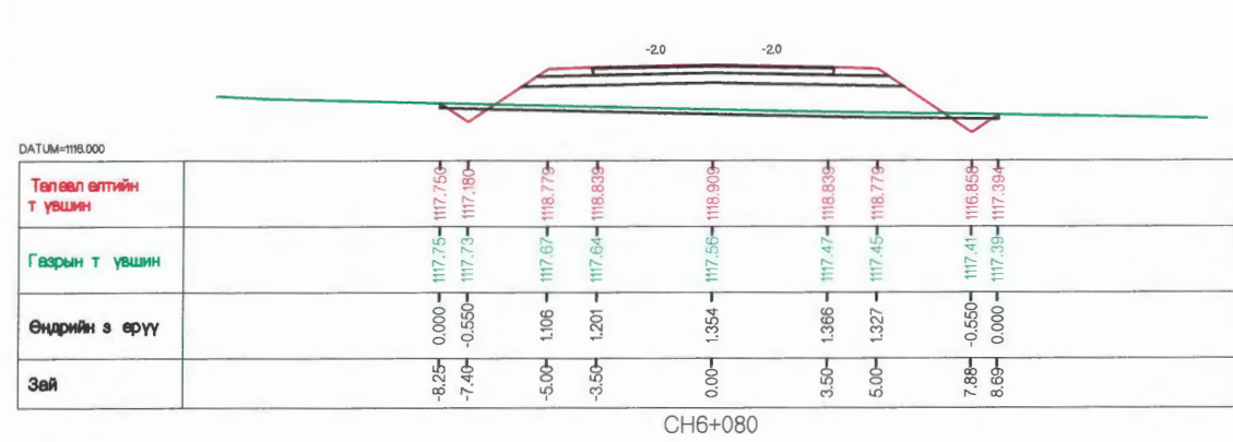
CH6+080
