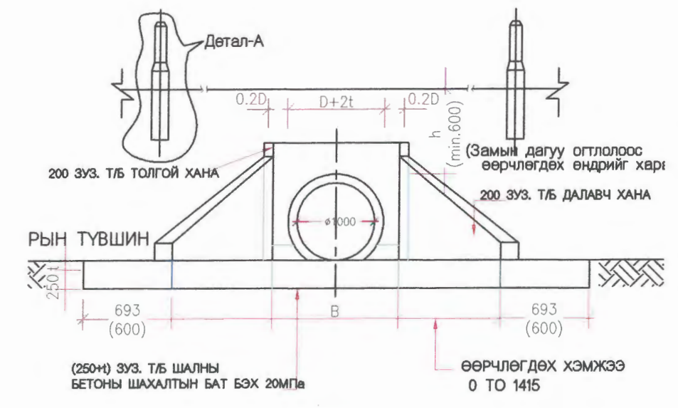
Огтлол С-С
