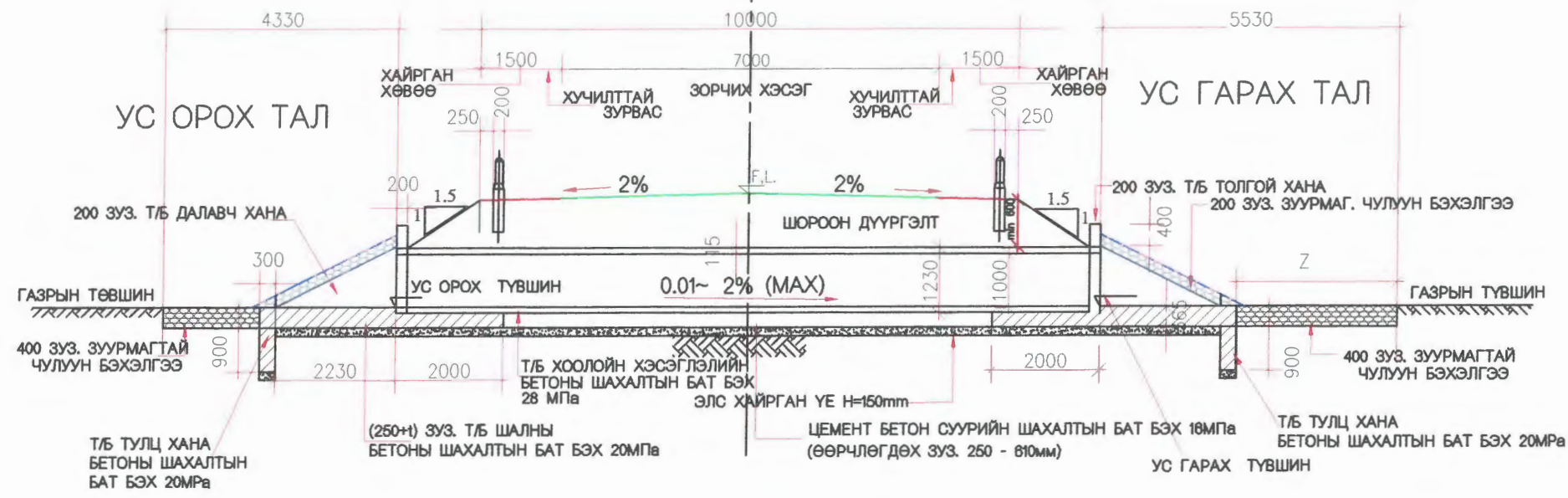
ОГТЛОЛ А-А
