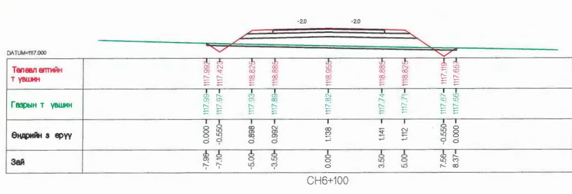
CH6+100
