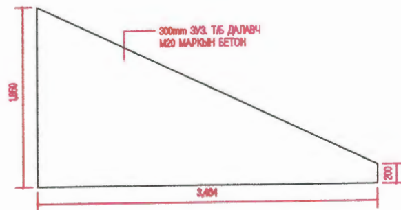
ОГТЛОЛ 1-1
