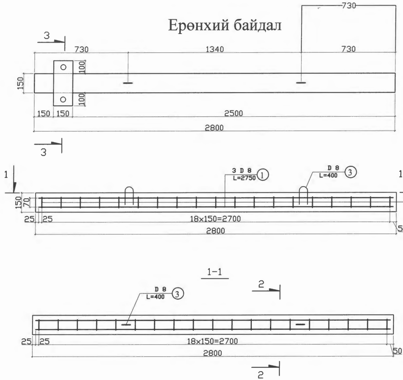
Км-ийн шонгийн арматурын хуваарь
