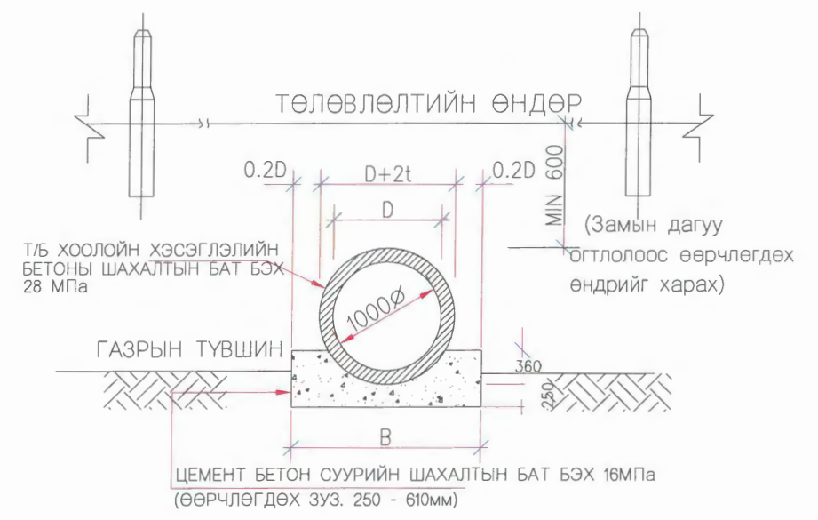
Огтлол В-В
