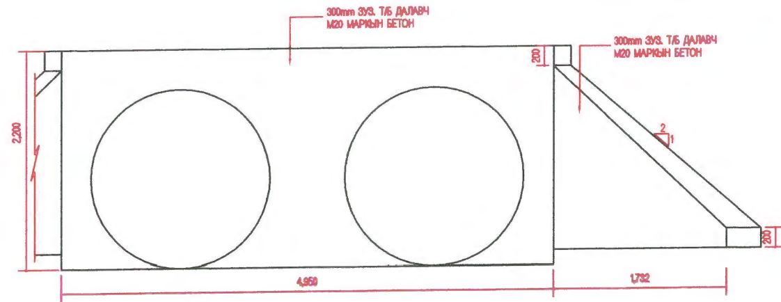
ХИЙЦҮҮДИЙН ХЭМЖЭЭ Т/Б ТОЛГОЙ,ДАЛАВЧ, ШАЛ, ТУЛЦ ХАНА
