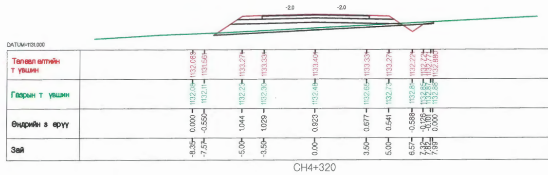
CH4+320
