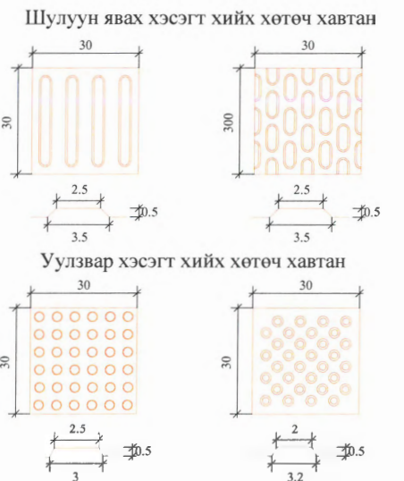
Хараагүй хүний хөтөч зам SCALE 1:20
