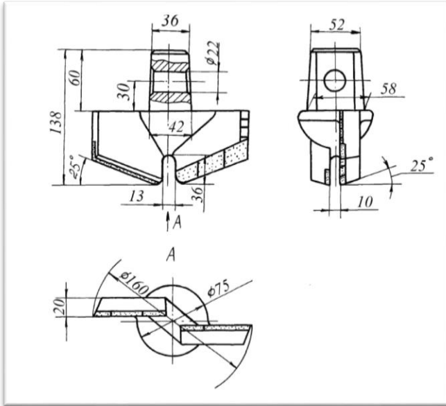
Зураг №1 өрмийн хошууны хэмжээсүүдийг мм-р үзүүлэв.
