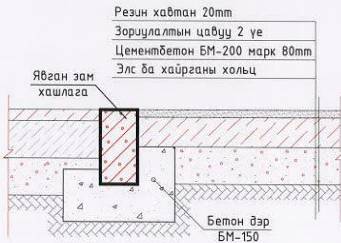
ХҮҮХДИЙН ТОГЛООМЫН ТАЛБАЙН РЕЗИН ХУЧИЛТ ОГТЛОЛ-4
