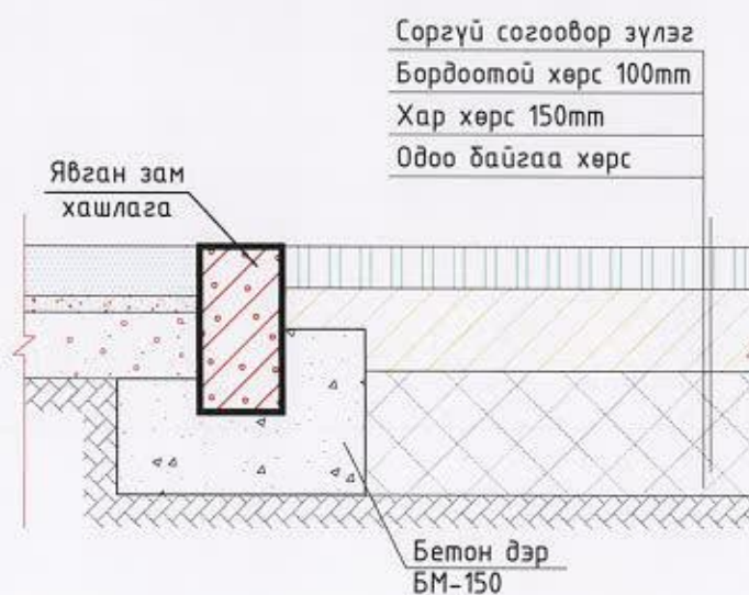
ЗҮЛЭГЖҮҮЛЭХ ТАЛБАЙН ОГТЛОЛ-5
