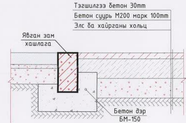
БЕТОН ХУЧИЛТТАЙ ЧИЙРЭГЖҮҮЛЭХ ТАЛБАЙН ОГТЛОЛ-3
