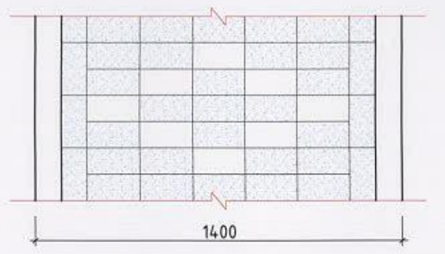
ШАХМАЛ ХАВТАН ХУЧИЛТТАЙ ЗАМ ОГТЛОЛ-2
