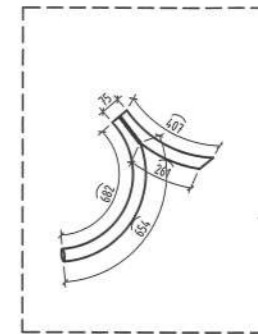
ХЭСЭГЛЭЛ 1 М150
