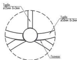
Хэсэглэл 2 М1:10
