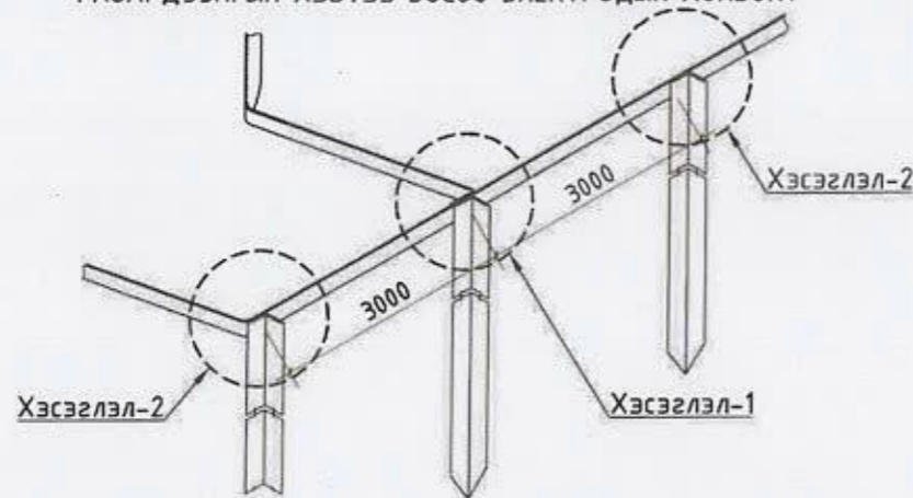
ГАЗАРДУУЛГЫН ХЭВТЭЭ БОСОО ЭЛЕКТРОДЫН ХОЛБОЛТ
