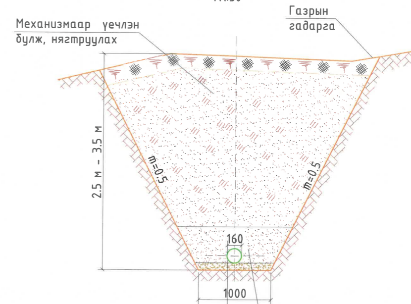
Нэг маягийн хөндлөн огтлол М1:50
