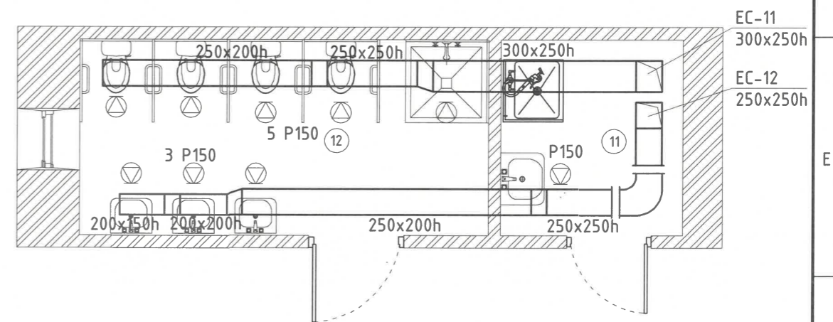
ХЭСЭГЧИЛСЭН БАЙГУУЛАЛТ "Д"
