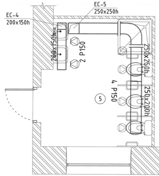
ХЭСЭГЧИЛСЭН БАЙГУУЛАЛТ "В"
