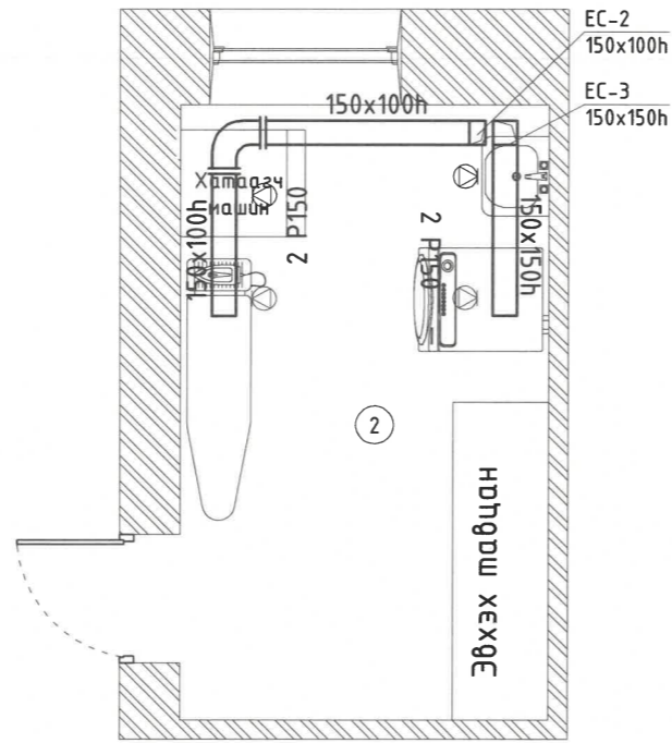
ХЭСЭГЧИЛСЭН БАЙГУУЛАЛТ "Б"
