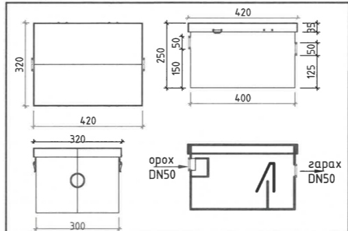
Тос баригчийн зураг
