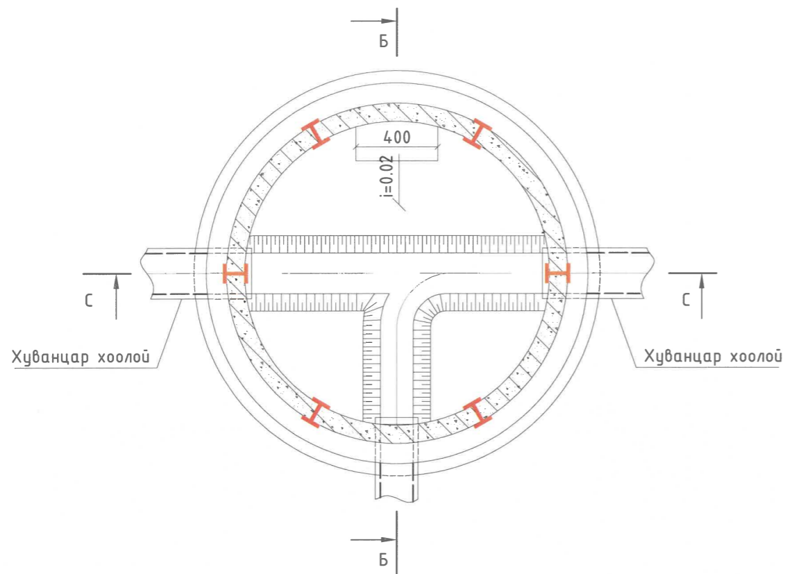
Схем I Хүдгийн байгуулалт Огтлол А-А М1:25
