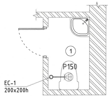
ХЭСЭГЧИЛСЭН БАЙГУУЛАЛТ "А"
