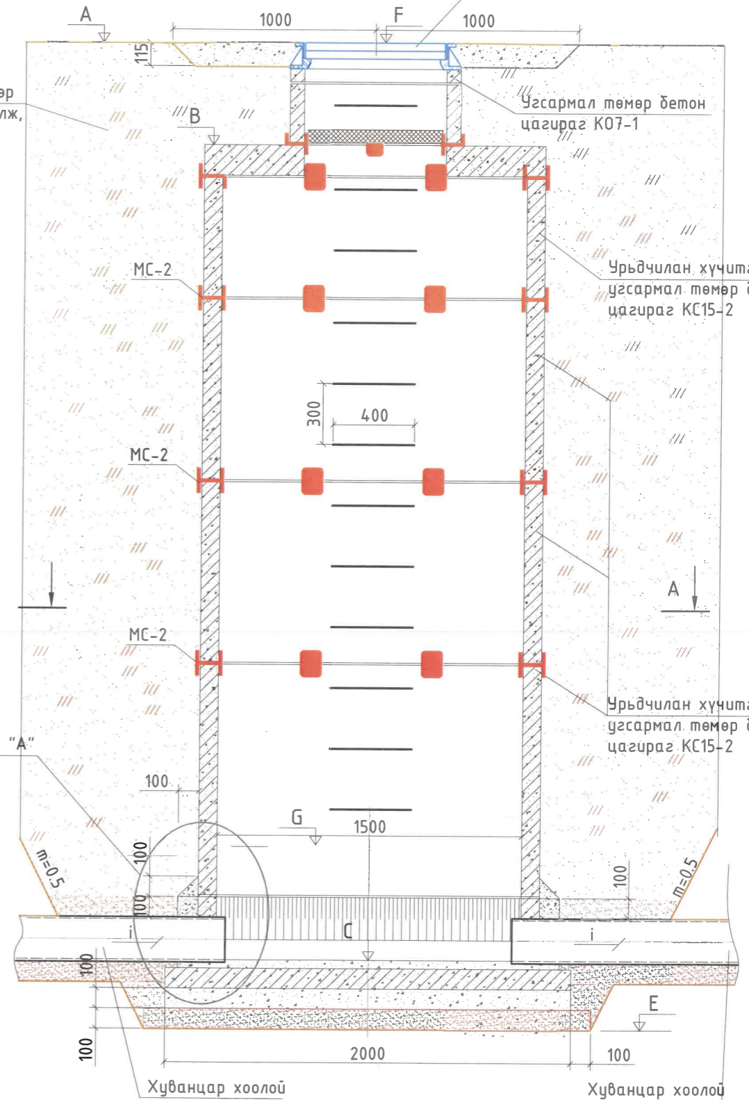
Огтлол С-С M1:25
