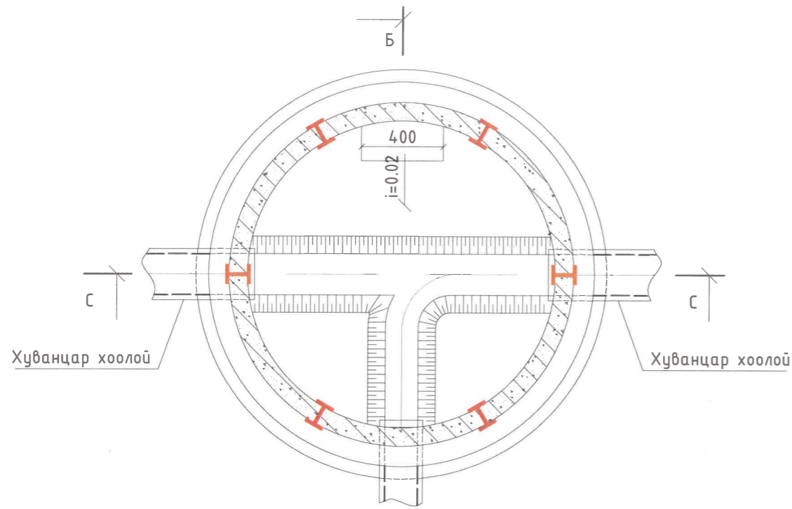
Схем I Худгийн байгуулалт Огтлол А-А M1:25
