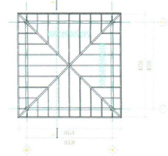
Дээврийн бүтээц М:75
