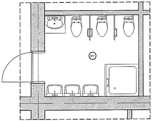
АХЛАХ БҮЛГИЙН "А" ӨРӨӨНИЙ ШАЛНЫ БАЙГУУЛАЛТ М1:50
