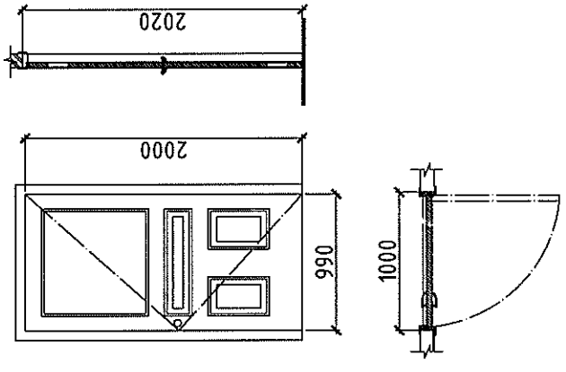
Модон хаалга M1:50
