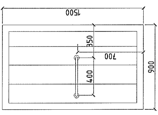
Шүршүүрийн хуванцар хаалт Хавтан /3ш/
