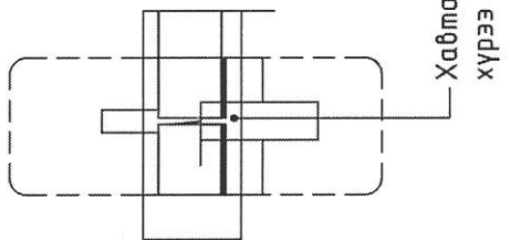
ХЭС-2 /M1:5/
