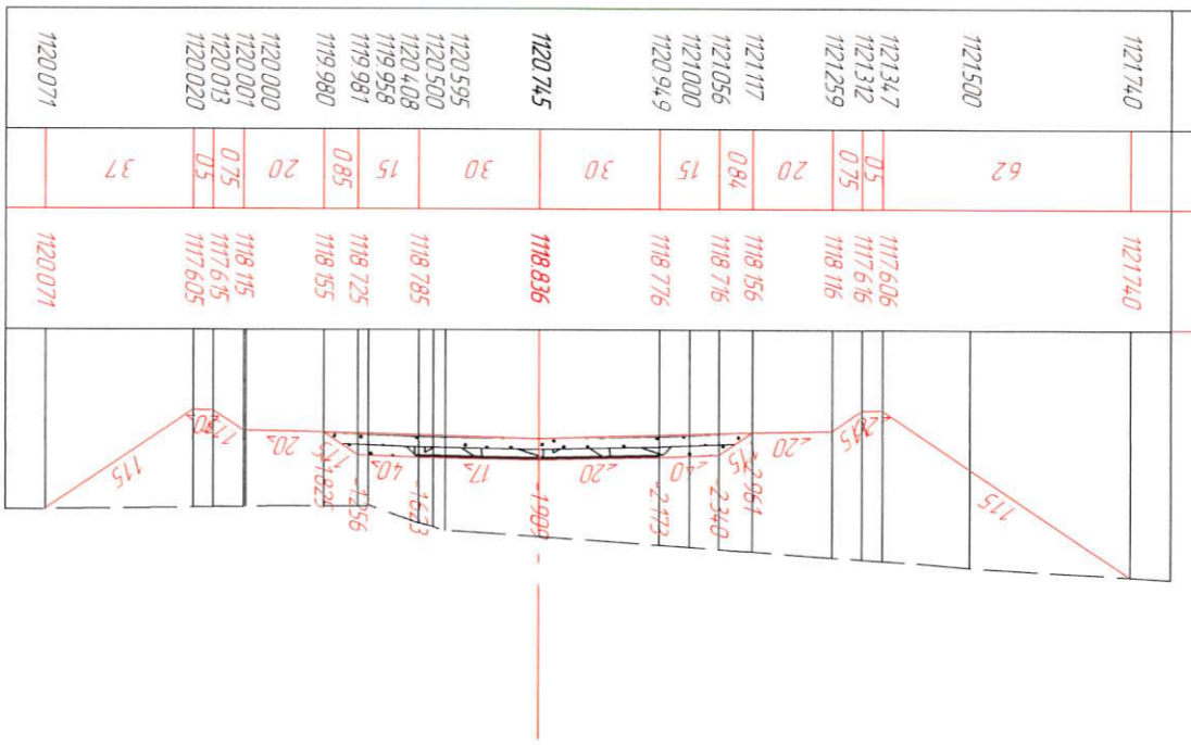
НК 5+140.00
