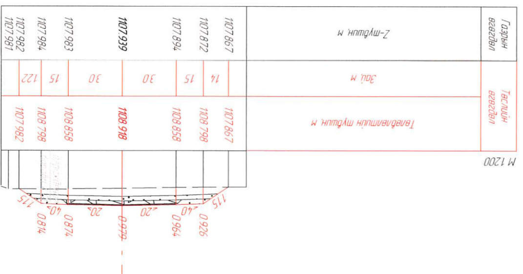
ПК 2+380.00
