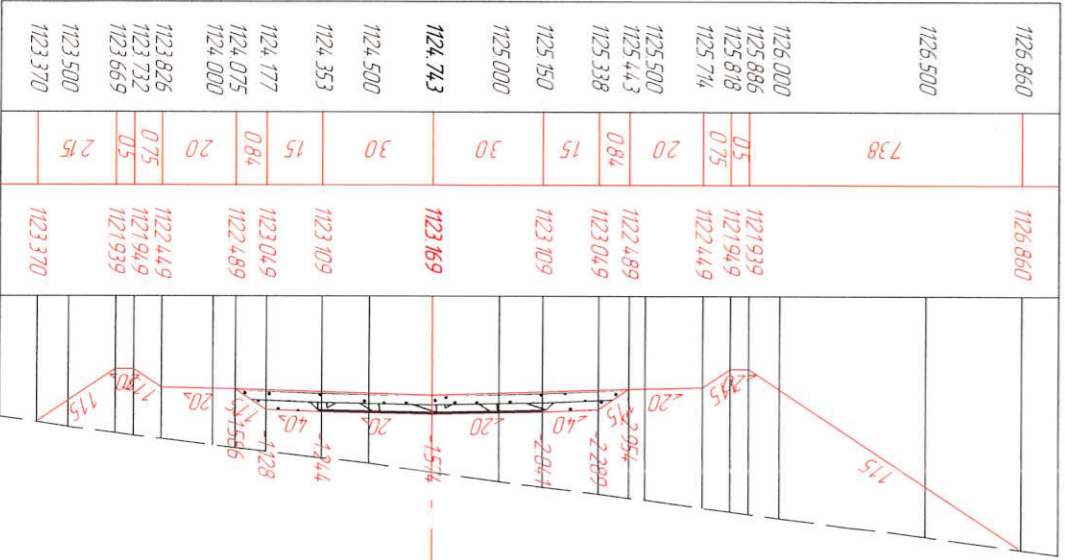
ЛК 6+380.00
