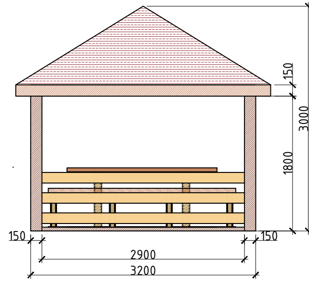
ХАЖУУ ТАЛ М1:50
