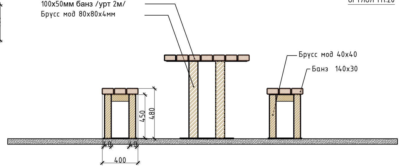
ОГТЛОЛ М1:20
