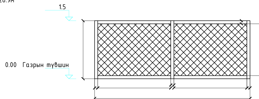
НҮҮР ТАЛ М1:25
