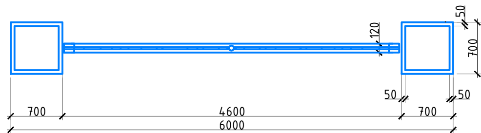
Харагдах байдал М1:50
