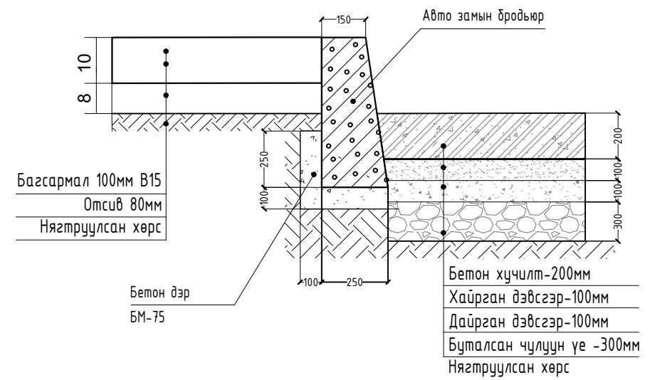
Огтлол 1-1 М1:10
