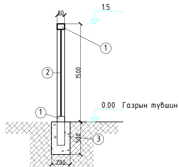
ОГТЛОЛ 1-1 М1:25
