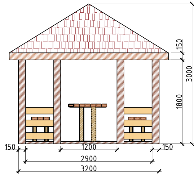
НҮҮР ТАЛ М1:50
