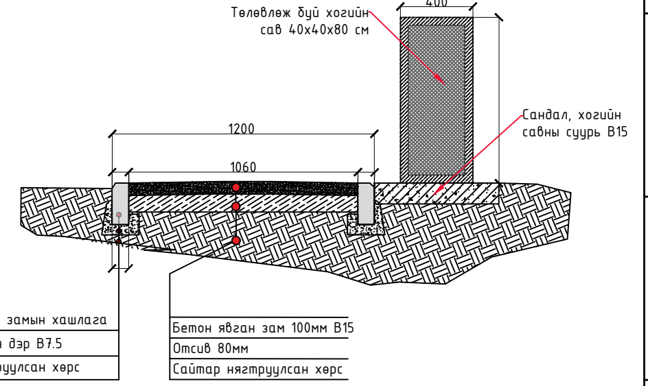
ОГТЛОЛ Б-Б M1:25
