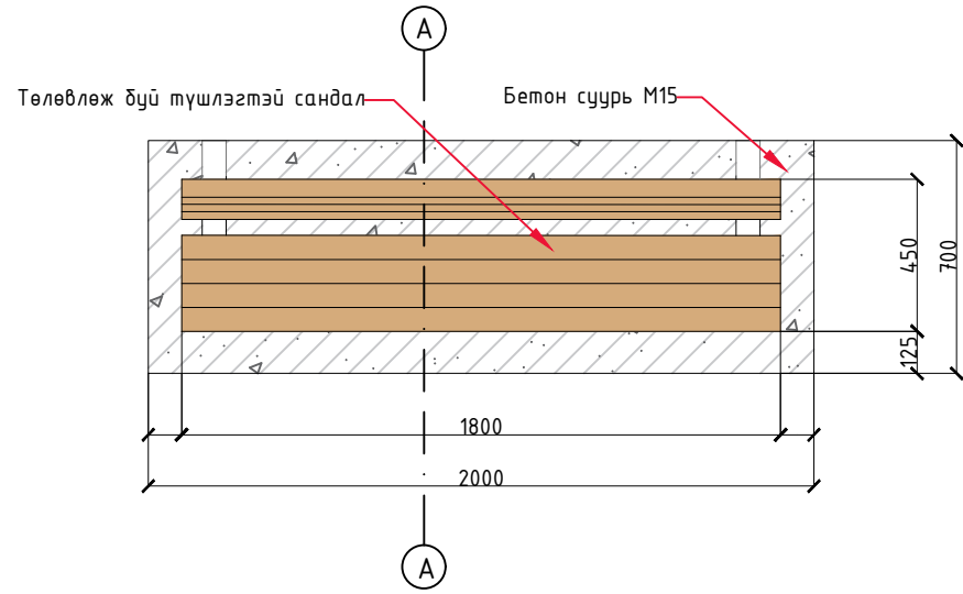
САНДАЛНЫ БАЙГУУЛАЛТ M1:25
