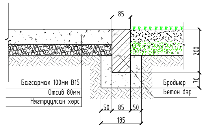
Огтлол 1-1 М1:10
