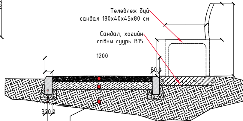
ОГТЛОЛ А-А M1:50
