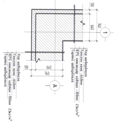
ХЭСЭГЛЭЛ-1 М1:25
