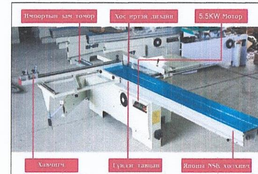
Хавтан зүсдэг хөрөө
