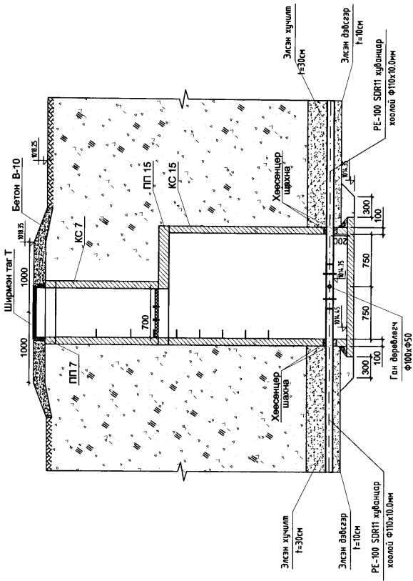
Цэвэр усны худаг ЦХ-12 М1:50 Огтлол 12-12
