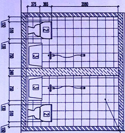
Ханын дэлгээс Б-Б
