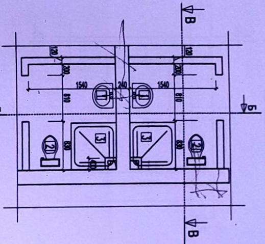
Хэсэгтэл "2"
