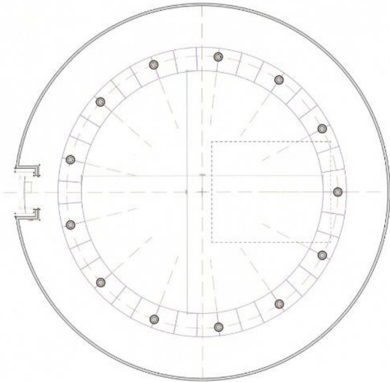
Гипсан ханын утврлганы байгуулалт /F-4 Деталь/
