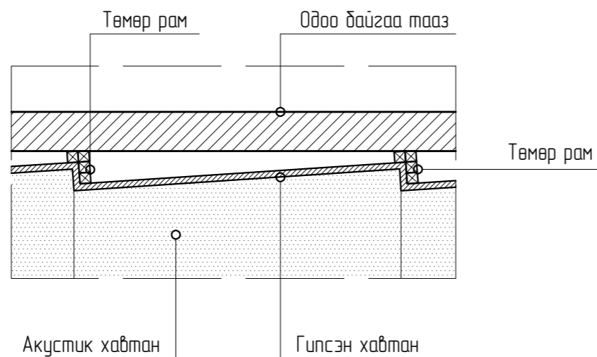
Таазны хэсэглэл М1:25
