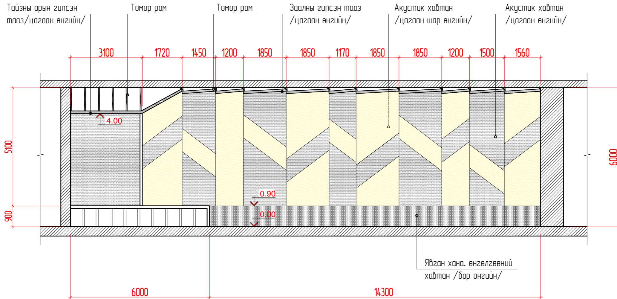
Таазны хэсэглэл M1:25
