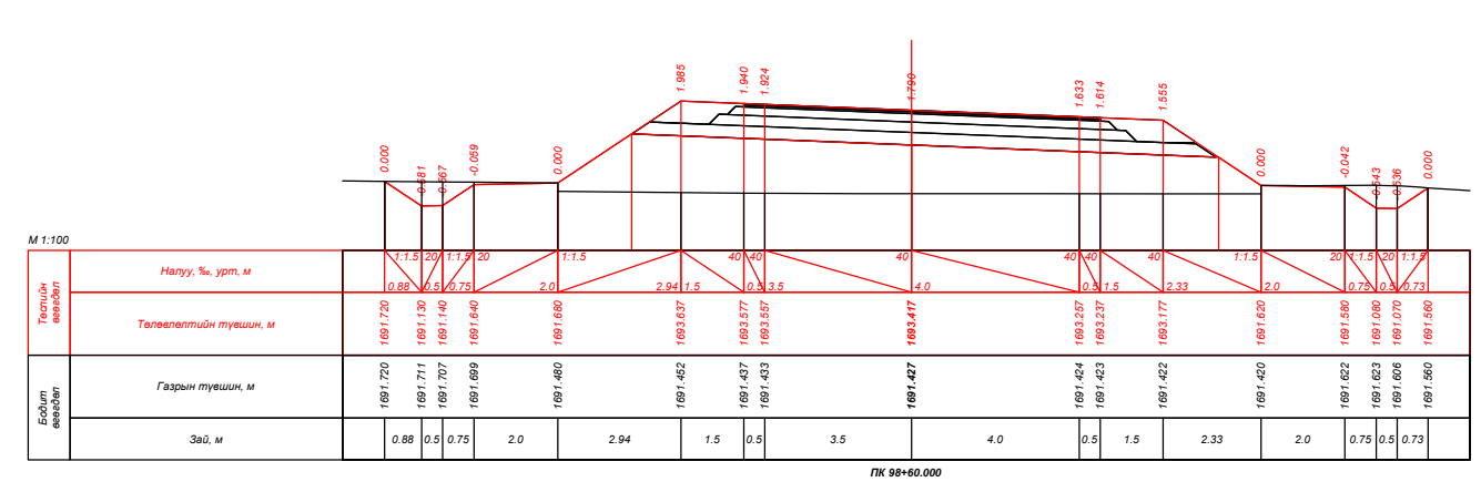
ПК 98+60.000
