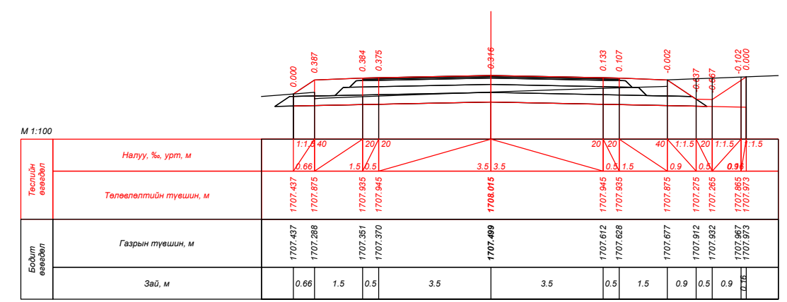
ПК 72+20.000
