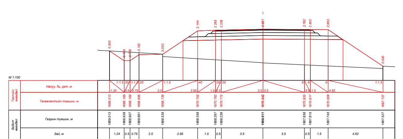
ПК 22+20.000
