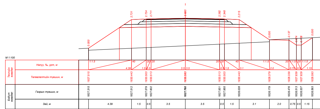
ПК 242+60.000
