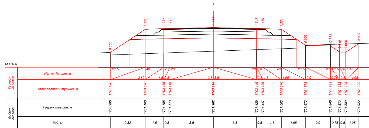
ПК 75+20.000
