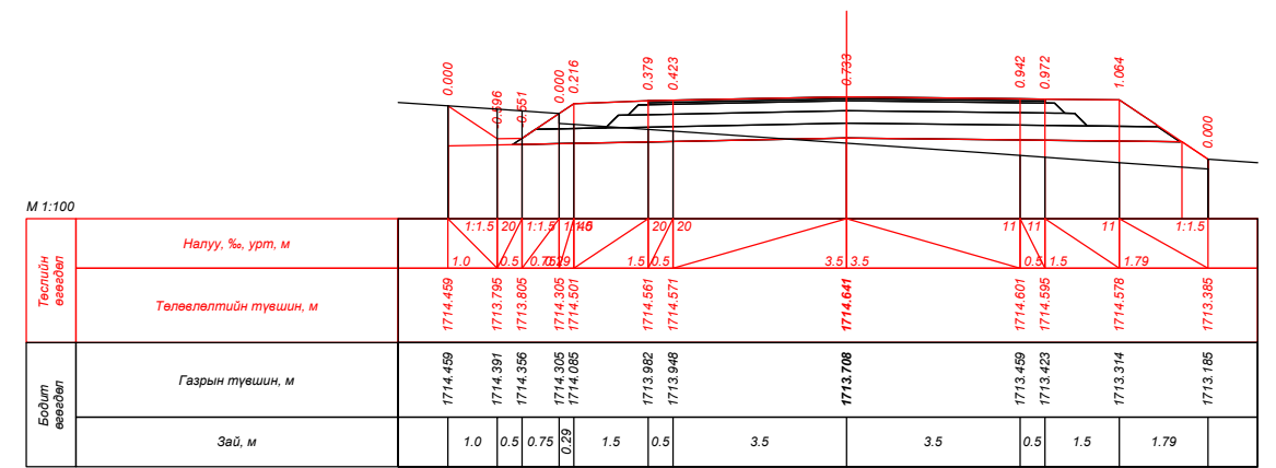
ПК 118+20.000
