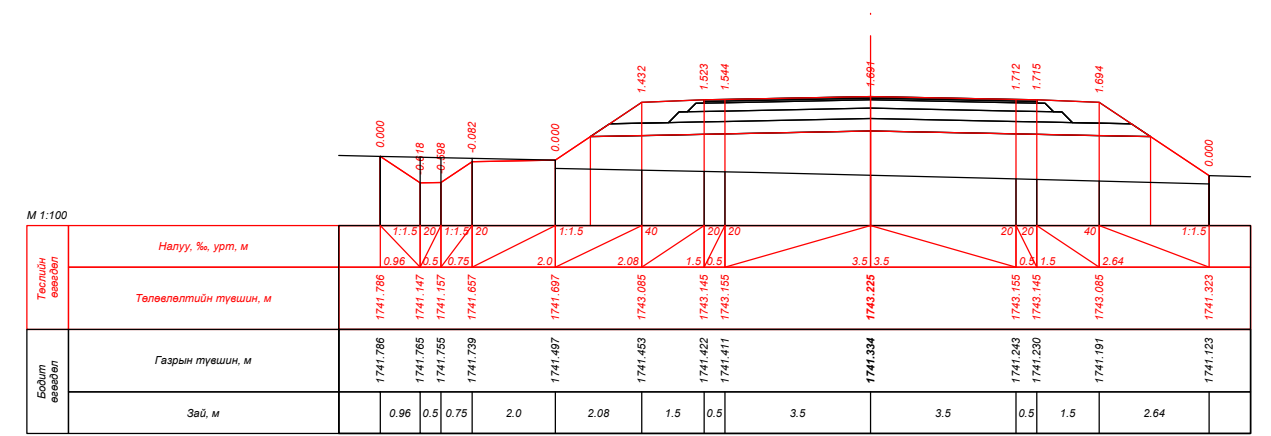
ПК 143+60.000
