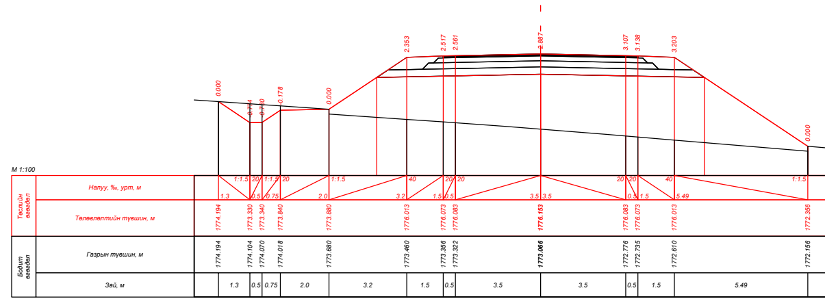
ПК 180+80.000
