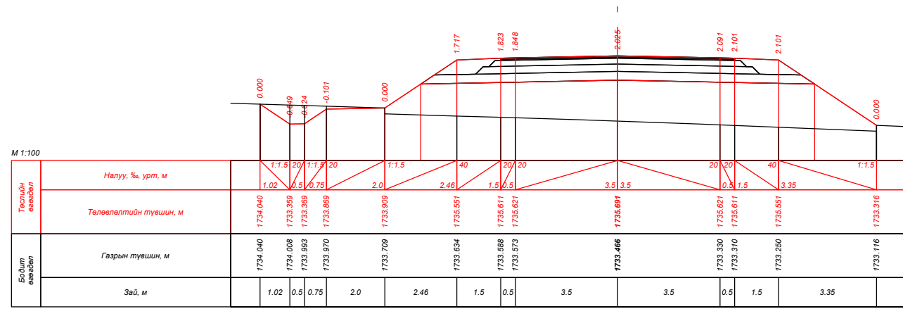
ПК 139+00.000
