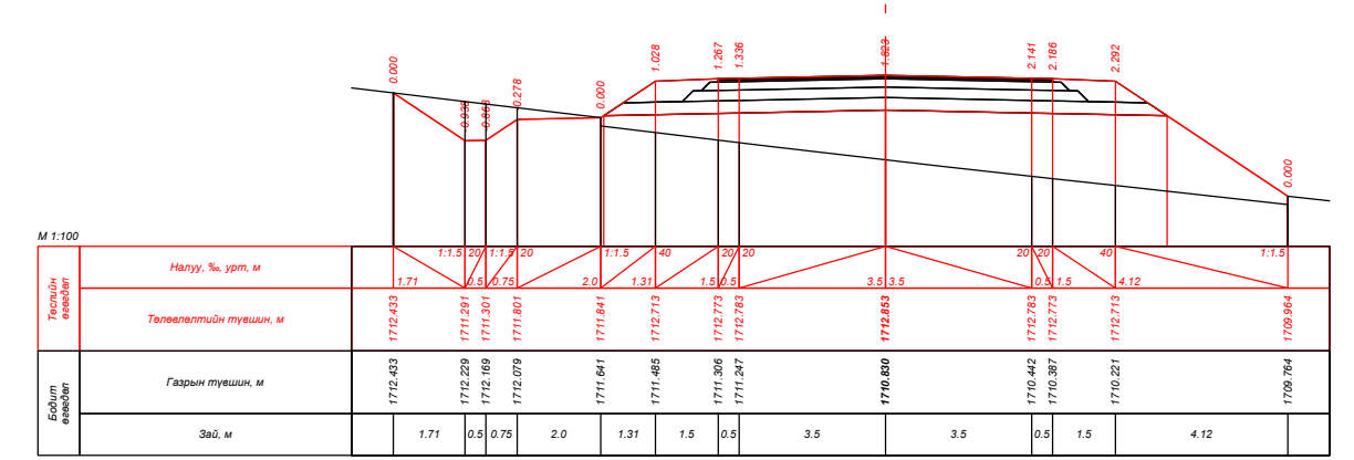
PK 110+60.000
