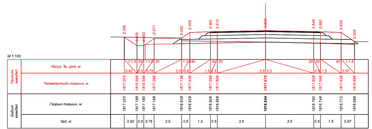
ПК 213+80.000
