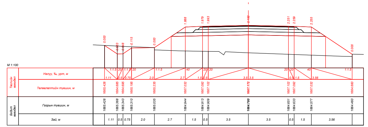
ПК 11+00.000
