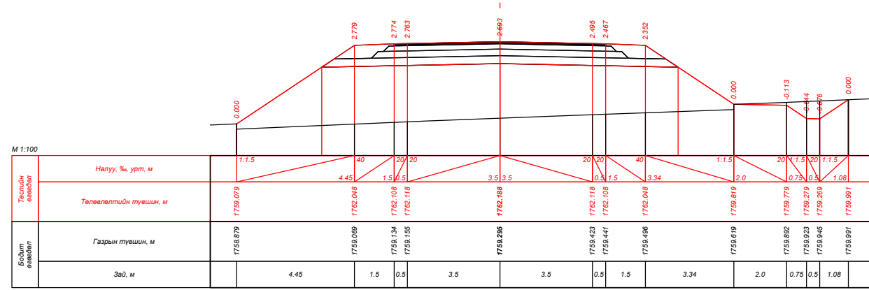
ПК 275+20.000
