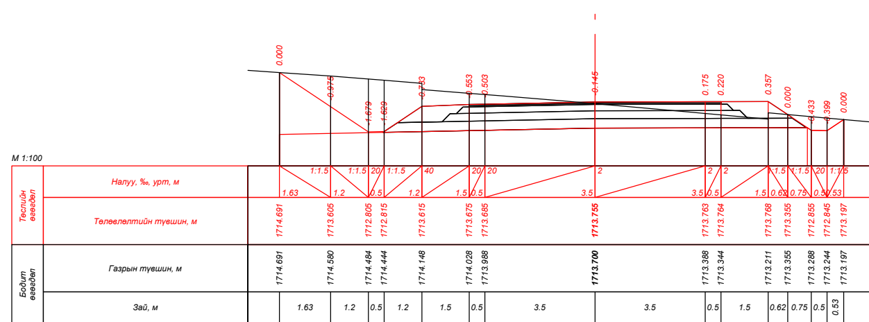
ПК 118+60.000
