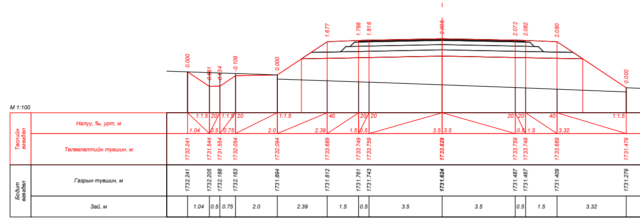
ПК 137+60.000
