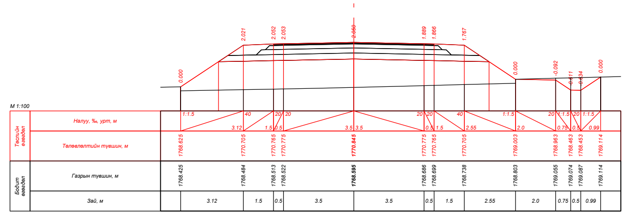
ПК 267+40.000
