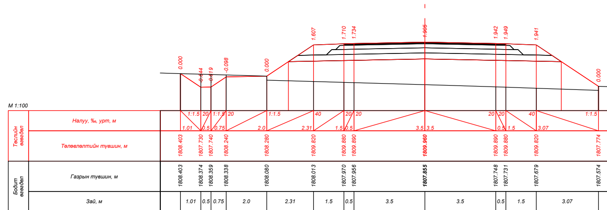
ПК 208+60.000
