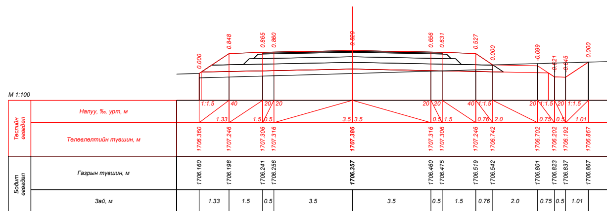
ПК 72+80.000
