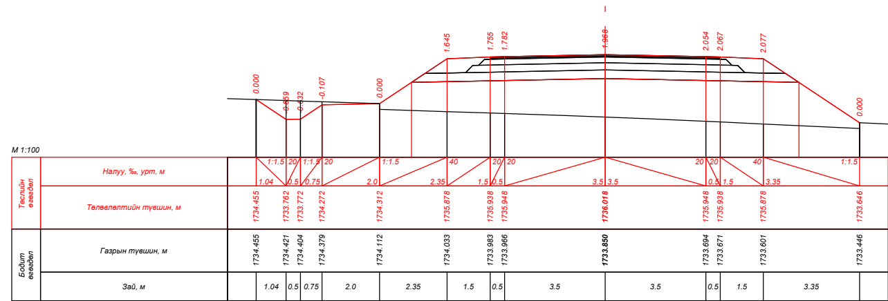
ПК 139+20.000
