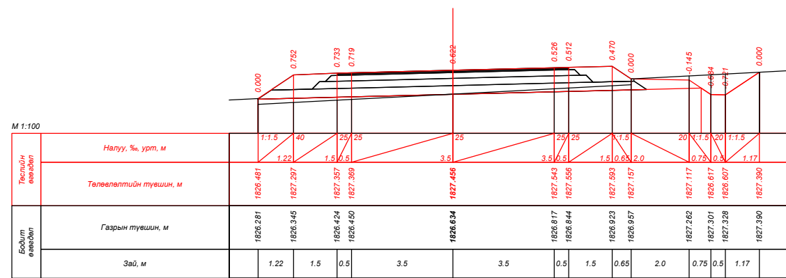
ПК 234+40.000
