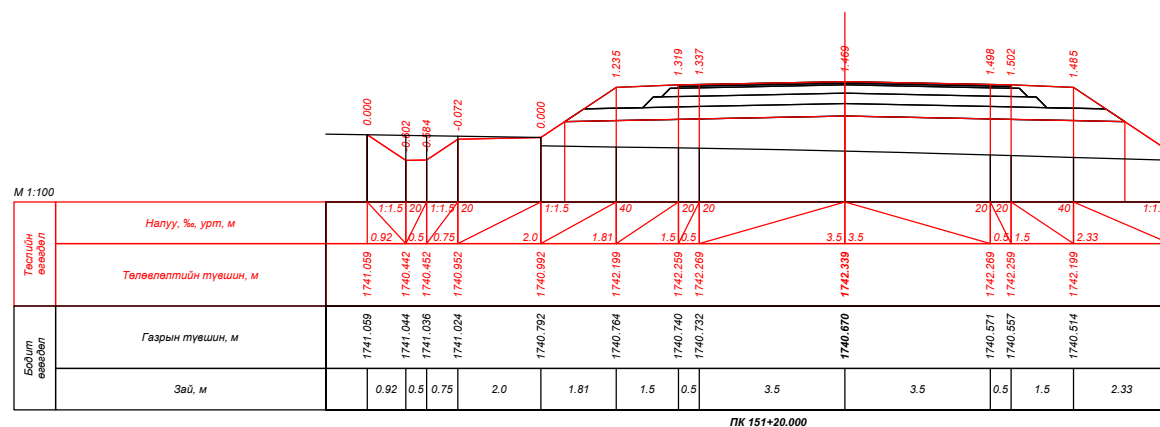
ПК 151+20.000
