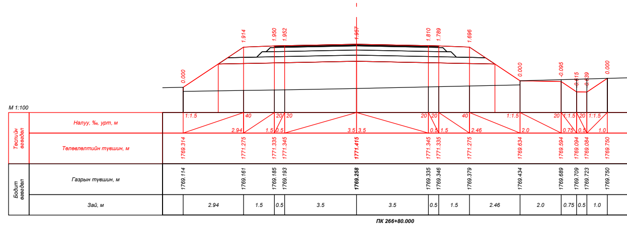
ПК 266+80.000
