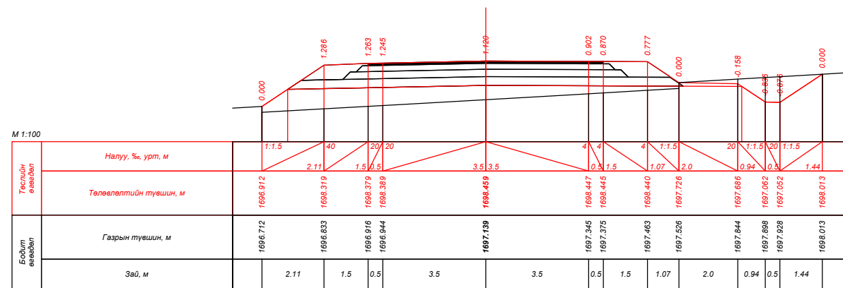
ПК 77+20.000
