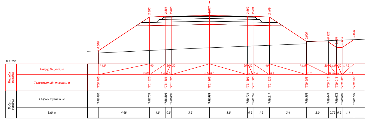
ПК 275+40.000
