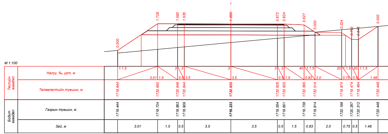
ПК 38+69.294
