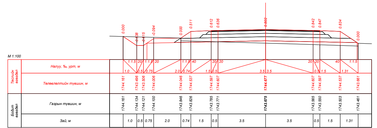
ПК 148+40.000
