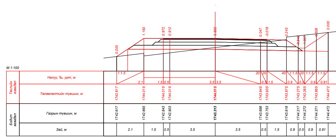
ПК 59+56.646
