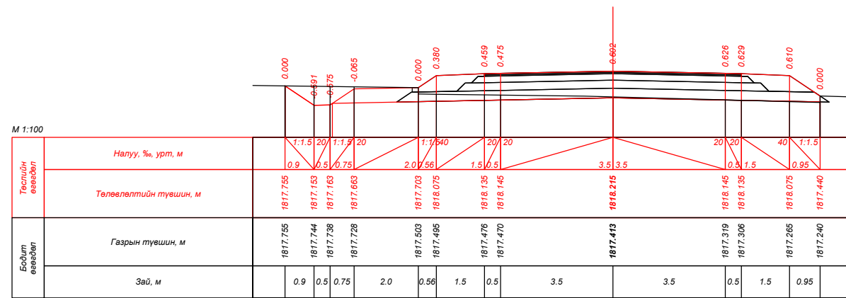
ПК 214+00.000
