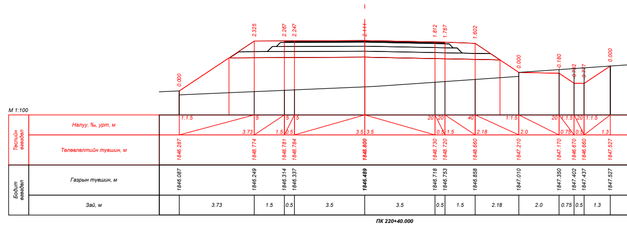
ПК 220+40.000
