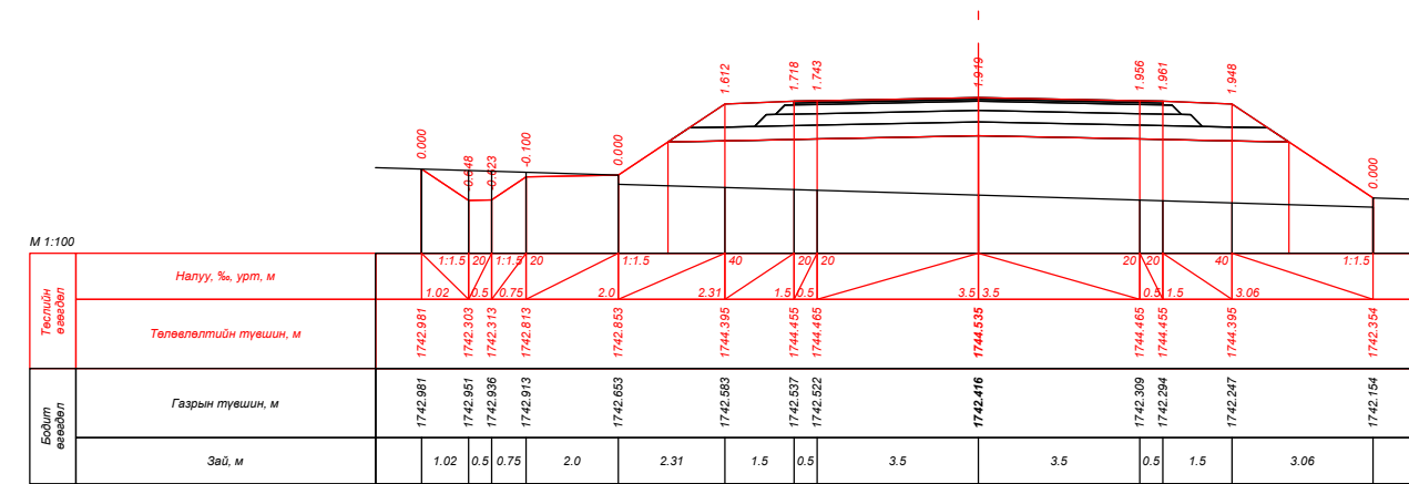
ПК 144+40.000
