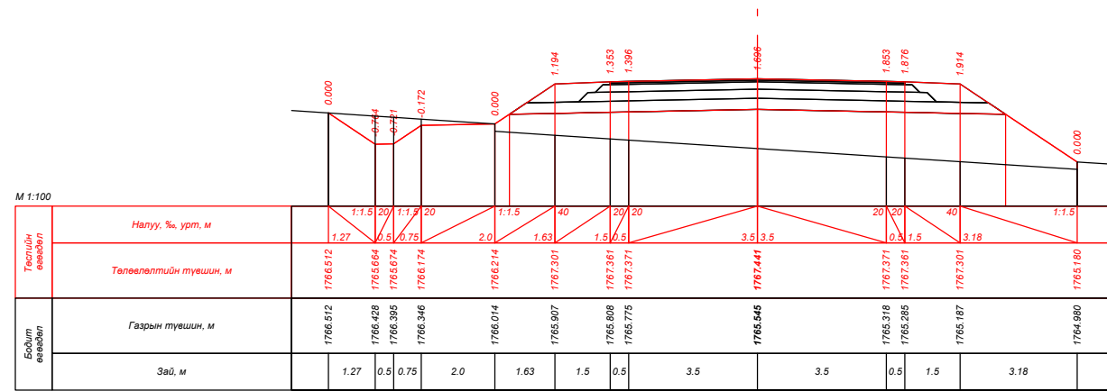
ПК 172+40.000
