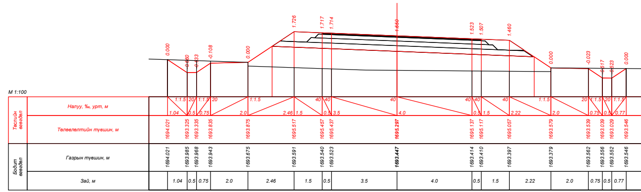
ПК 101+60.000
