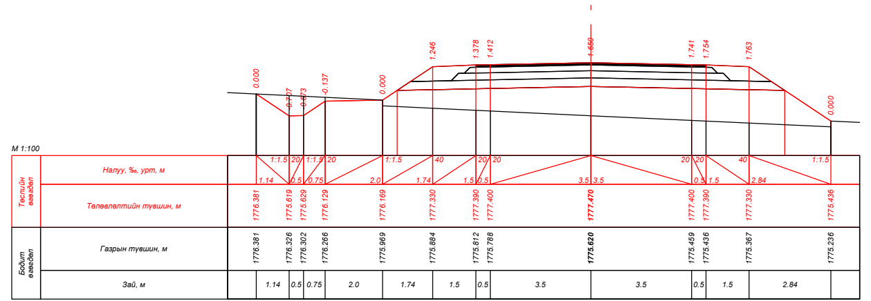
ПК 177+60.000
