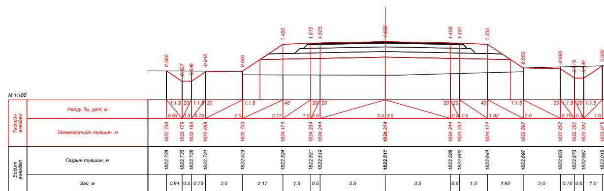
ПК 215+60.000
