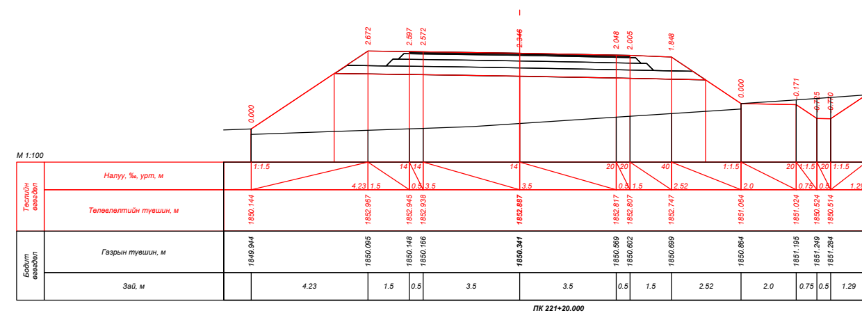
ПК 221+20.000
