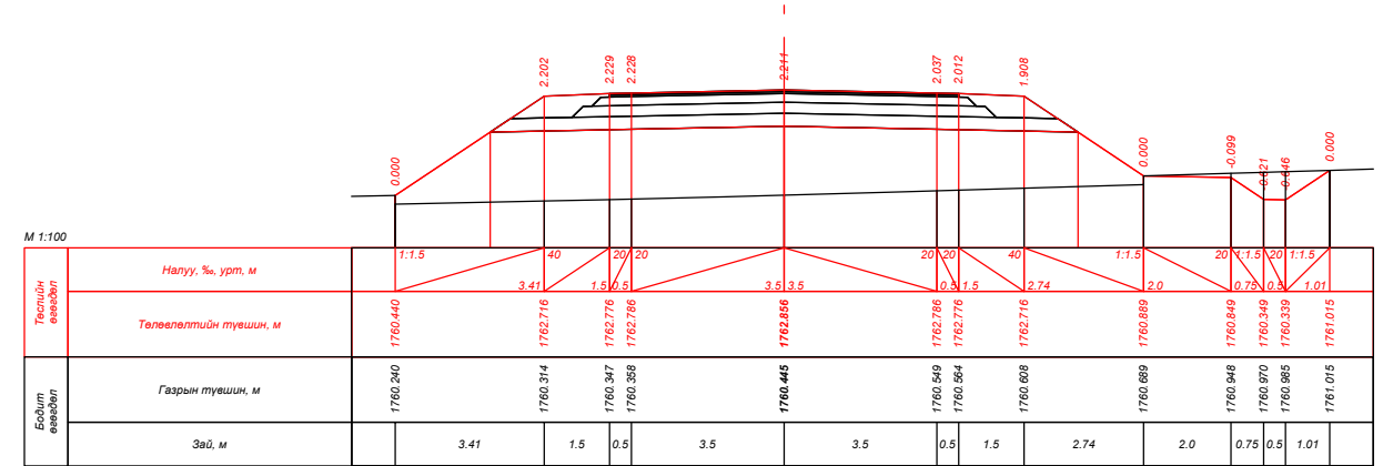
ПК 274+60.000
