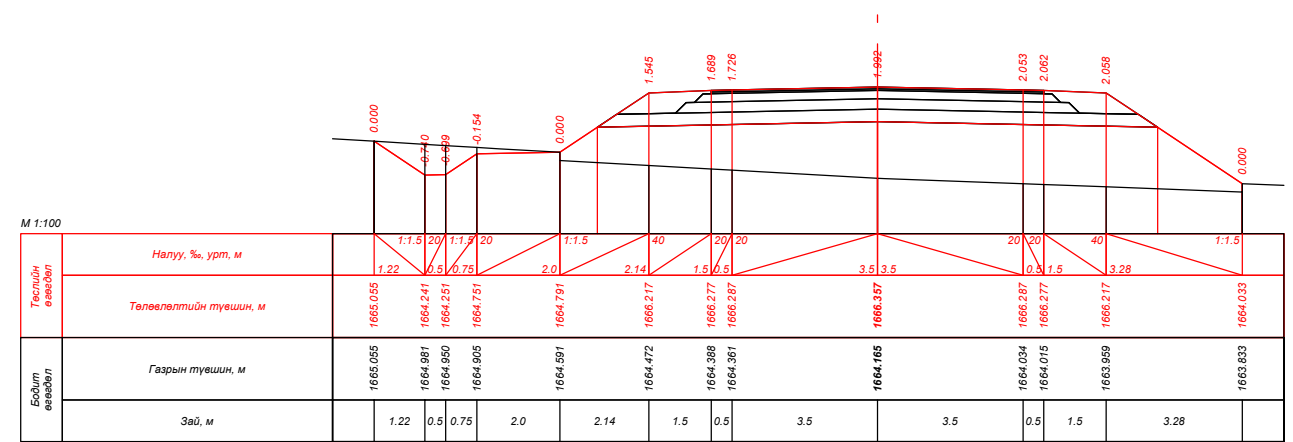
ПК 14+20.000
