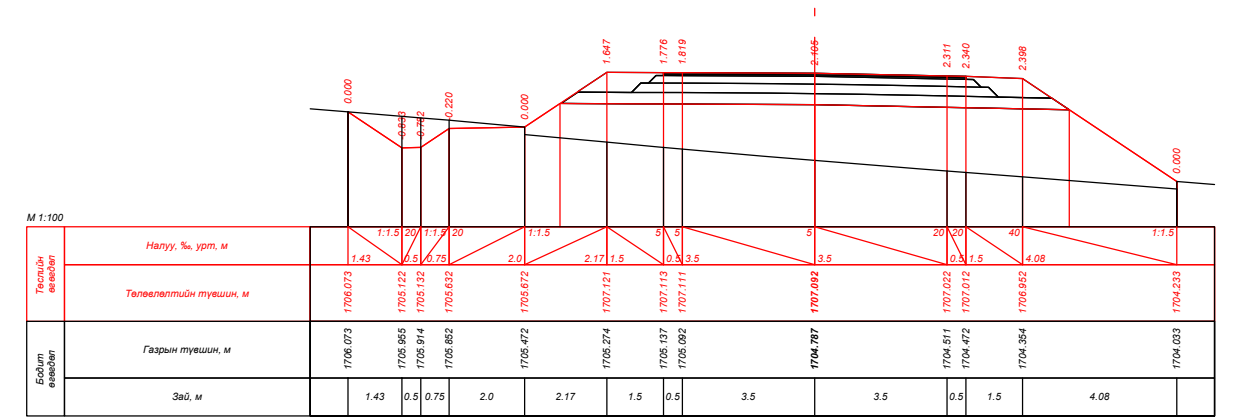
ПК 106+80.000
