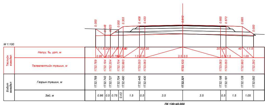
ПК 136+40.000
