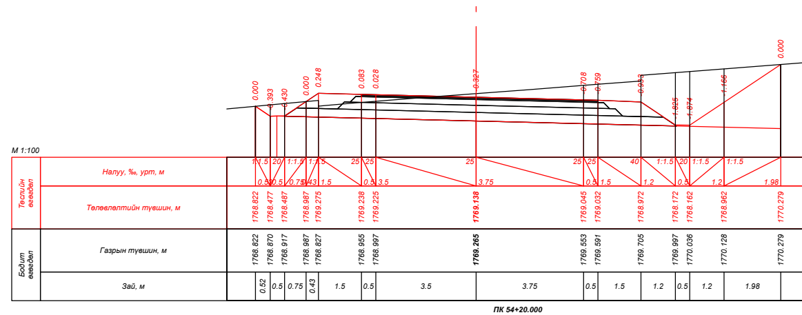
ПК 54+20.000
