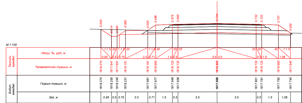
ПК 214+20.000
