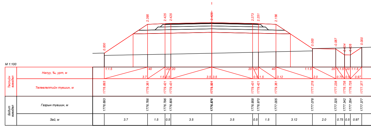
ПК 258+40.000
