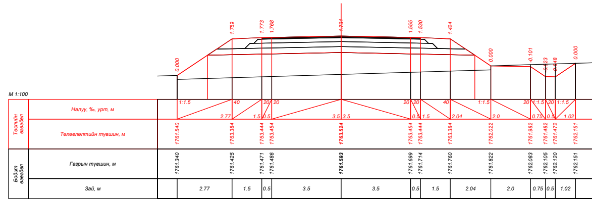
ПК 274+00.000
