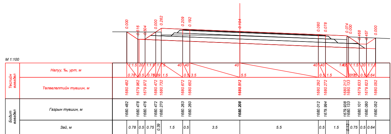
ПК 3+28.871
