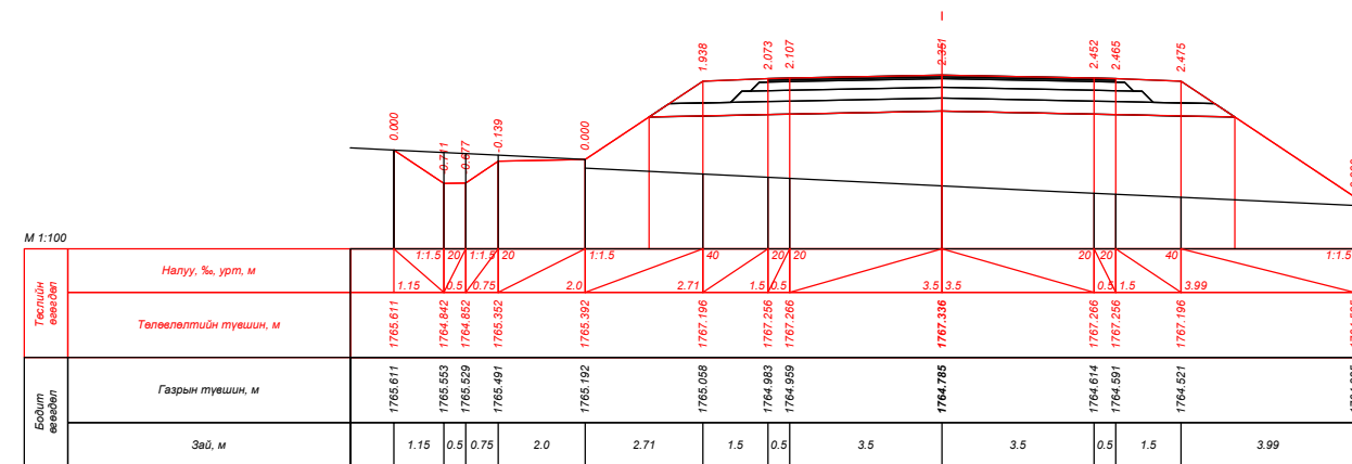
ПК 170+60.000
