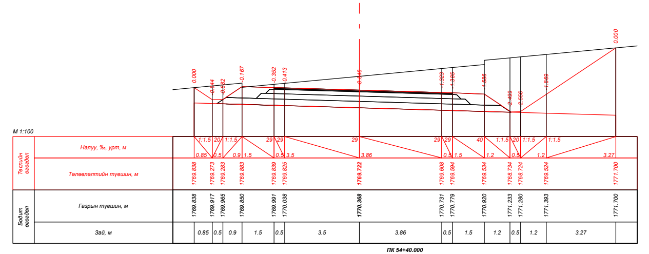
ПК 54+40.000
