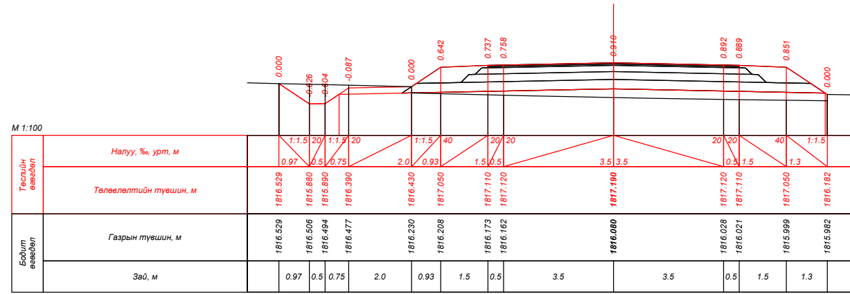
ПК 213+60.000
