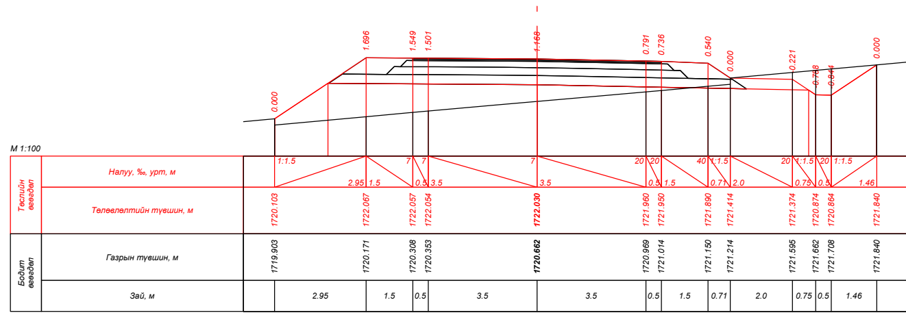
ПК 39+00.000
