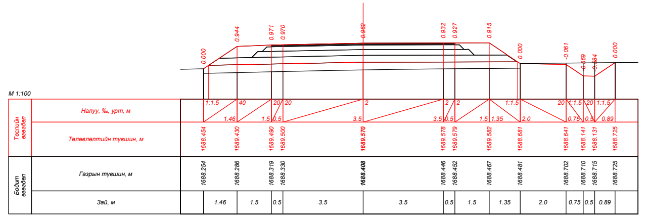
ПК 86+20.000
