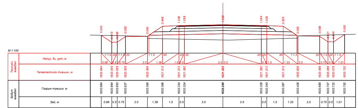
ПК 215+00.000
