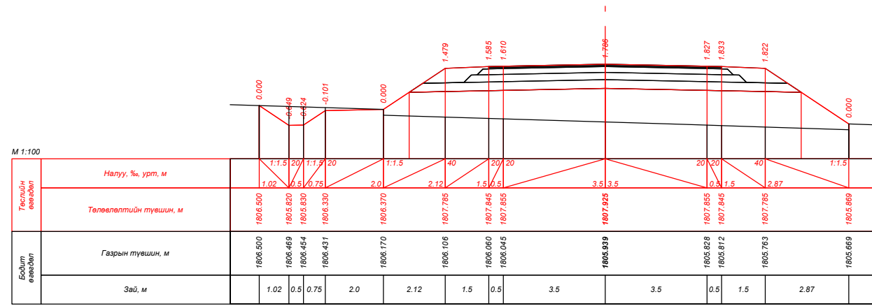
ПК 207+80.000
