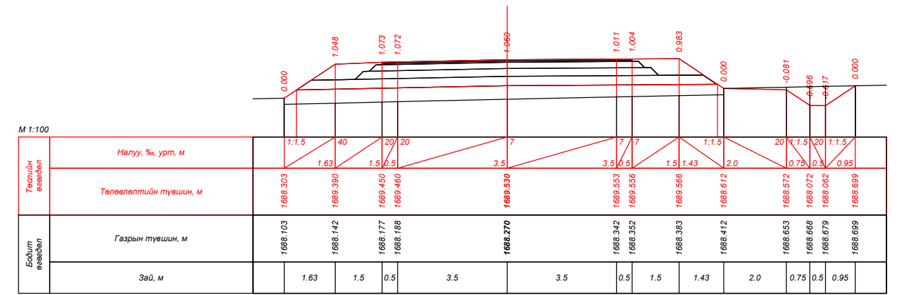
ПК 86+00.000
