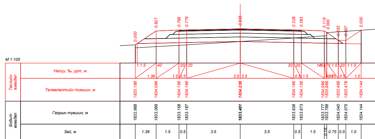
ПК 229+71.629
