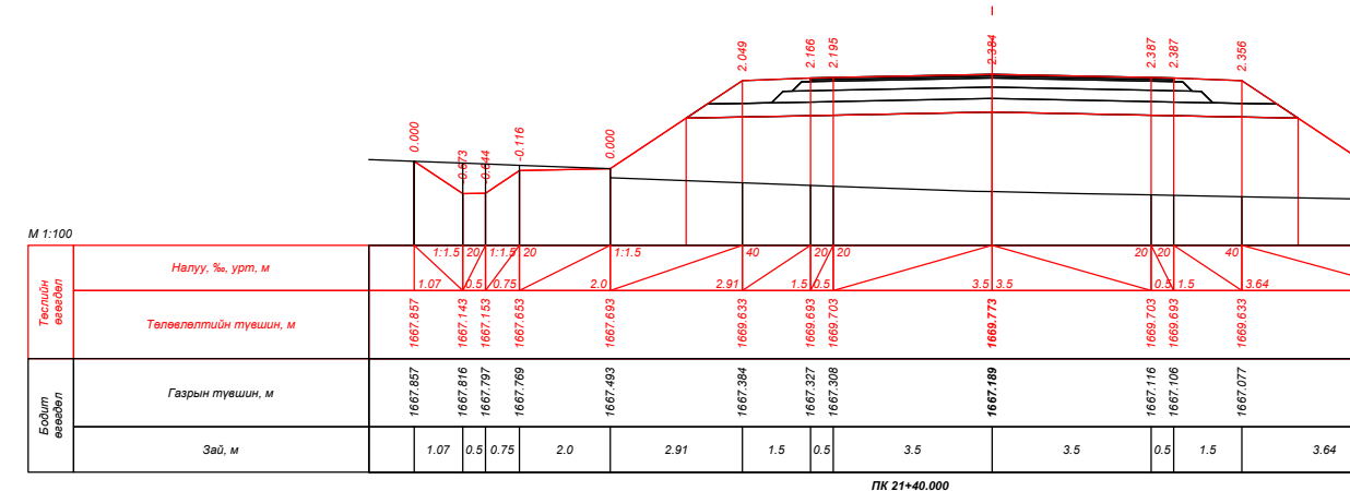
ПК 21+40.000
