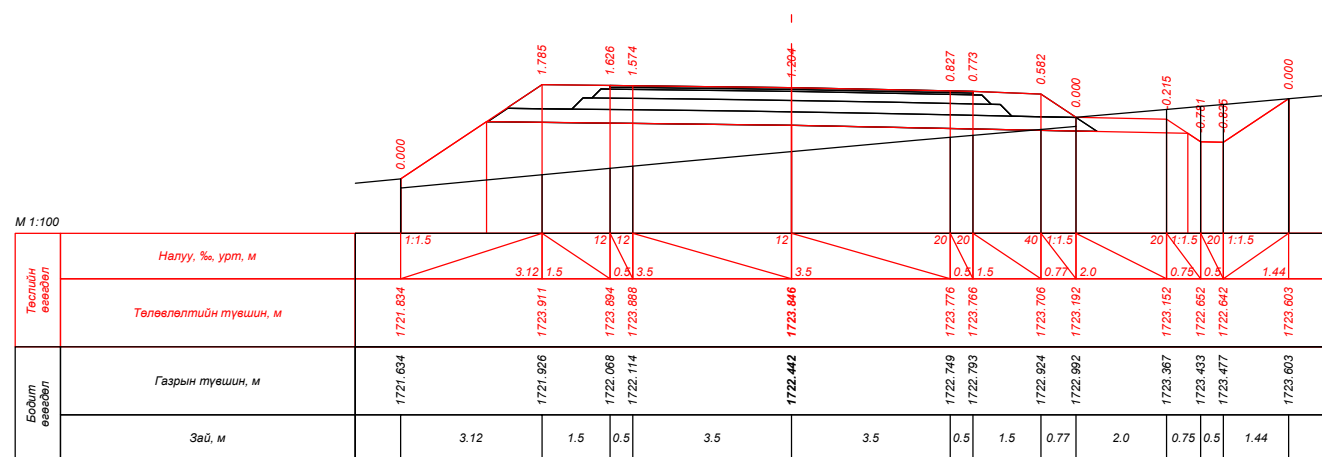
ПК 39+40.000
