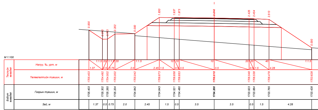
ПК 106+60.000
