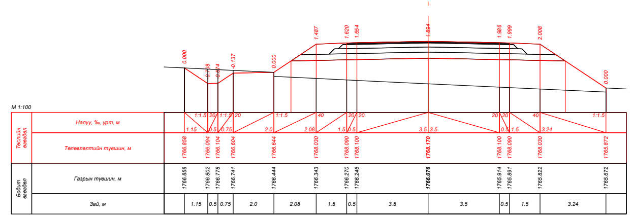
ПК 169+80.000
