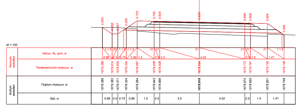
ПК 2+80.000
