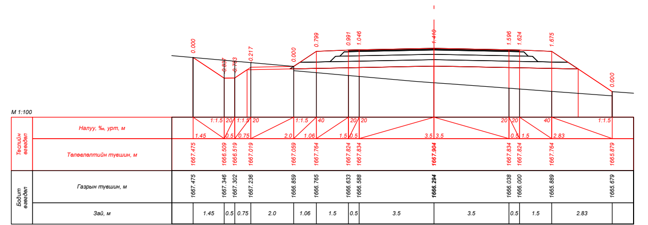
ПК 15+00.000
