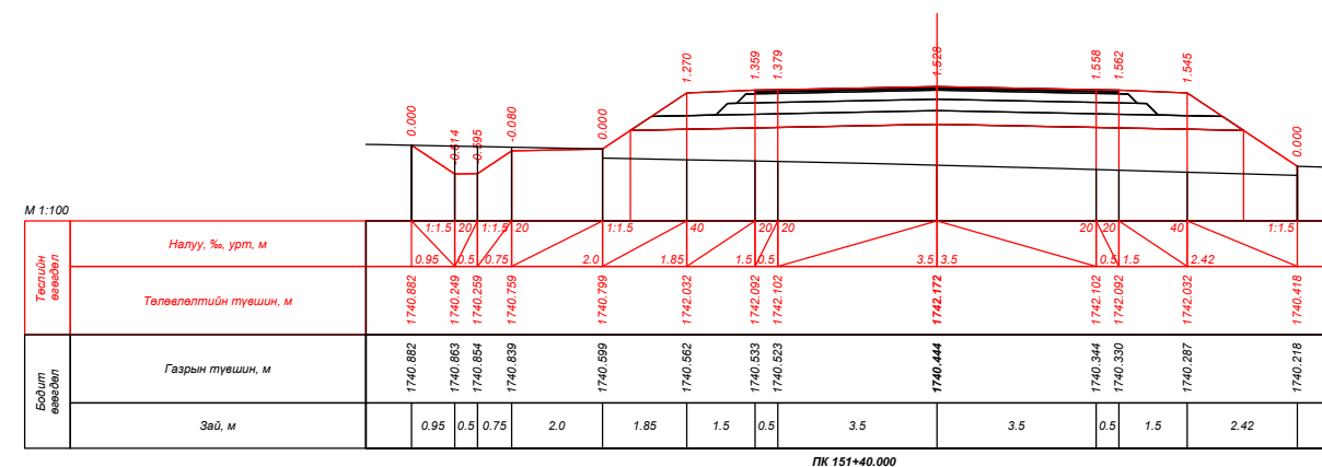
ПК 151+40.000
