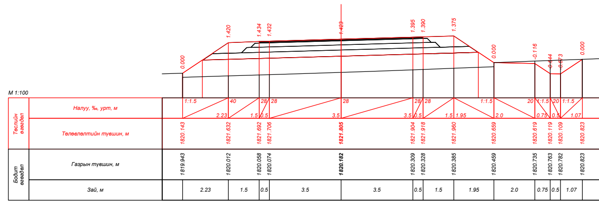
ПК 239+20.000
