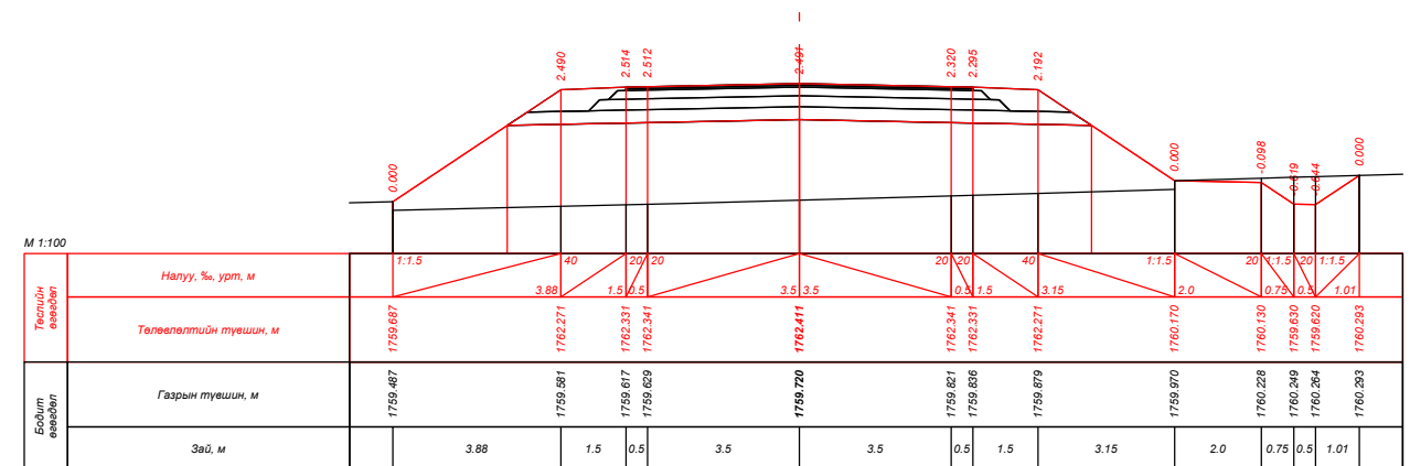
ПК 275+00.000
