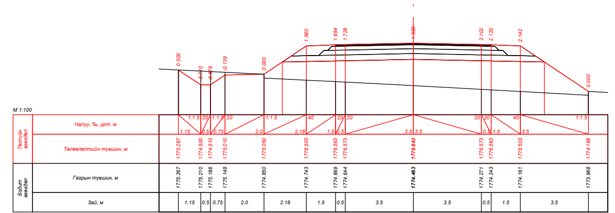
ПК 183+60.000
