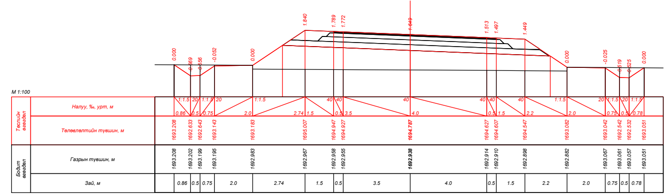
ПК 101+00.000
