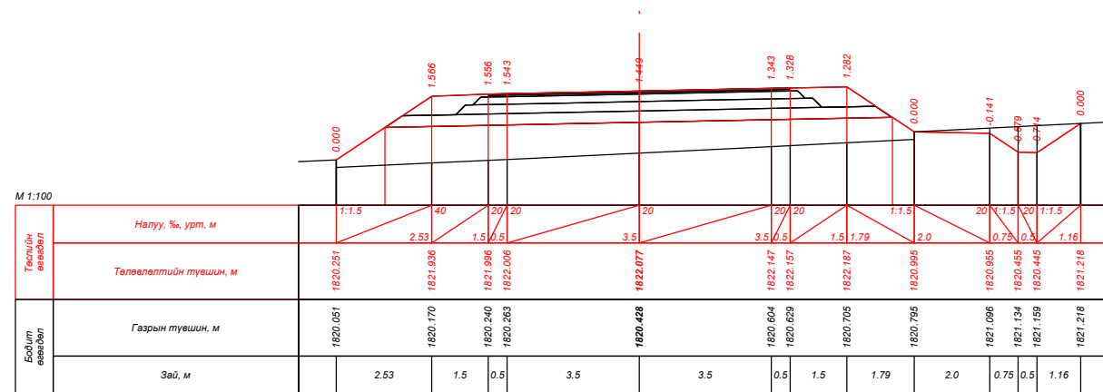
ПК 239+60.000
