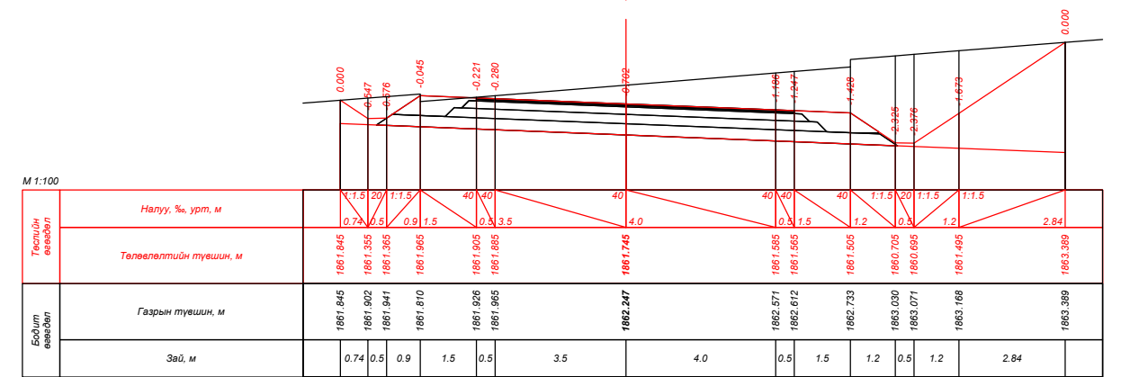
ПК 224+20.000
