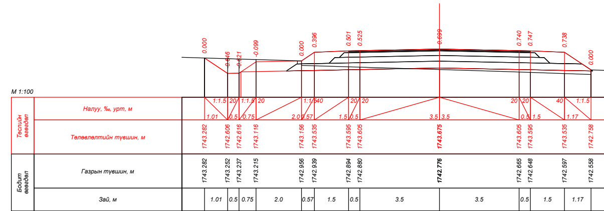
ПК 149+60.000
