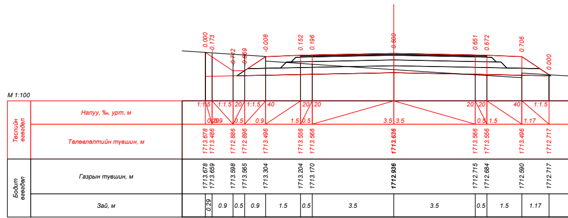
ПК 126+80.000
