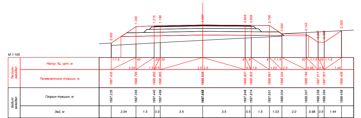
ПК 77+00.000
