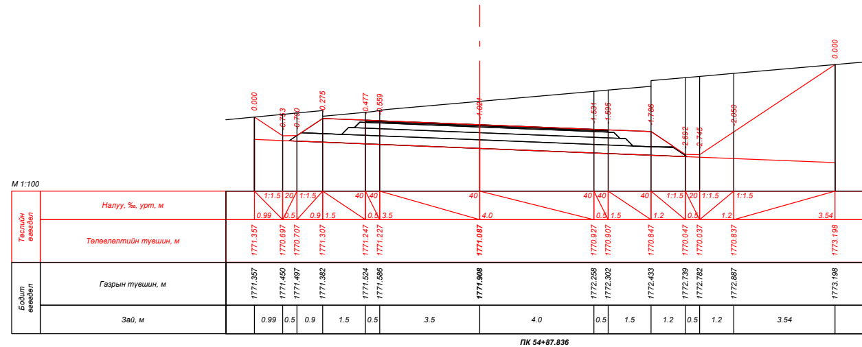
ПК 54+87.836
