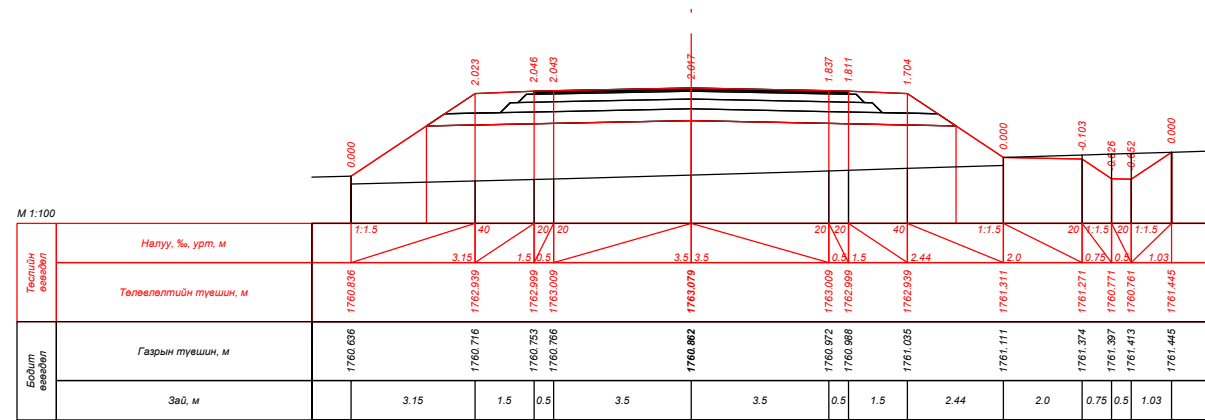
ПК 274+40.000
