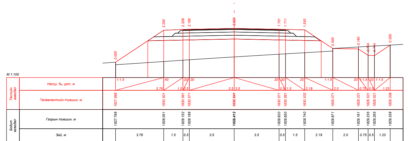
ПК 232+20.000
