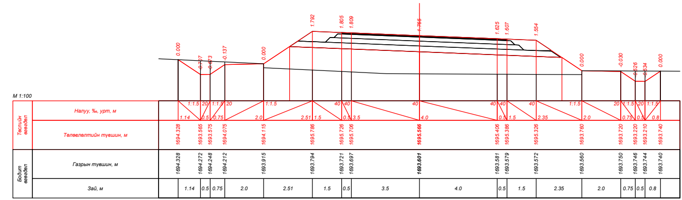
ПК 101+80.000
