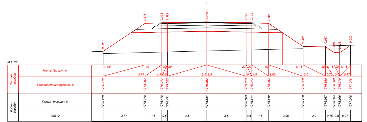
ПК 258+60.000
