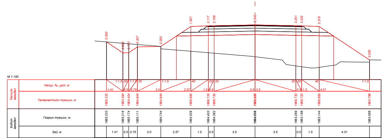
ПК 11+40.000
