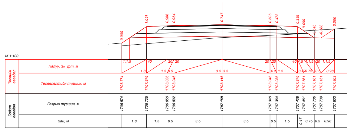
ПК 72+00.000
