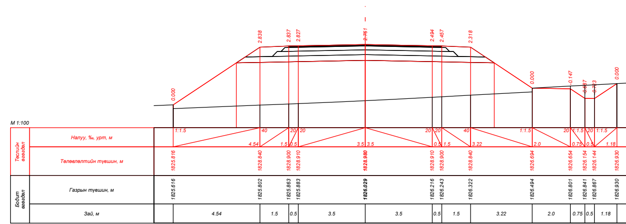
ПК 242+20.000
