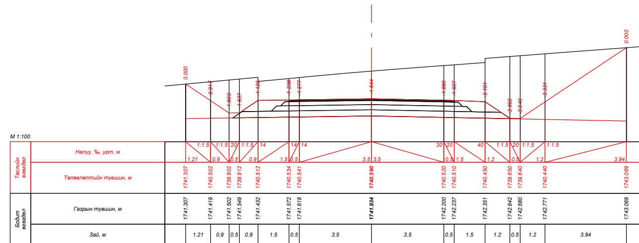
ПК 60+20.000
