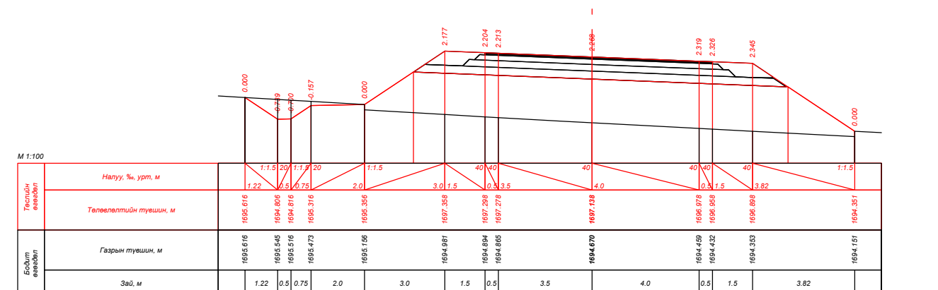
ПК 102+60.000
