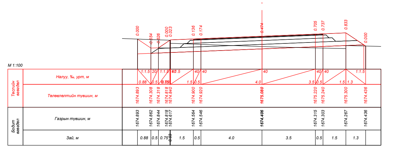
ПК 25+20.000
