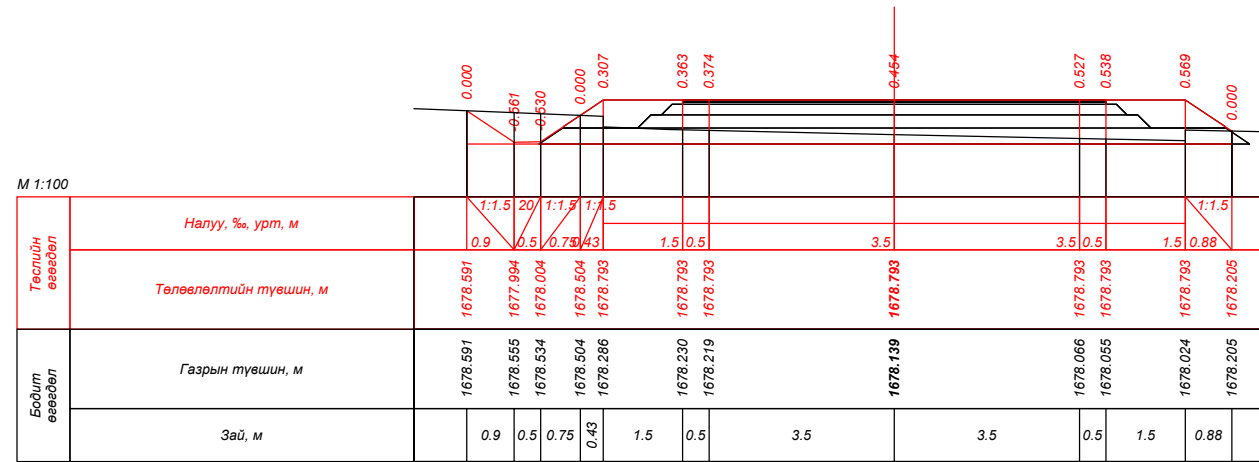
ПК 2+28.356
