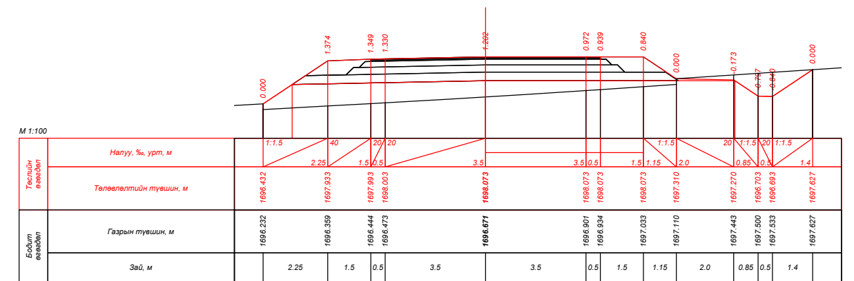
ПК 77+36.228
