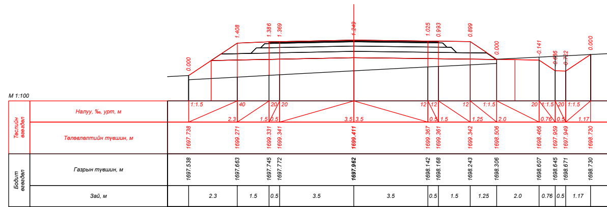
ПК 76+80.000
