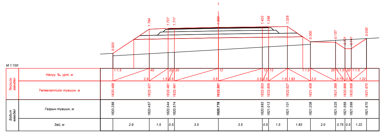
ПК 240+00.000
