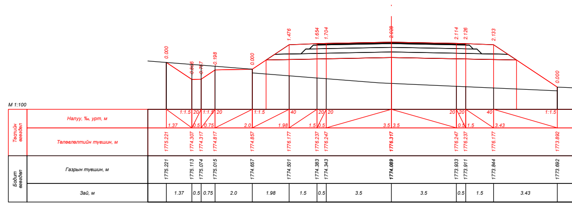
ПК 183+40.000
