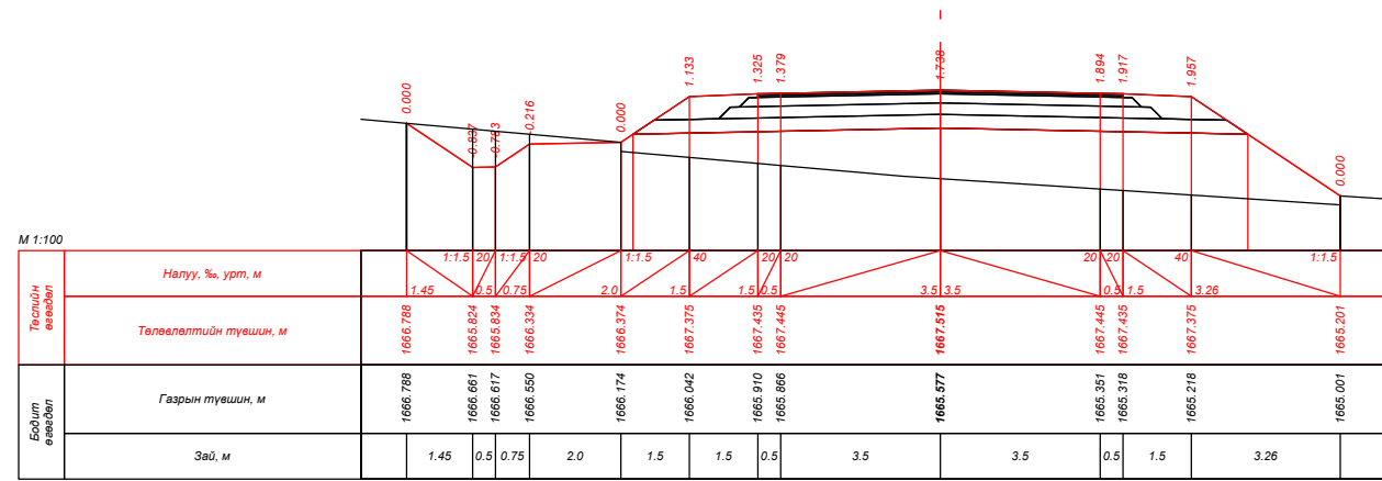
ПК 14+80.000
