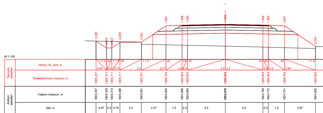
ПК 207+40.000
