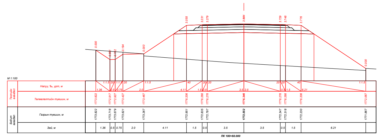
ПК 180+60.000
