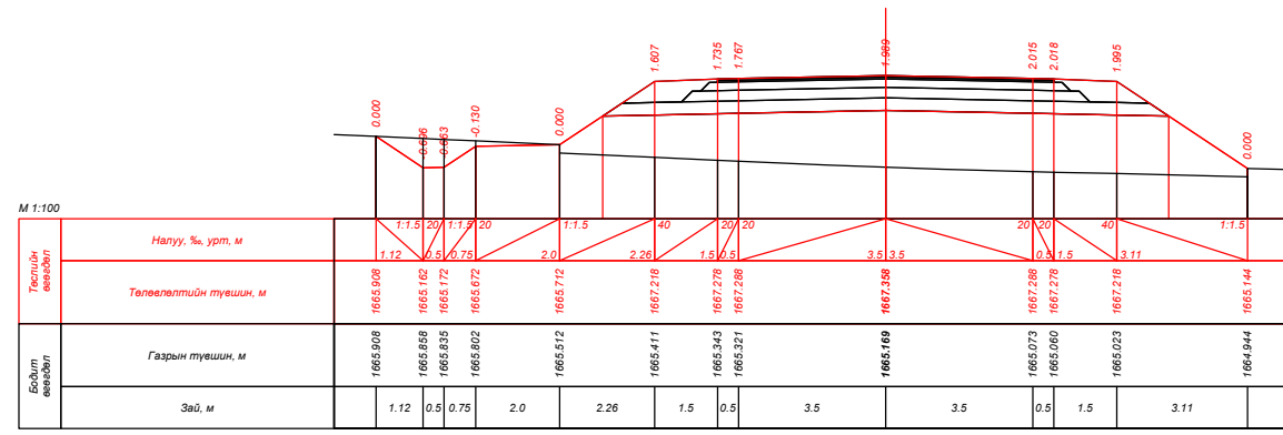
ПК 10+80.000
