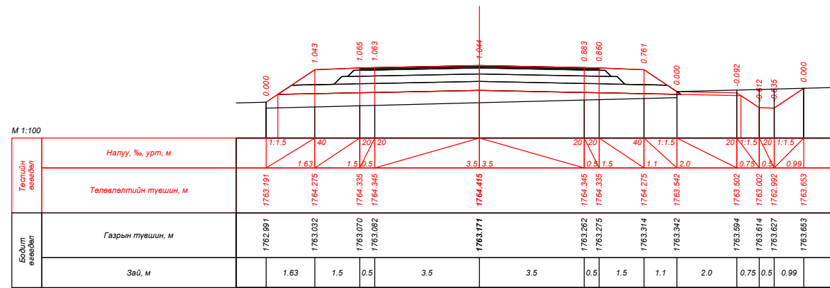
ПК 273+20.000
