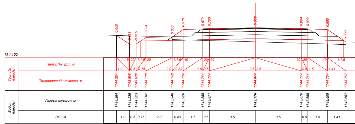
ПК 148+20.000
