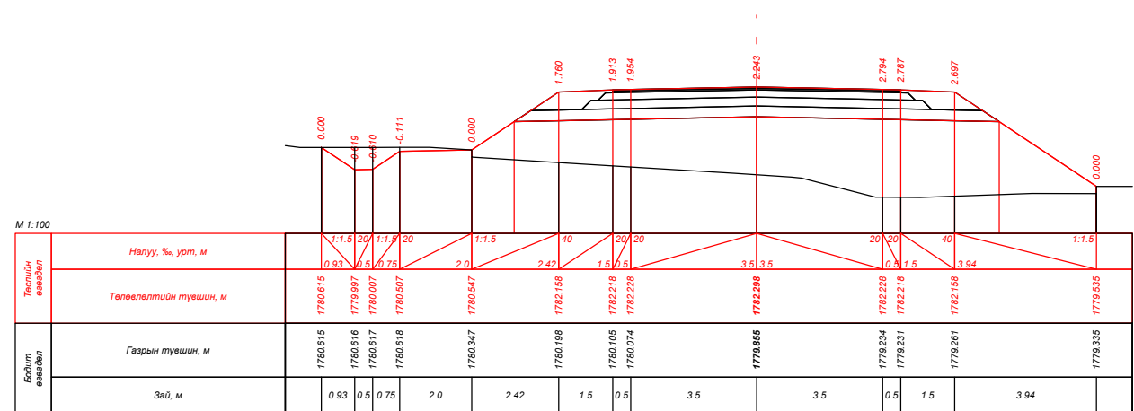
ПК 188+20.000
