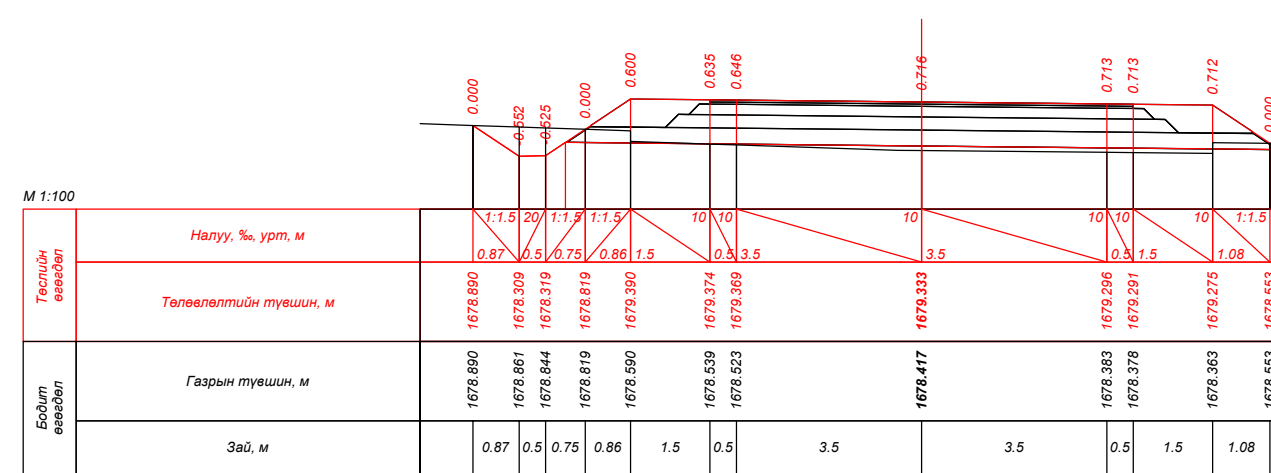
ПК 2+54.621
