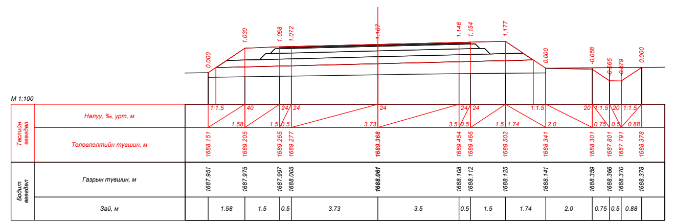
ПК 85+20.000
