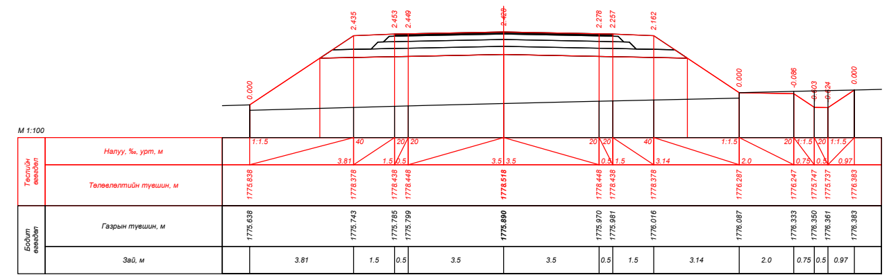
ПК 259+00.000
