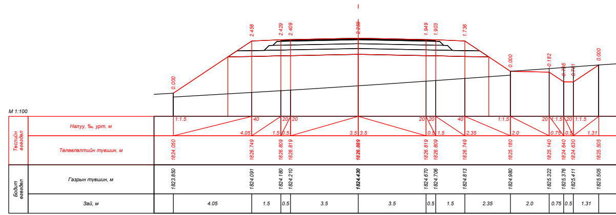
ПК 241+66.973
