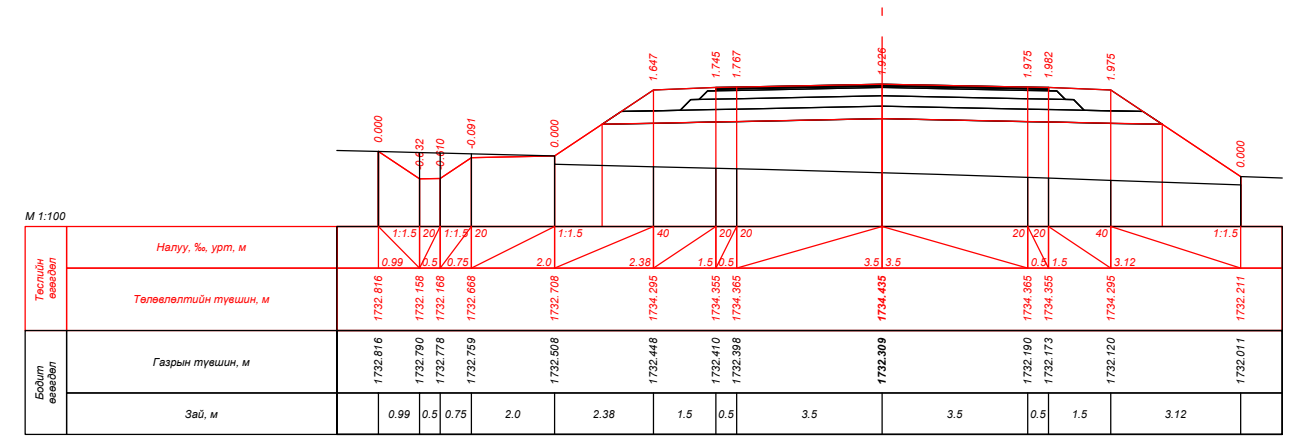
ПК 138+20.000
