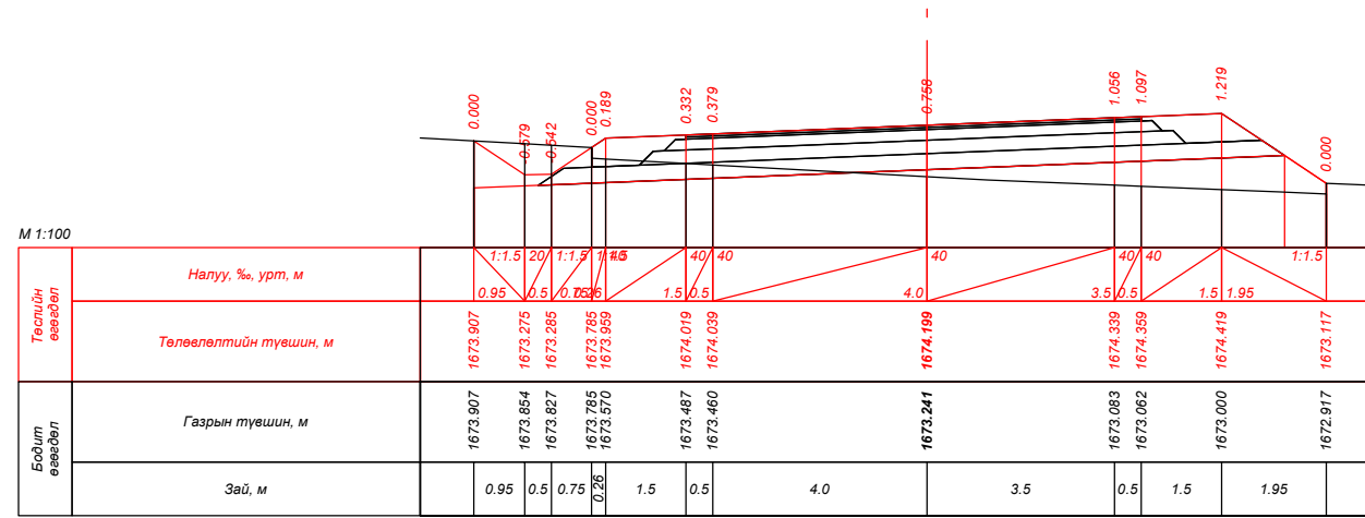
ПК 24+60.000
