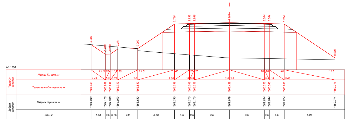
ПК 11+80.000
