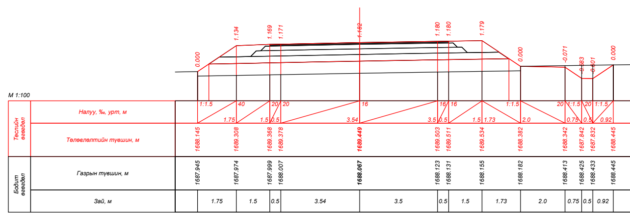
ПК 85+60.000
