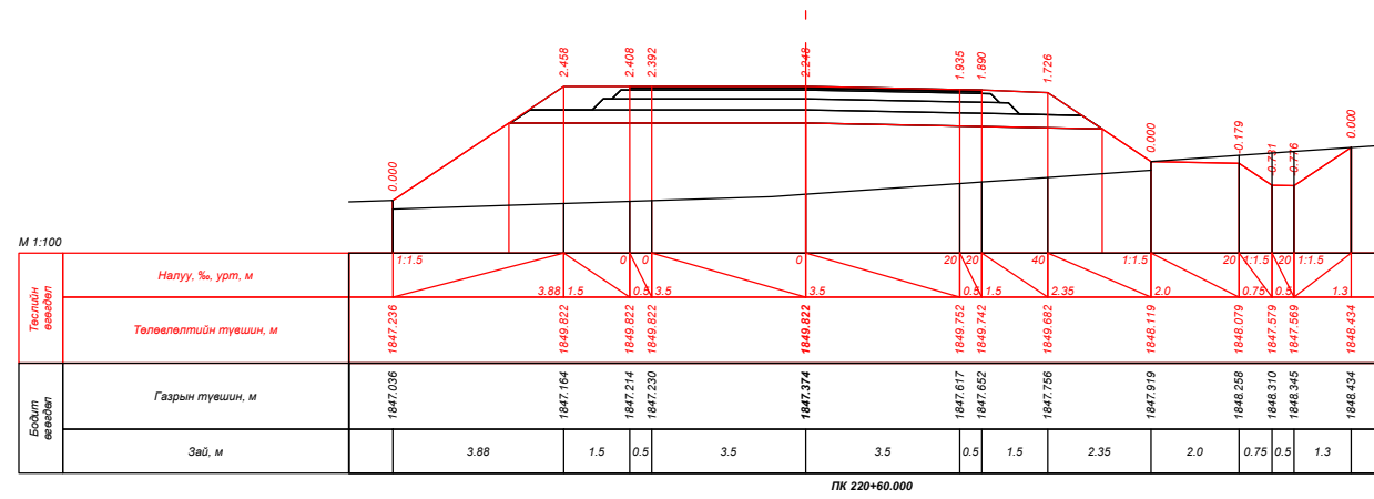
ПК 220+60.000
