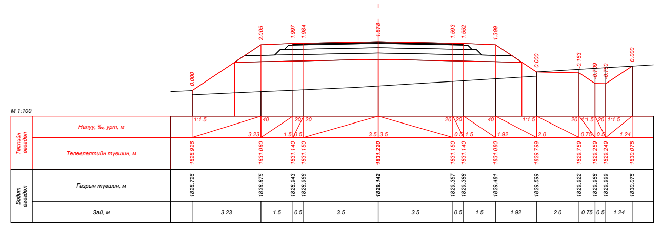
ПК 231+80.000
