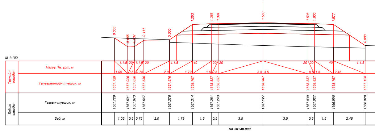
ПК 20+40.000
