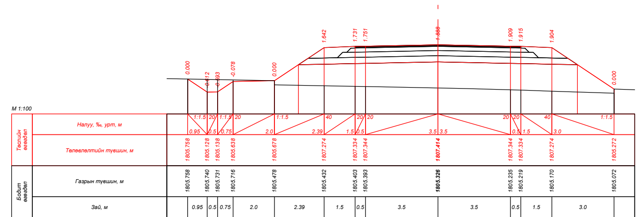
ПК 207+60.000
