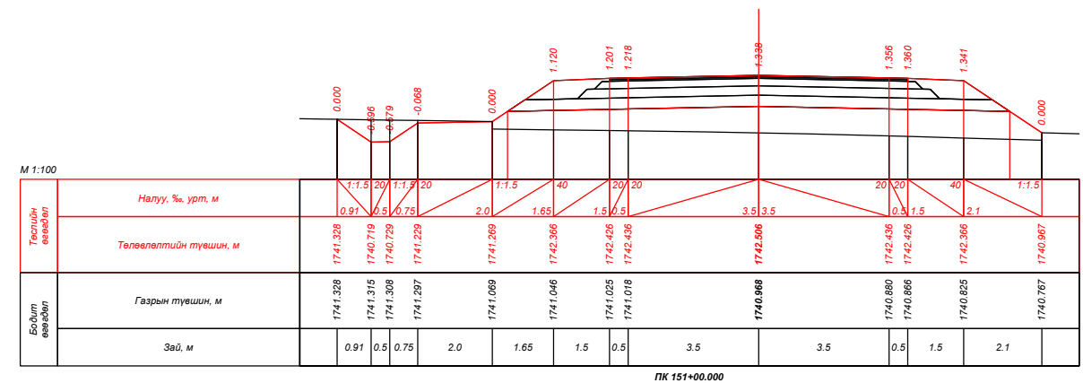
ПК 151+00.000
