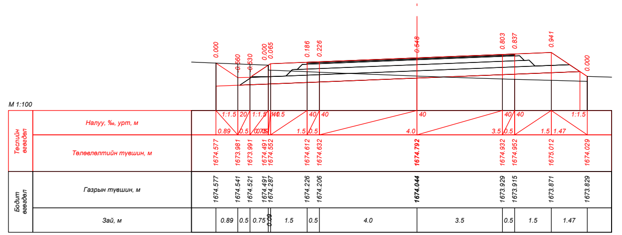
ПК 25+00.000
