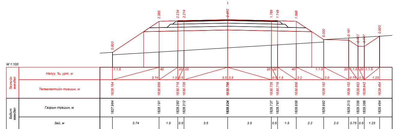
ПК 232+09.269
