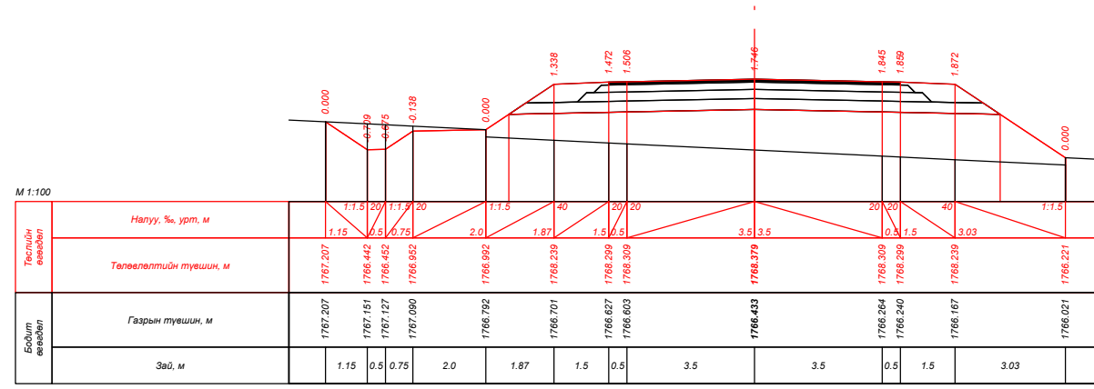
ПК 169+60.000
