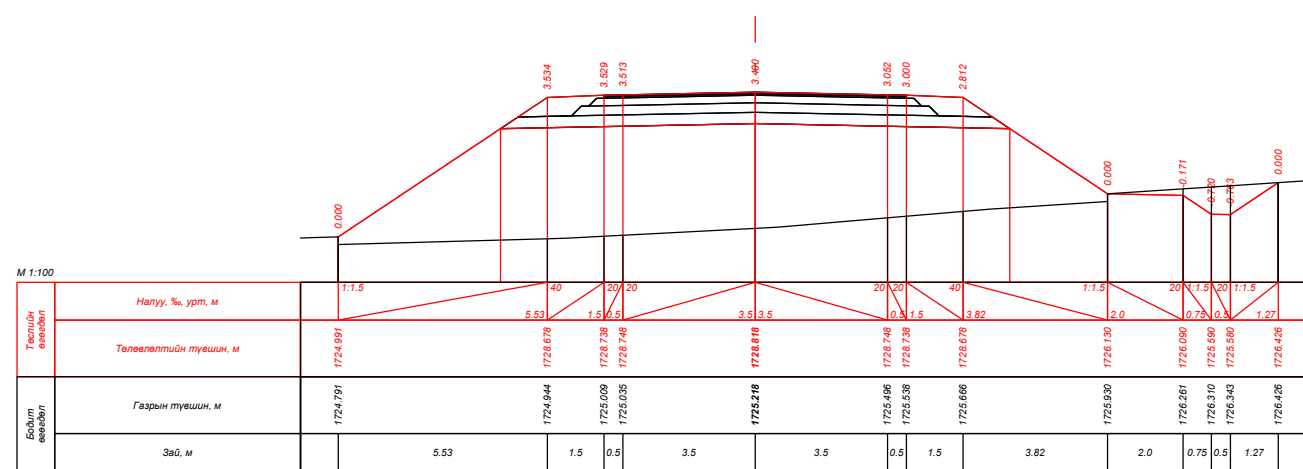
ПК 62+80.000
