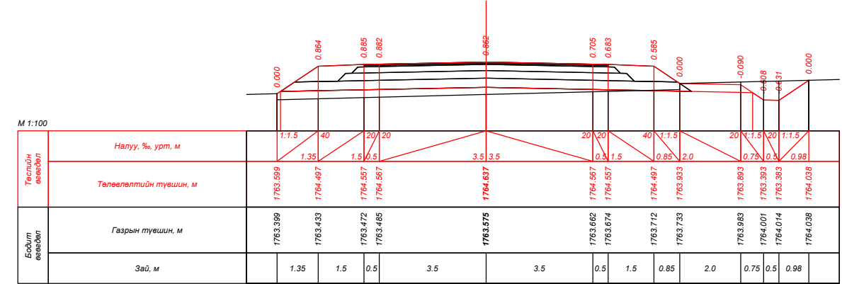
ПК 273+00.000
