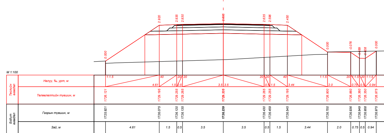
ПК 62+60.000
