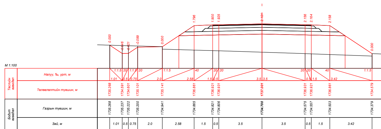
ПК 139+80.000
