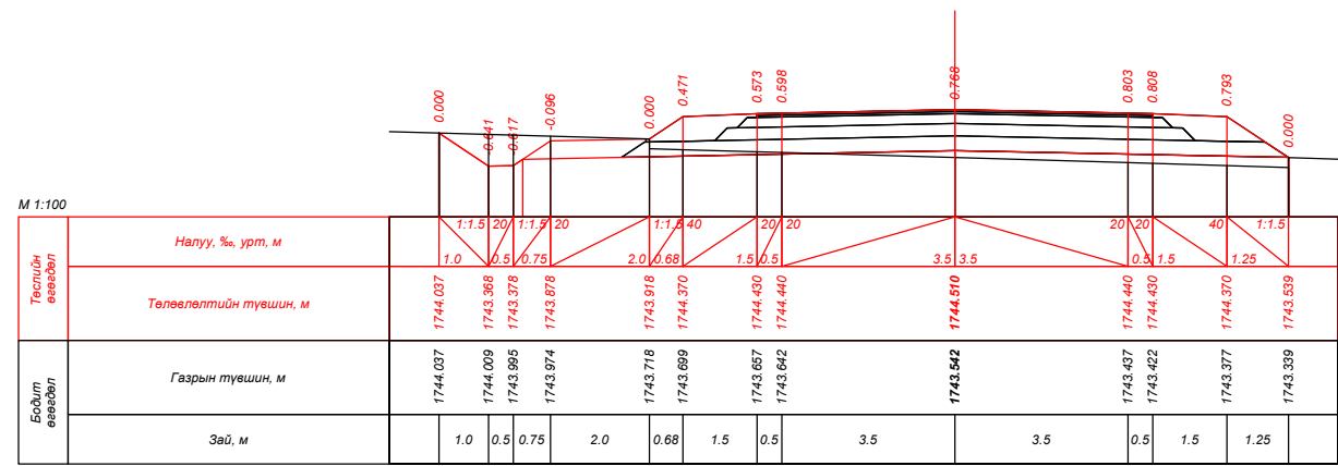
ПК 148+60.000
