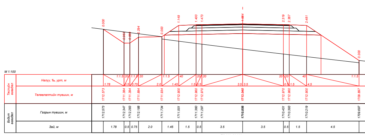
PK 110+80.000
