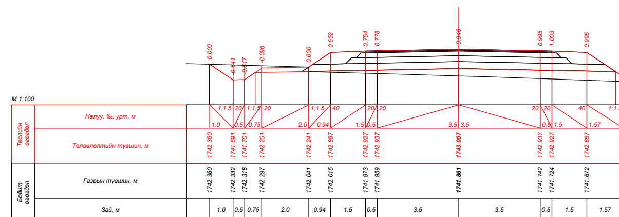
ПК 150+40.000
