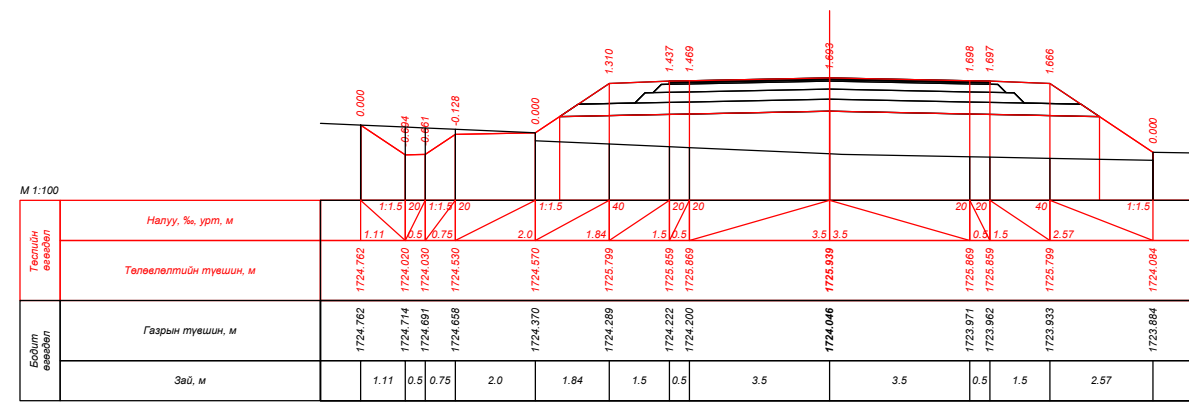
ПК 132+80.000
