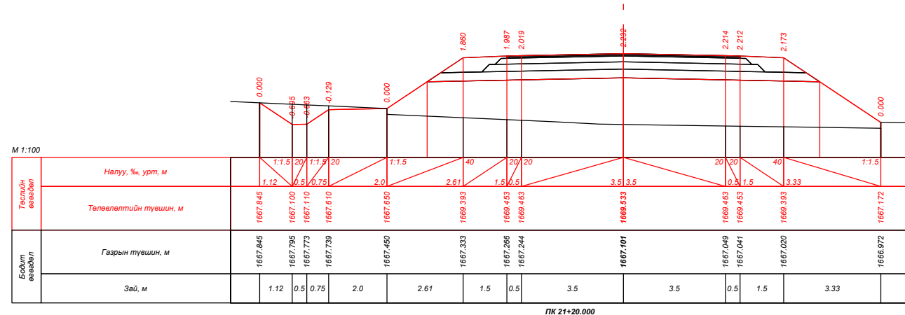
ПК 21+20.000
