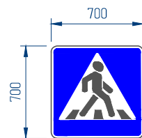
5.19a Явган хүний гарц
