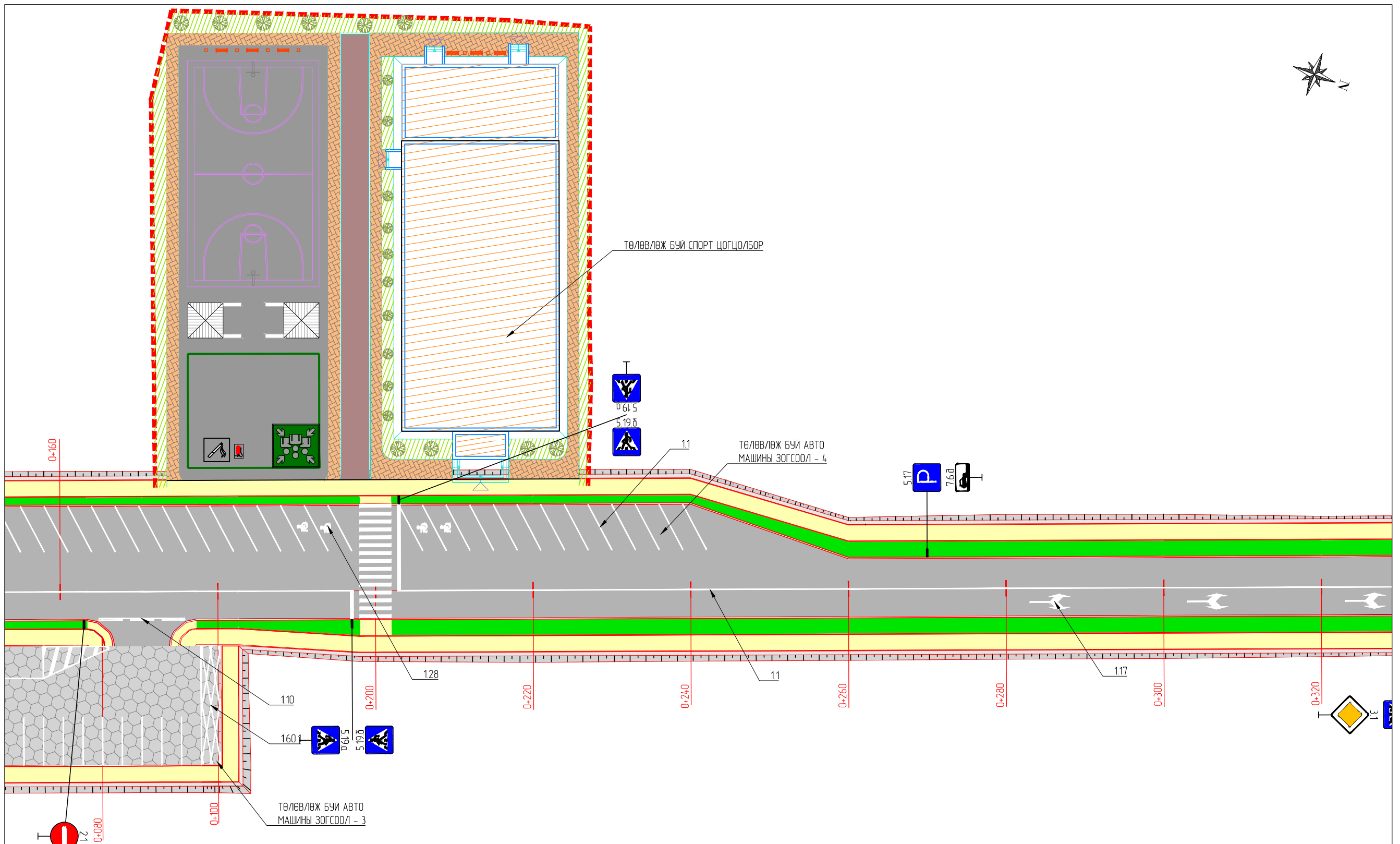
ТҮЛХҮҮР ЗУРАГ
