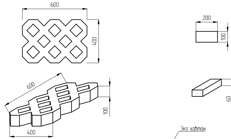
АШИГЛАХ МАТЕРИАЛЫН ХЭМЖЭЭС
