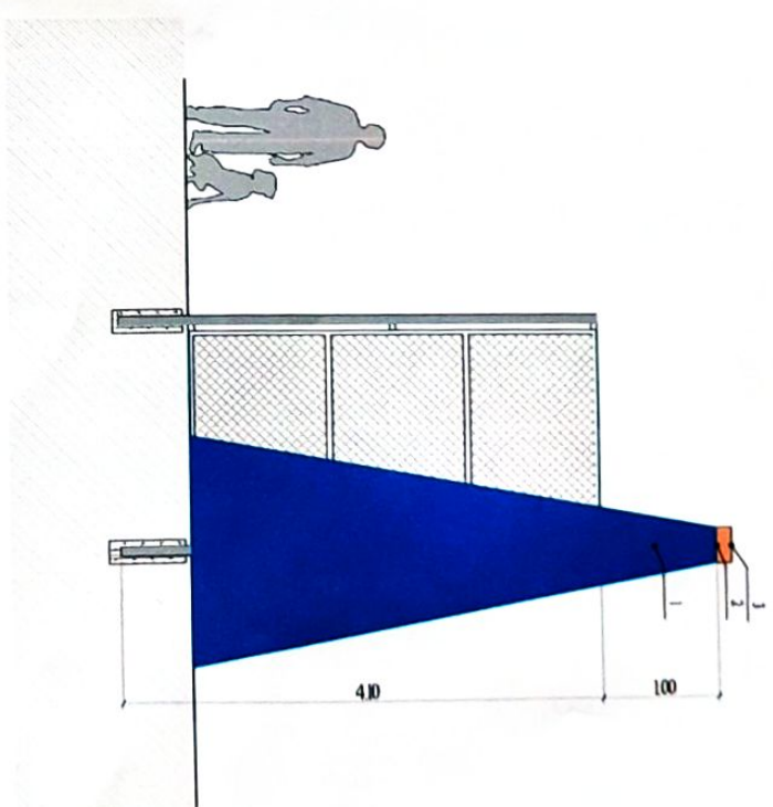
ХЭСГИЛЭЛ 1 М1:50 ГЭРЭЛТҮҮЛЭГТИЙН ХЭСГИЛЭЛ
