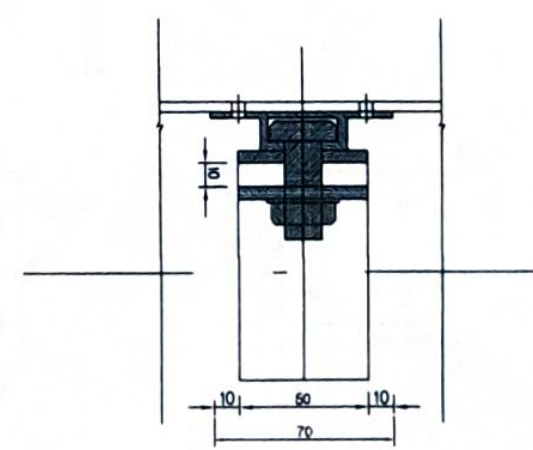
Н хэсгийн
