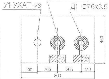
Сувгийн огтлол J-J
