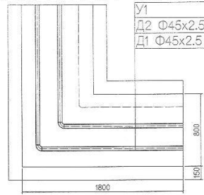
ЭРГЭЛТИЙН ӨНЦӨГ ЭӨ-5,22-ИЙН БАЙГУУЛАЛТ М1:40
