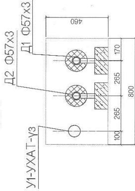
Сувгийн огтлол В-В М1:25
