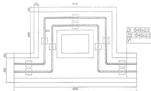
КОМПЕНСАТОР-7,12-ИЙН БАЙГУУЛАЛТ М1:40
