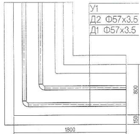
ЭРГЭЛТИЙН ӨНЦӨГ ЭӨ-1,2,3,4,23,24-ИЙН БАЙГУУЛАЛТ М1:40
