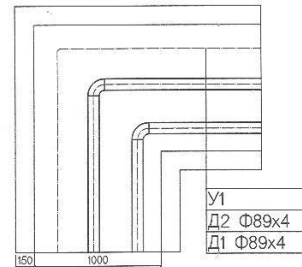
ЭРГЭЛТИЙН ӨНЦӨГ ЭӨ-8,9-ИЙН БАЙГУУЛАЛТ М1:40
