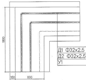
ЭРГЭЛТИЙН ӨНЦӨГ ЭӨ-7,13,16,17,18,27-ИЙН БАЙГУУЛАЛТ М1:40
