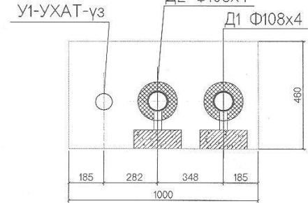
Сувгийн огтлол E-E
