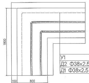
ЭРГЭЛТИЙН ӨНЦӨГ ЭӨ-14,15,19,20,25,26,28,29,30,31,32,33,34-ИЙН БАЙГУУЛАЛТ М1:40
