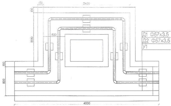
КОМПЕНСАТОР-1,11-ИЙН БАЙГУУЛАЛТ М1:40
