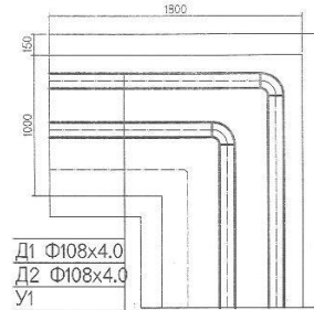
ЭРГЭЛТИЙН ӨНЦӨГ ЭӨ-6-ИЙН БАЙГУУЛАЛТ М1:40
