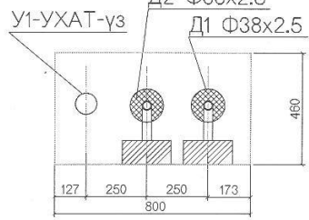
Сувгийн огтлол L-L
