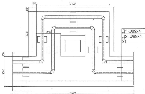
КОМПЕНСАТОР-5,6,8-ИЙН БАЙГУУЛАЛТ М1:40
