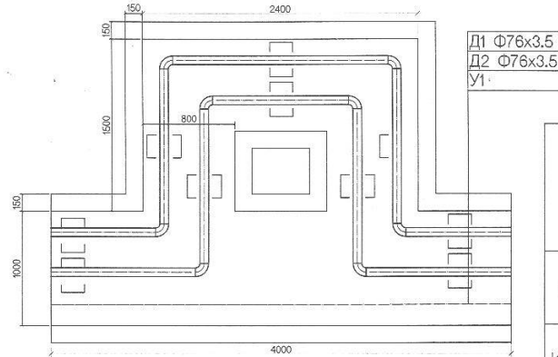
КОМПЕНСАТОР-9,10-ИЙН БАЙГУУЛАЛТ М1:40
