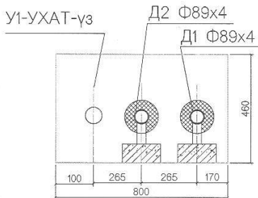
Сувгийн огтлол F-F
