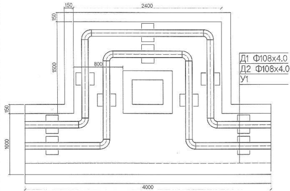
КОМПЕНСАТОР-5,6,8-ИЙН БАЙГУУЛАЛТ М1:40
