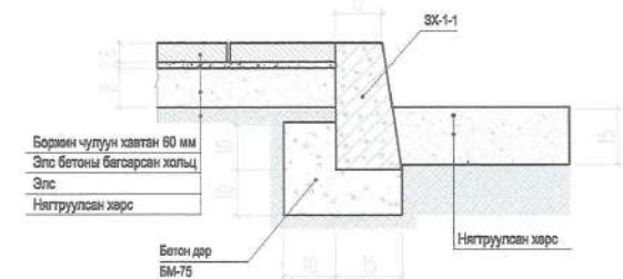
Хучилттай явган зам ба сайжруулсан шороон зам Огтлол 1-1
