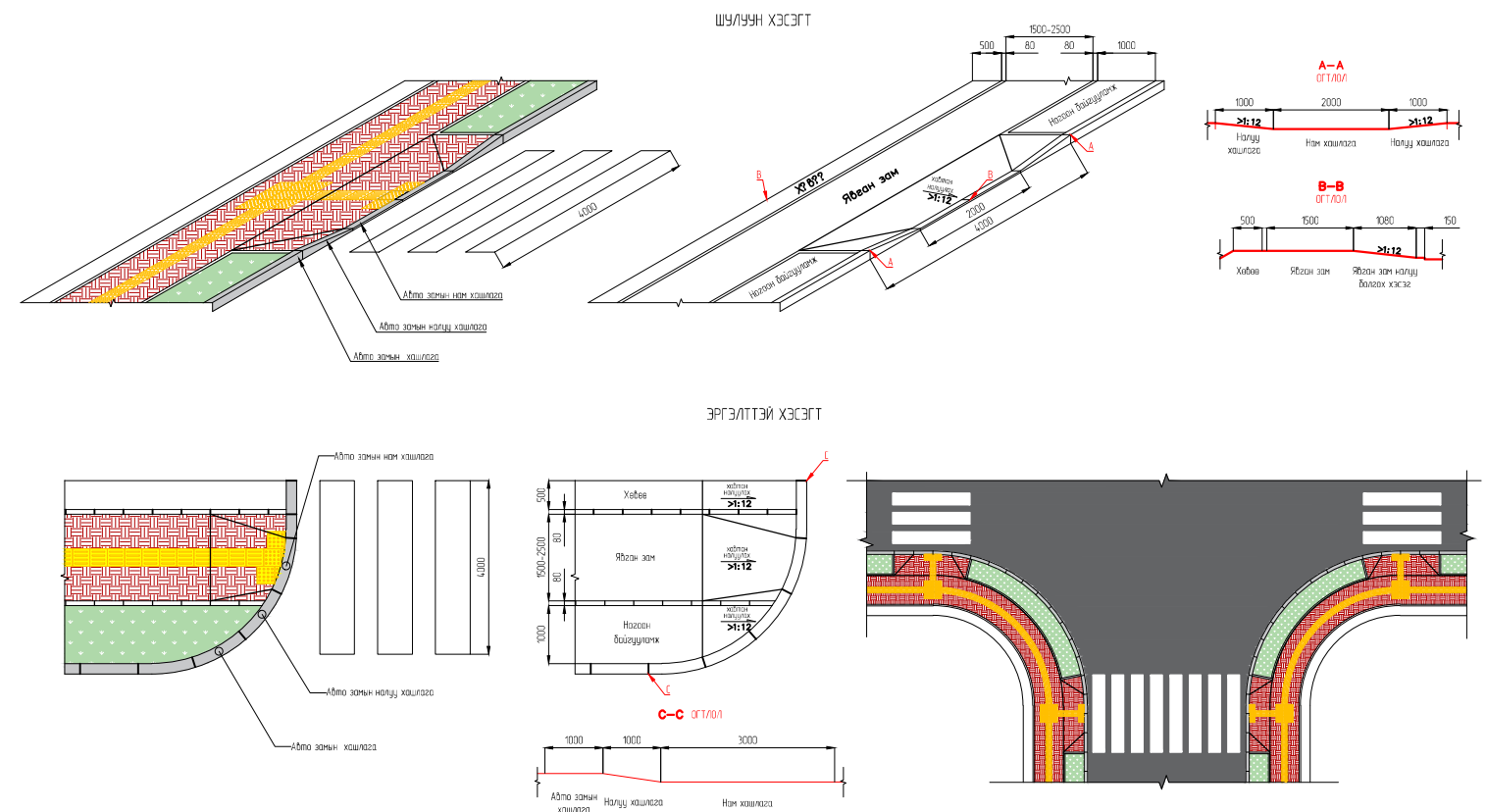
Зураг 11. Явган хүний гарц дээрх явган замыг хийх аргачлал
