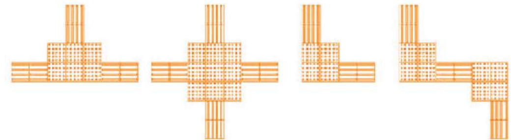
Зураг 10. Хөтөч хавтан өрөх (Жишээ)
