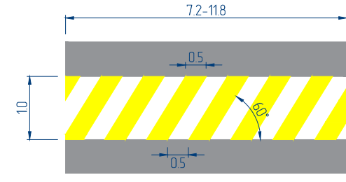
123 Хурд саазуурыг тэмдэглэх
