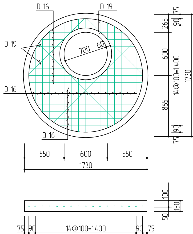
Зураг 6. Хүзүүвчний нарийвчилсан зураг
