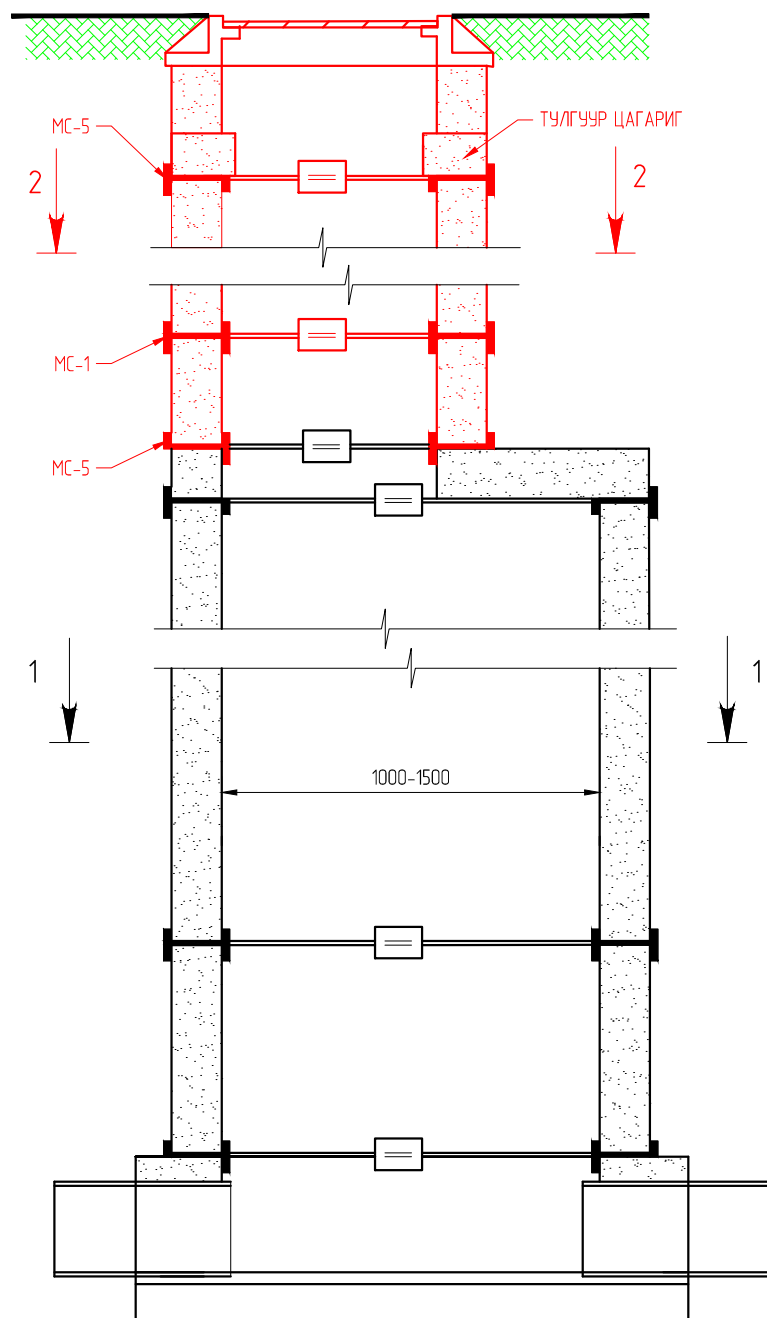
ТӨМӨРБЕТОН ХУДАГ ӨНДӨРЛӨХ СХЕМ
