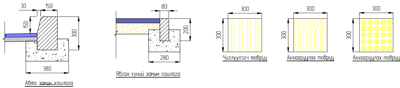
Зураг 8. Авто зам болон явган хүний замын хашлага, чиглүүлэгч хавтангийн хэмжээс
