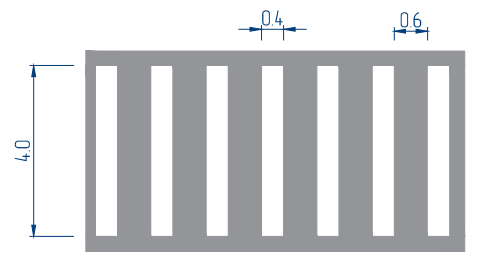
1.13.а Захицуулдаггүй явган хүний гарц
