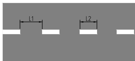
1.5 Тээврийн хэрэгсэлийн эсрэг урсгалыг тусгаарлах ( V<60 км/цаг; L2=1.00-3.00; L1=3.00-9.00 )
