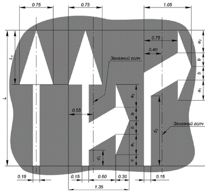
4.1б Баруун гар тийш явна
