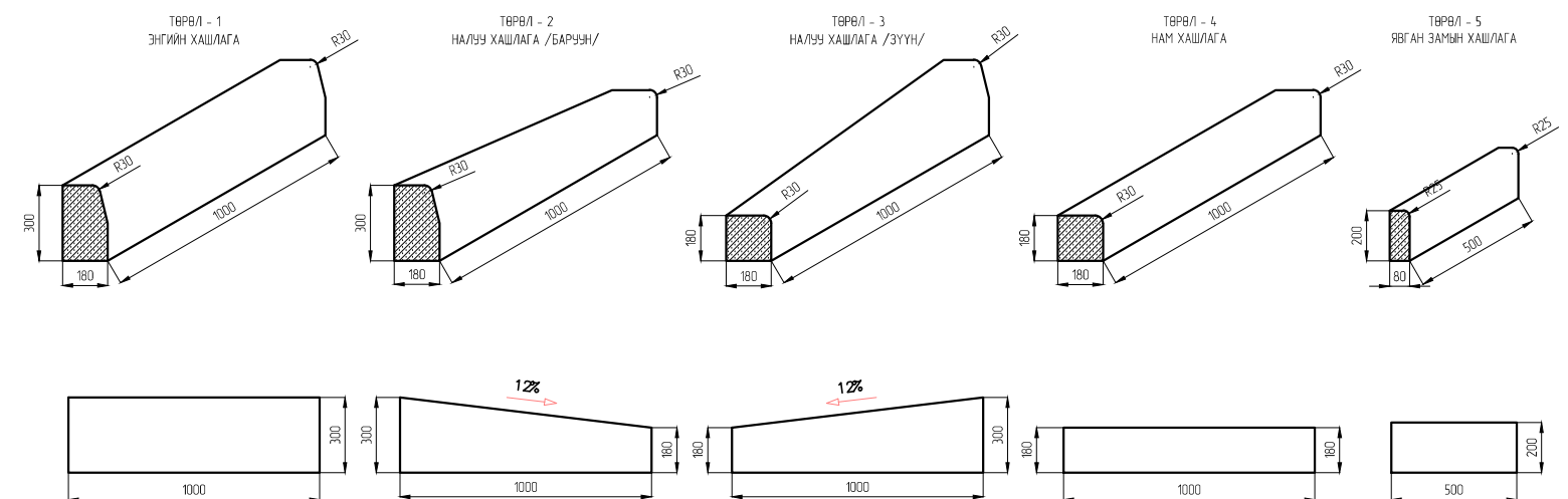
Зураг 7. Авто зам болон явган хүний замын хашлагын хэмжээс
