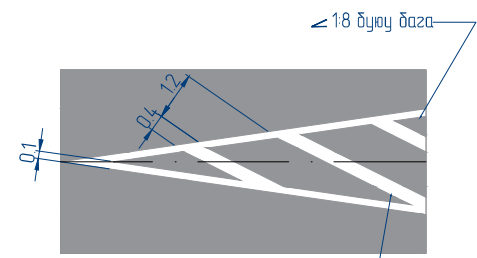
1.15.а Тээврийн хэрэгслийн хөдөлгөөний эсрэг урсгалыг тусгаарласан арлыг тэмдэглэх.
