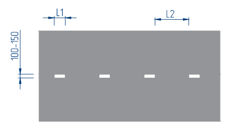
15 Тээврийн хэрэгцэлийн эсрэг урсгалыг тусгаарлах (V<60 км/цаг; L2=100-300; L1=300-900)
