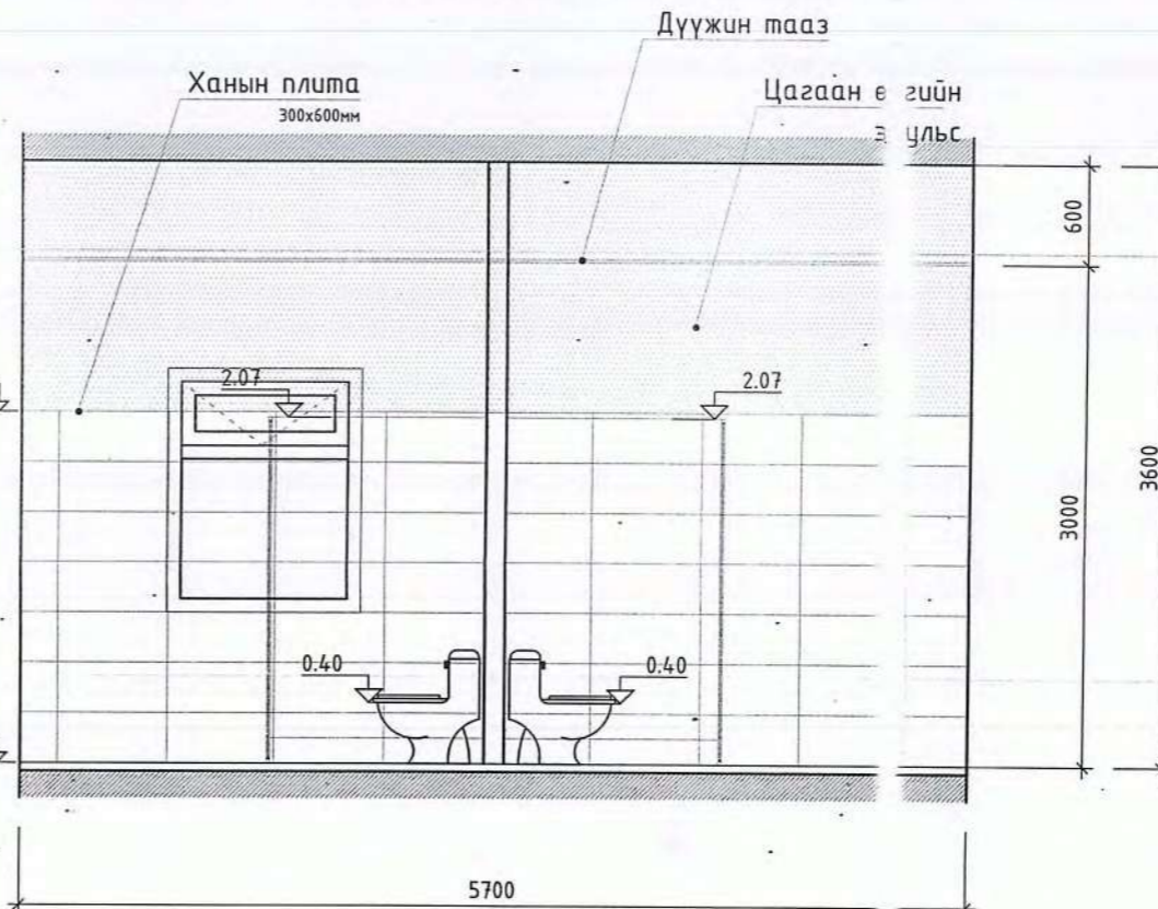
Огтлол 1-1 /Эрэгтэй ариун цэврийн өрөө/
