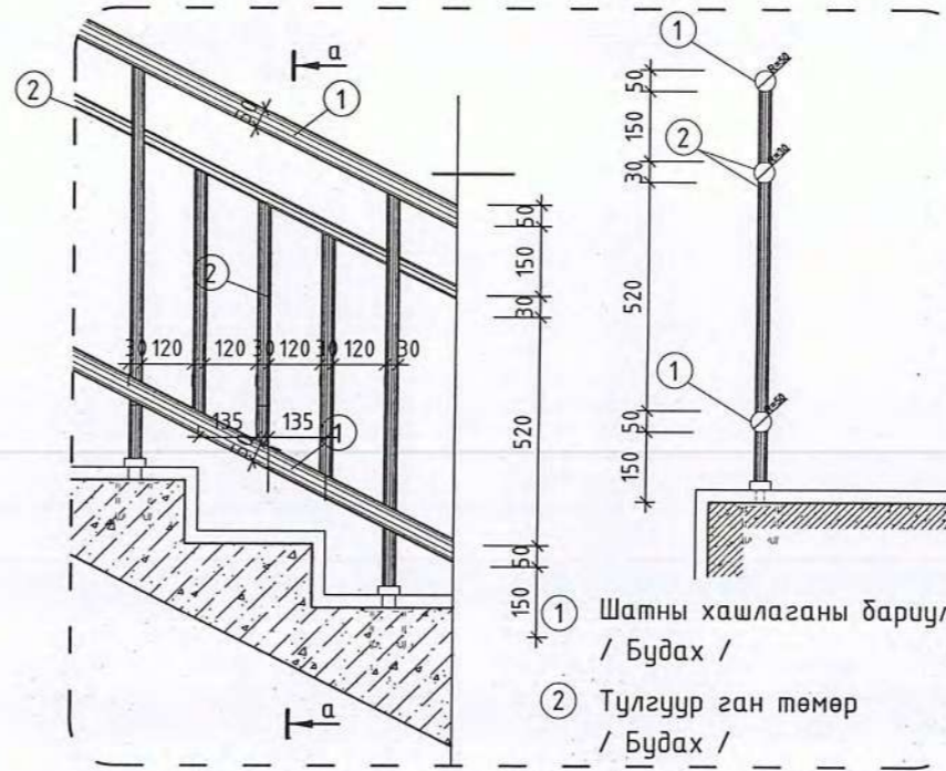
"Огтлол 1-1" М1:20
