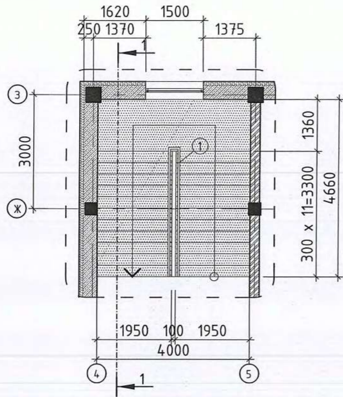
Хэсэгчилсэн байгуулалт М1:100
