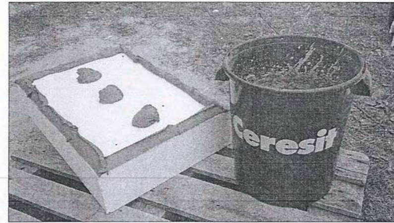
Хөөсөнцөрийн цавууг хөөсөнцөр дээр зөв түрхсэн байдал. Ингэж түрхэх нь хөөсөнцөр хавтангийн араар агаар сийгэх замыг хааж байдаг.
