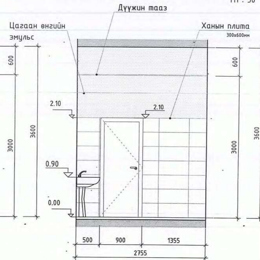
Ханын дэлгээс-2 /Эмэгтэй ариун цэврийн өрөө/ М1 : 50
