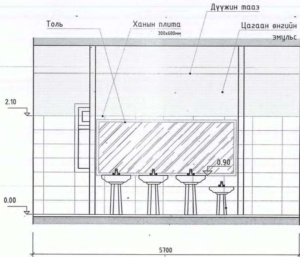
Ханын дэлгээс-1 /Эрэгтэй ариун цэврийн өрөө/
