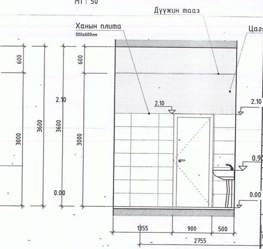
Ханын дэлгээс-2 /Эрэгтэй ариун цэврийн өрөө/
