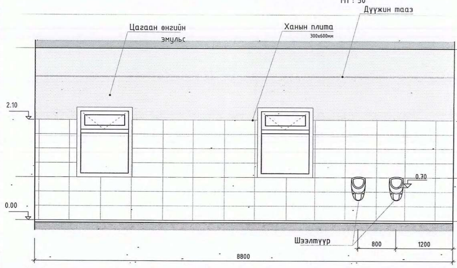
Ханын дэлгээс-3 /Эрэгтэй ариун цэврийн өрөө/
