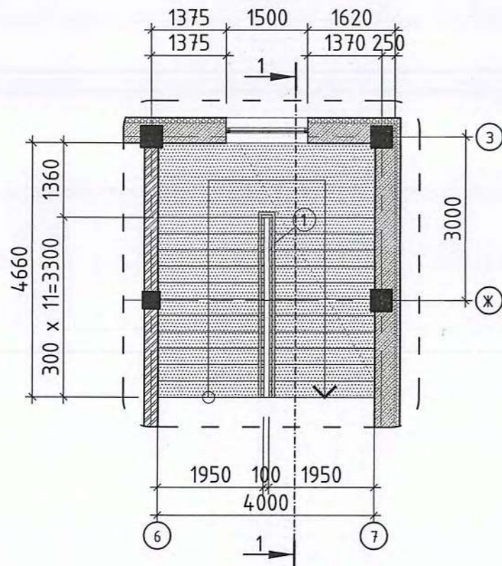
Хэсэгчилсэн байгуулалт М1:100
