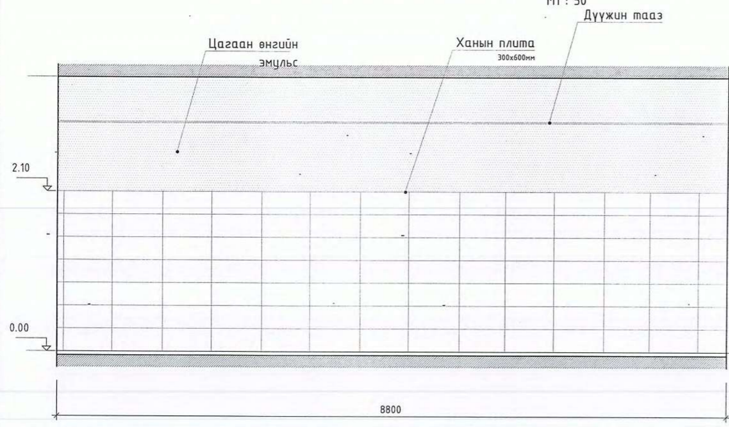
Ханын дэлгээс-3 /Эмэгтэй ариун цэврийн өрөө/
