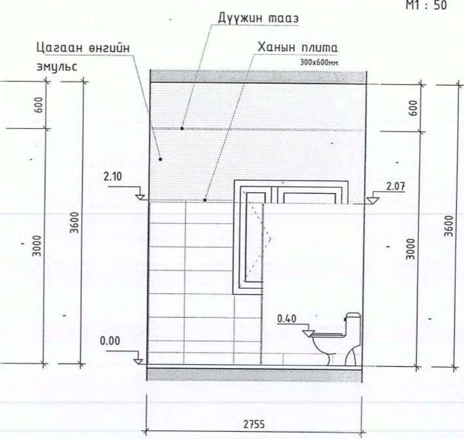
Ханын дэлгээс-4 /Эмэгтэй ариун цэврийн өрөө/
