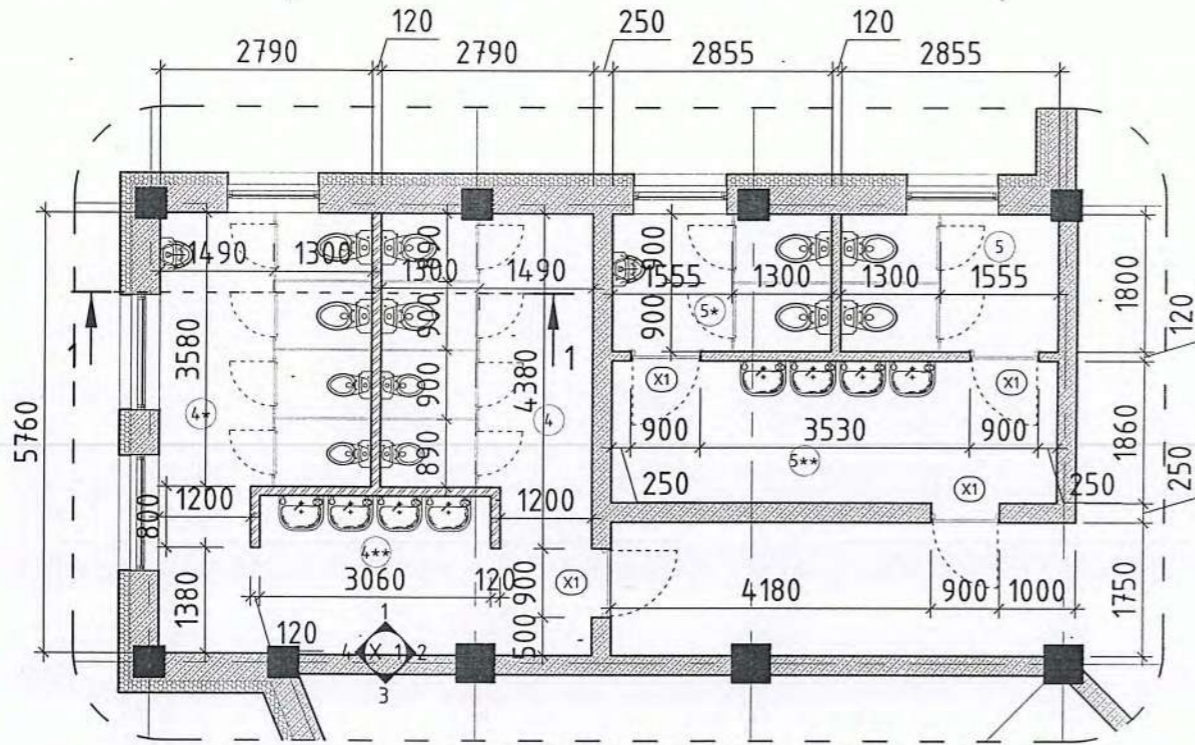
Ханын дэлгээс-1 /Эрэгтэй ариун цэврийн өрөө/
