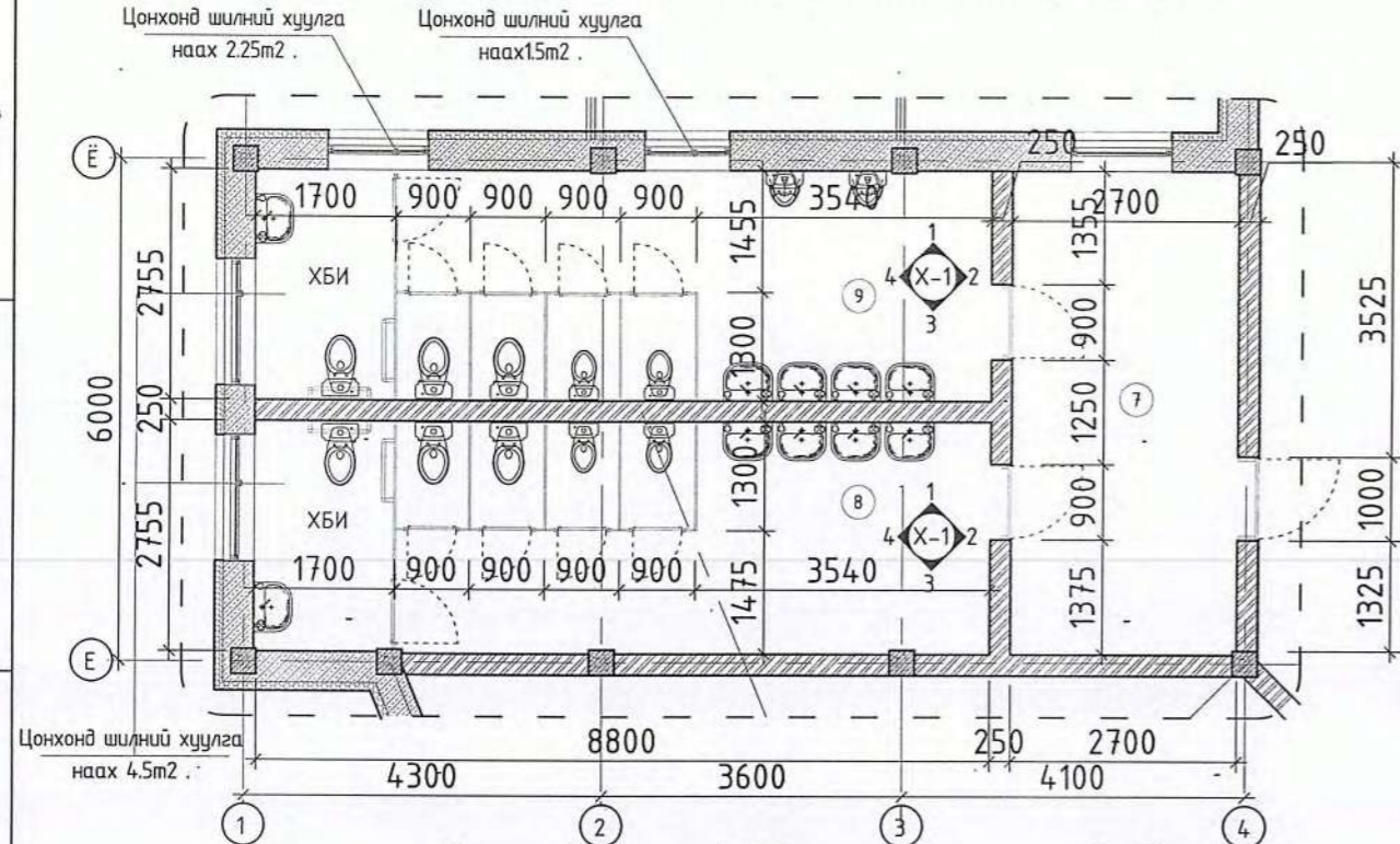
Ханын дэлгээс-1 /Эмэгтэй ариун цэврийн өрөө/ М1 : 50
