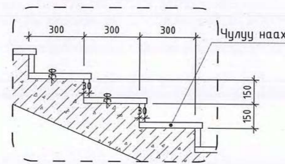
Огтлол а-а М1:20
