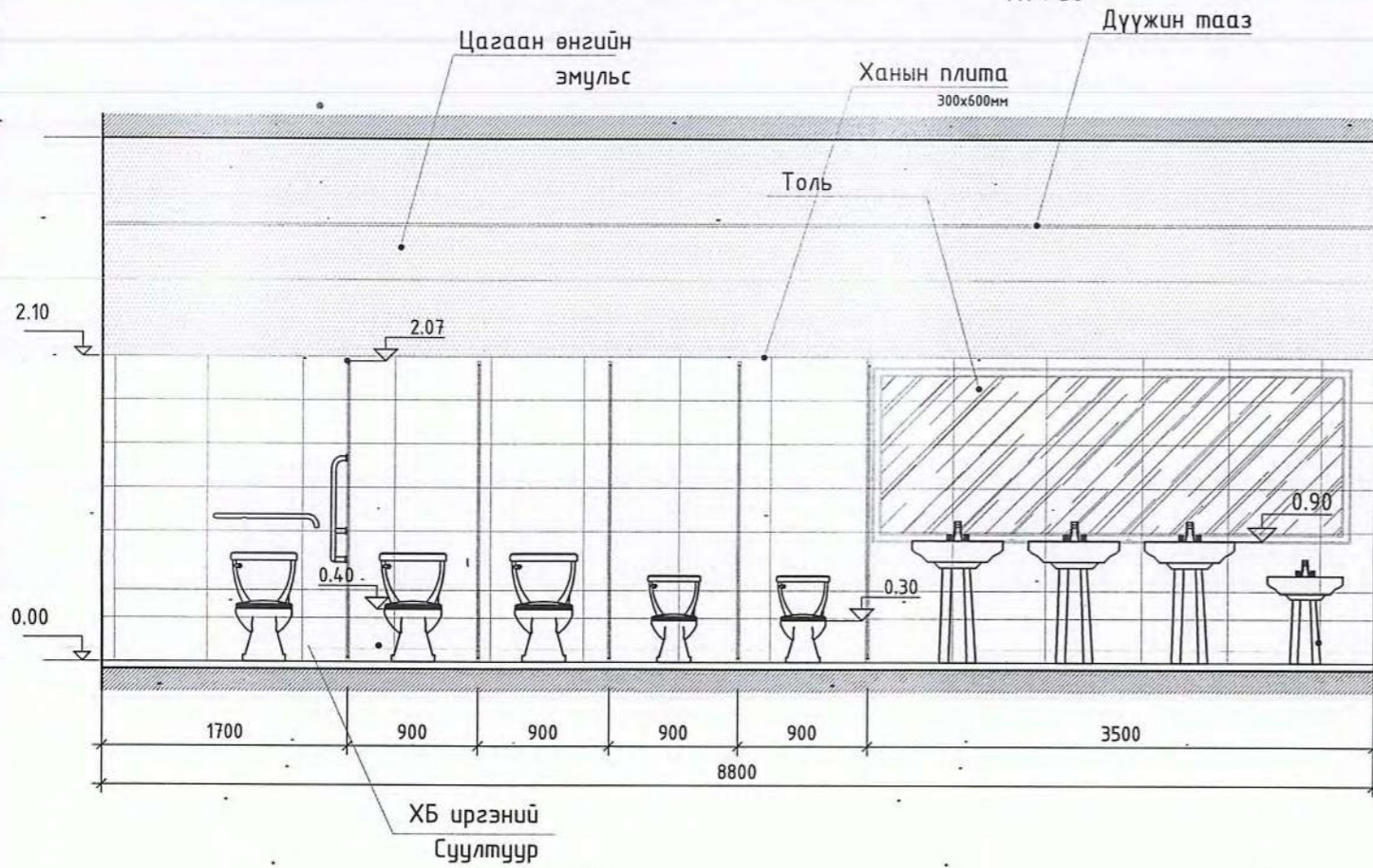
Ханын дэлгээс-1 /Эмэгтэй ариун цэврийн өрөө/ М1 : 50
