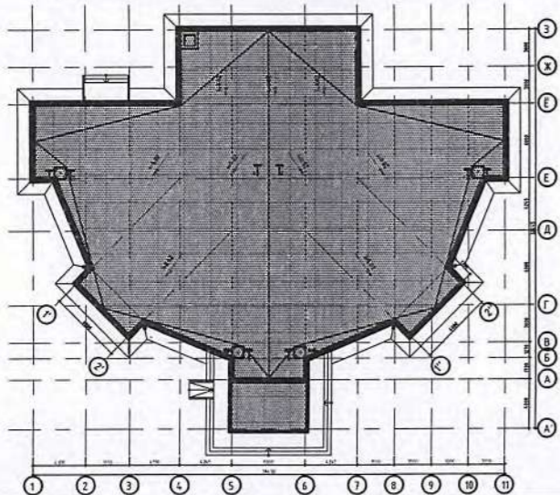
БАРИЛГЫН БҮДҮҮВЧ: М1:500
