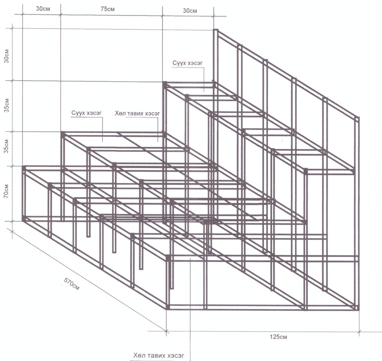
Үзэгчдийн сандалны рамны схем зураг - 1
