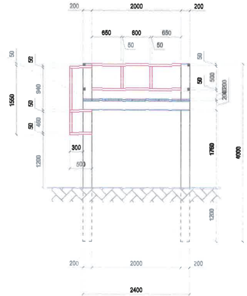
Огтлол 1-1 М1:50
