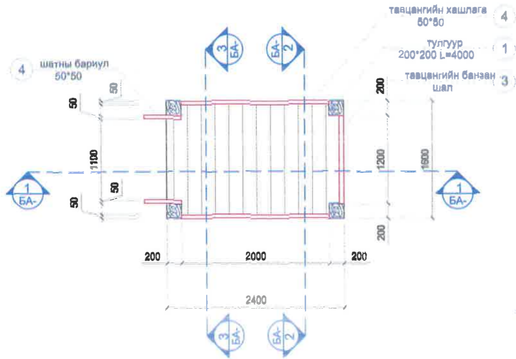
Хяналтын тавцангийн байгуулалт М1:50
