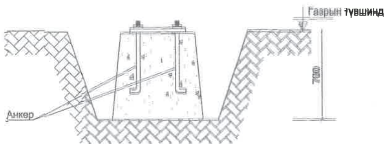
Гэрэлтүүлэг суулгах суурь
