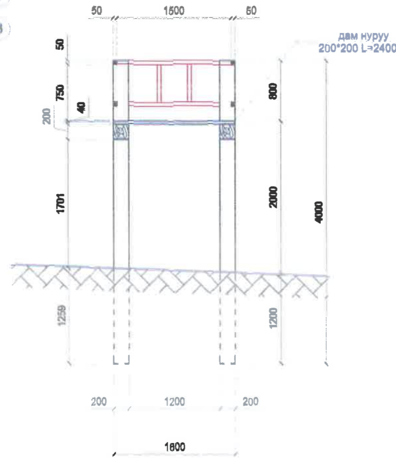
Огтлол 2-2 М1:50
