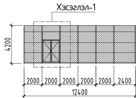
ОГТЛОЛ D-D М1:250
