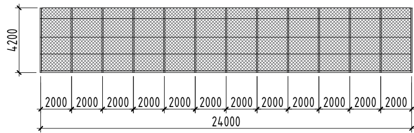
ОГТЛОЛ В-В М1:250
