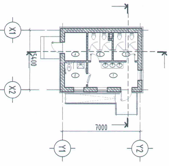
ЕРӨНХИЙ СХЕМ М1:200
