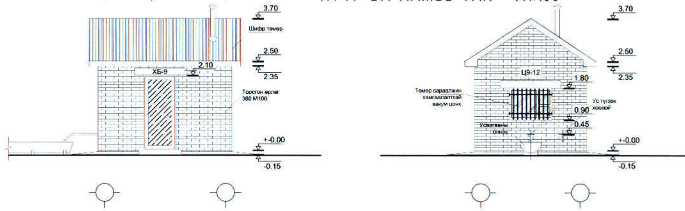
НҮҮР БА ХАЖУУ ТАЛ M1:100
