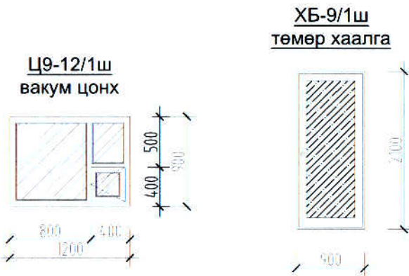
Цонх, хаалга M1:50
