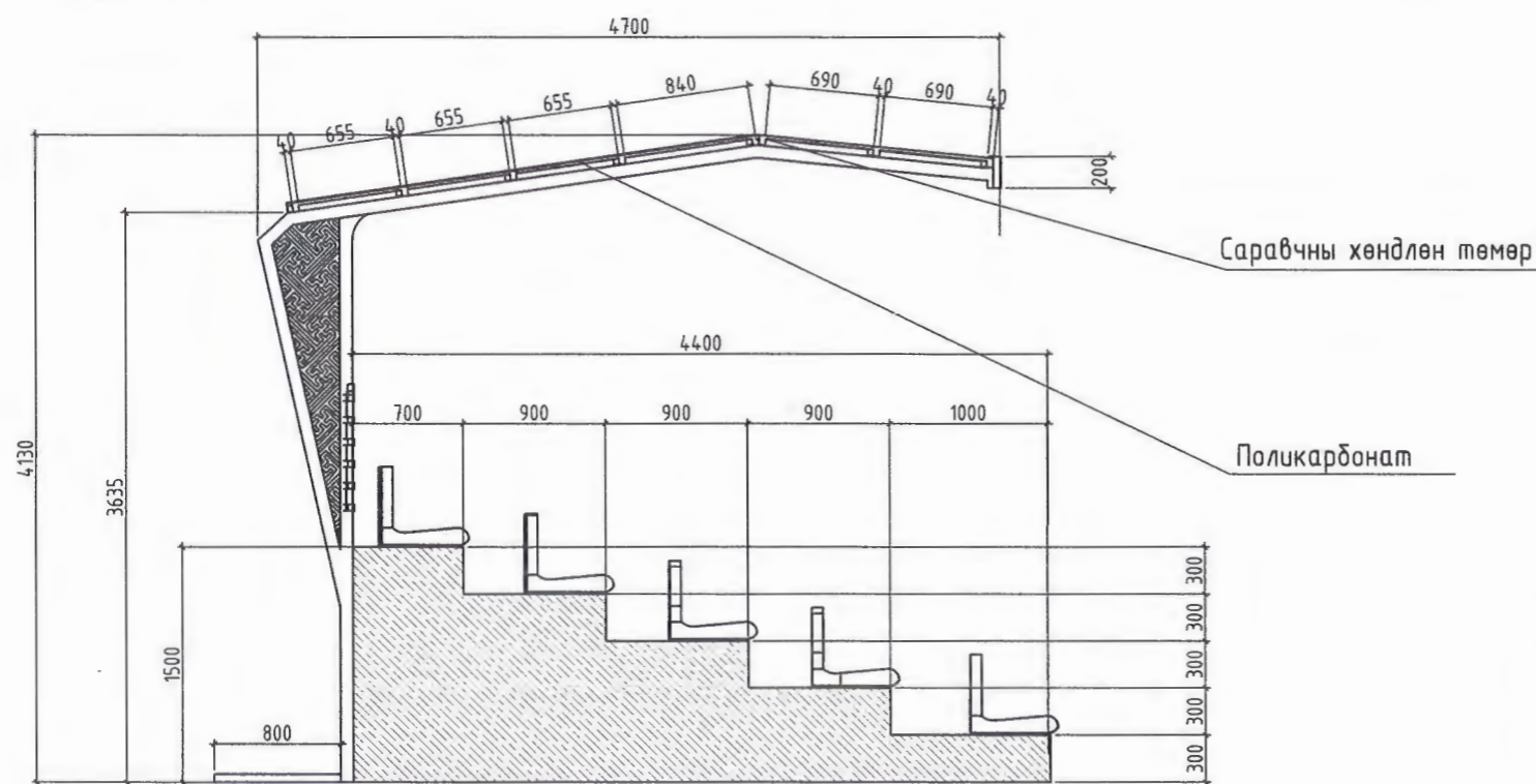
Хажуу огтлол M1:100
