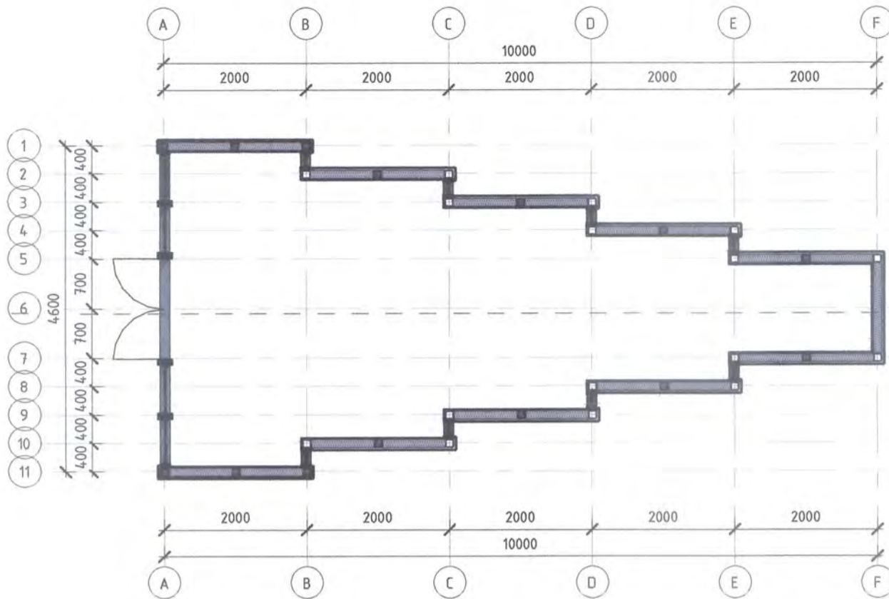
Байгуулалт M:1 : 75
