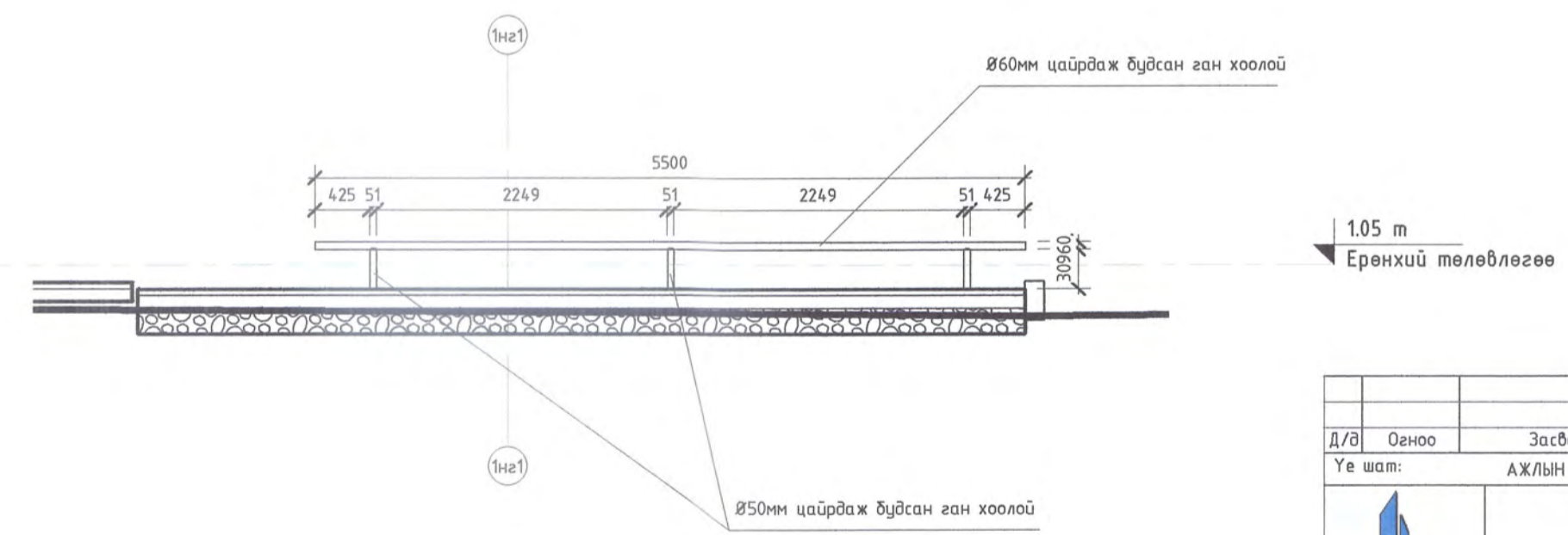
Огллол А-А М 1 : 50
