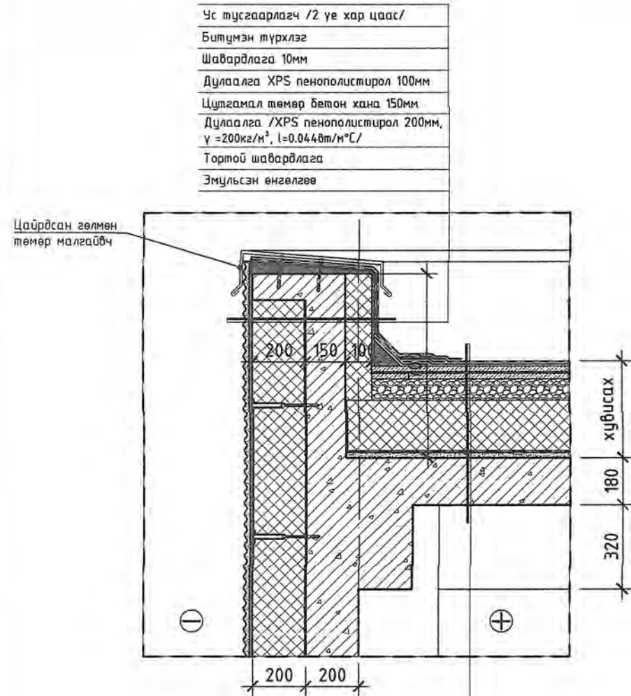
ХЭСЭГ ЛЭЛ - 7 M1:20
