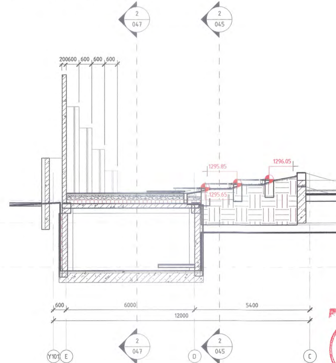
Задгай театр огтлол А М 1 : 100
