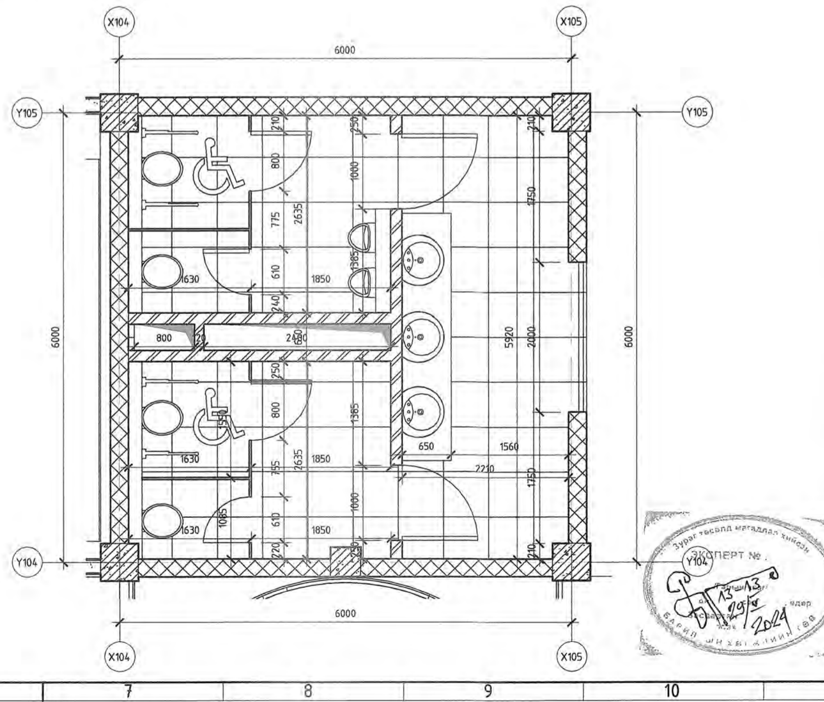
2-р давхрын хэсэгчилсэн байгуулалт 2 М: 1 : 50
