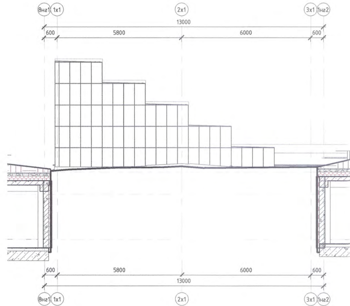
Орц 1 нүүр тал М 1 : 100
