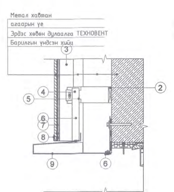
1 Цонх сүх хэсгэлэл M: 1 : 10
