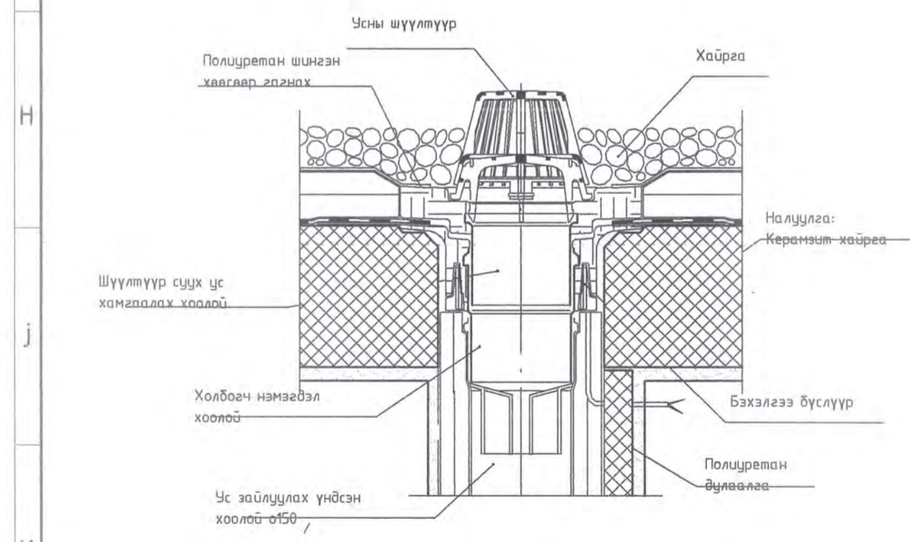
Борооны цсны хаялга M: 1 : 10
