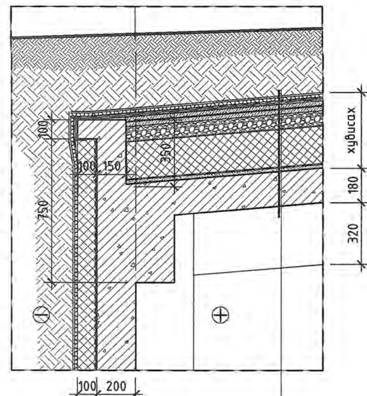
ХЭСЭГ ЛЭЛ - 13 M1:20
