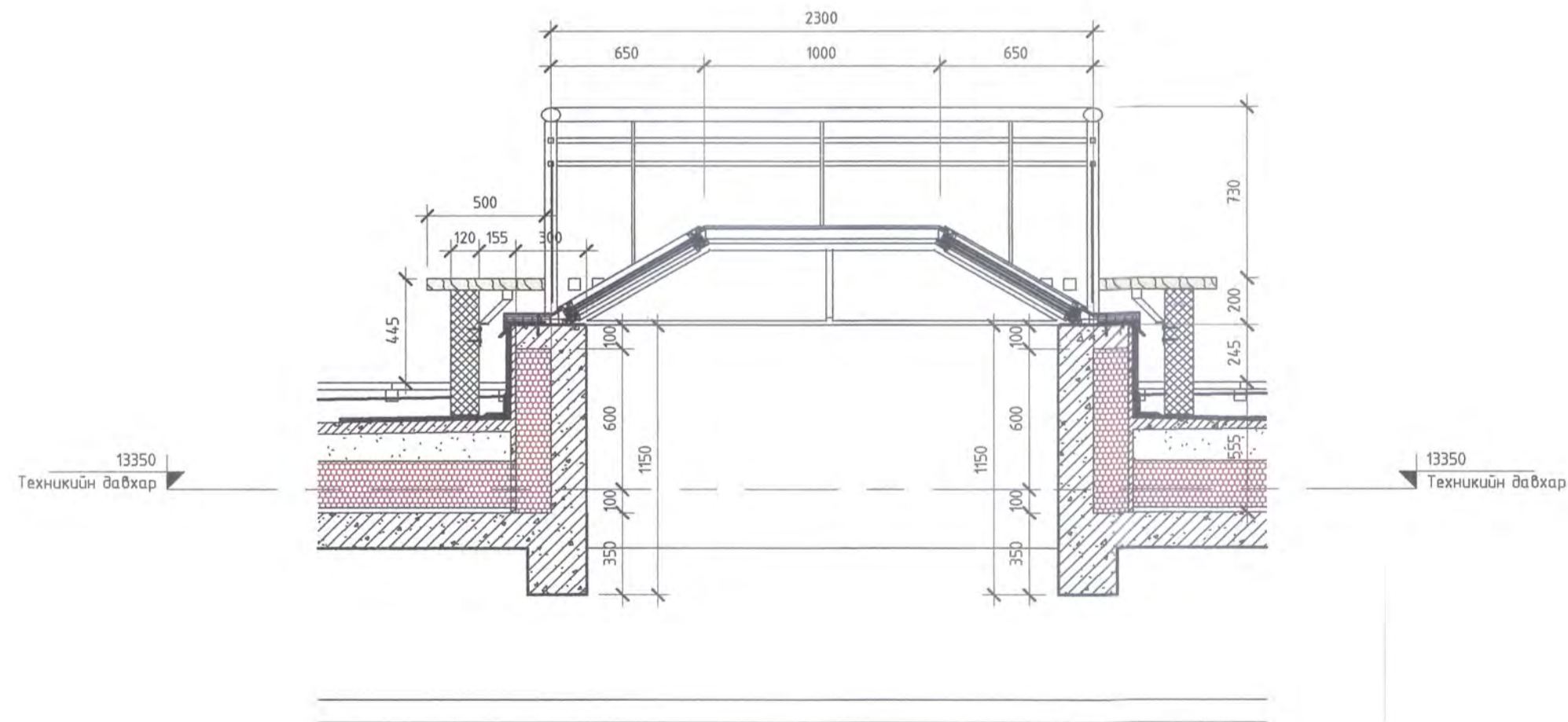
2 Section 5-5 - Callout 2 M: 1 : 25
