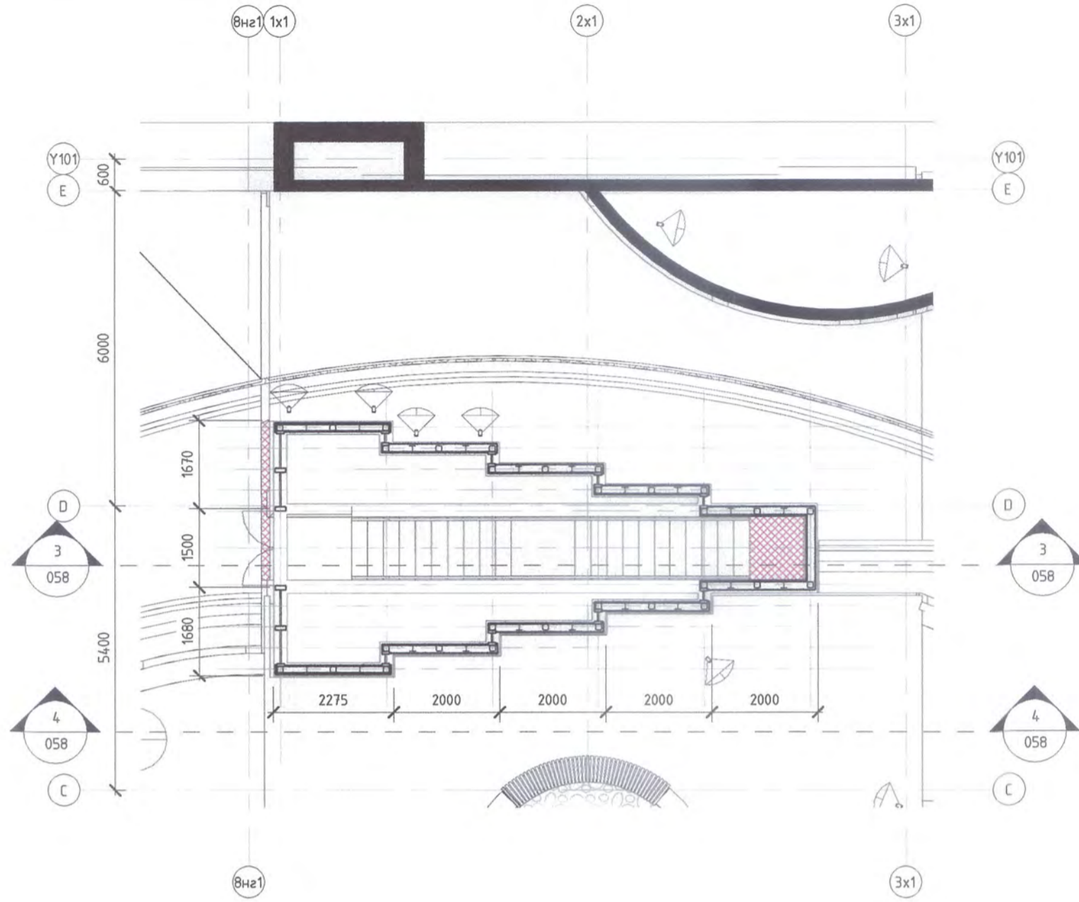
Авто зогсоолын галын гарц 1 М 1 : 100
