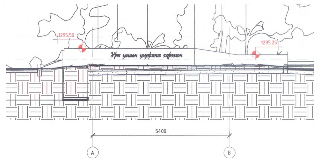
Хаяг байршлын ханын нүүр тал М1 : 75
