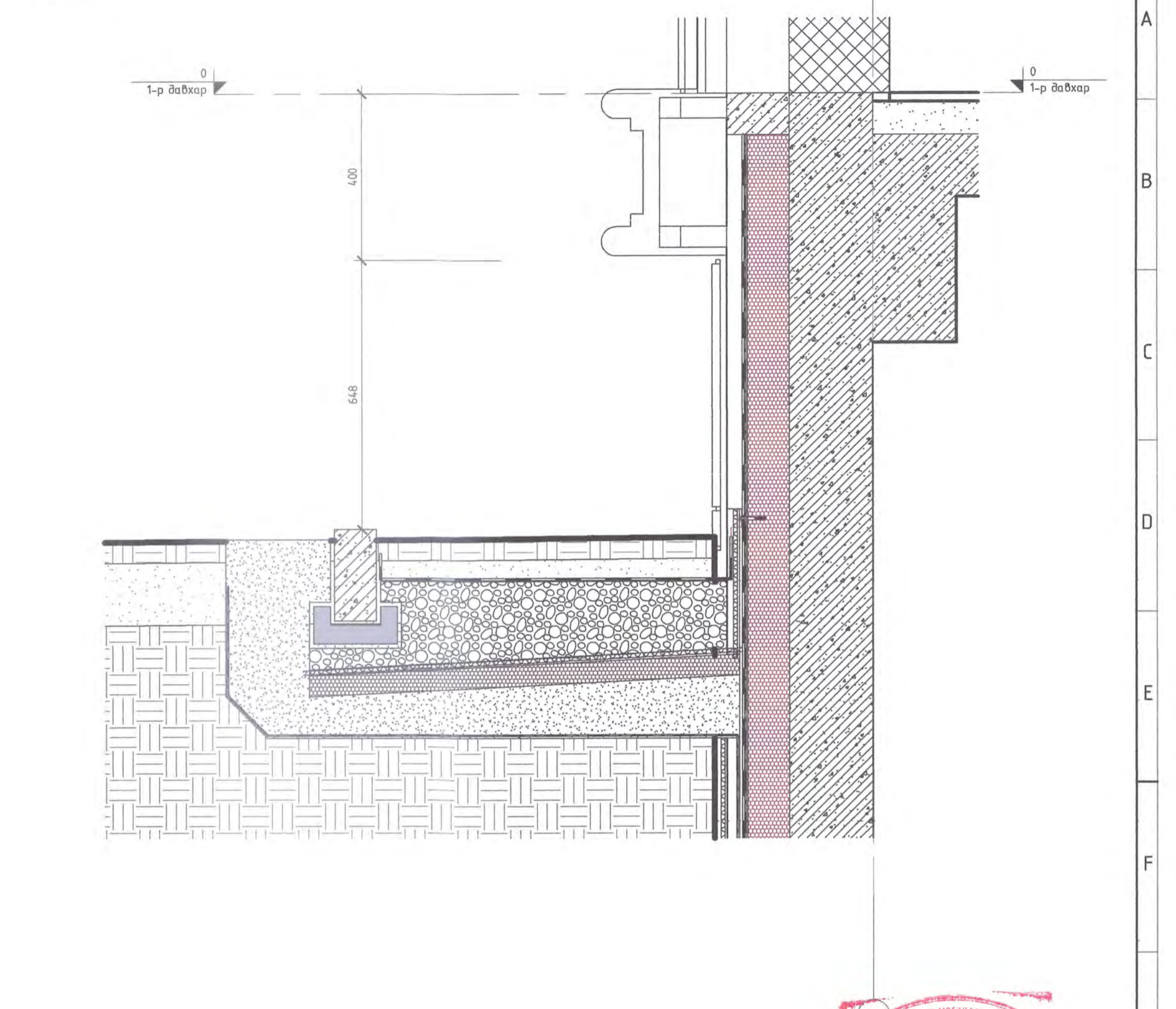
5 Section 5-5 - Callout 6 M: 1 : 10
