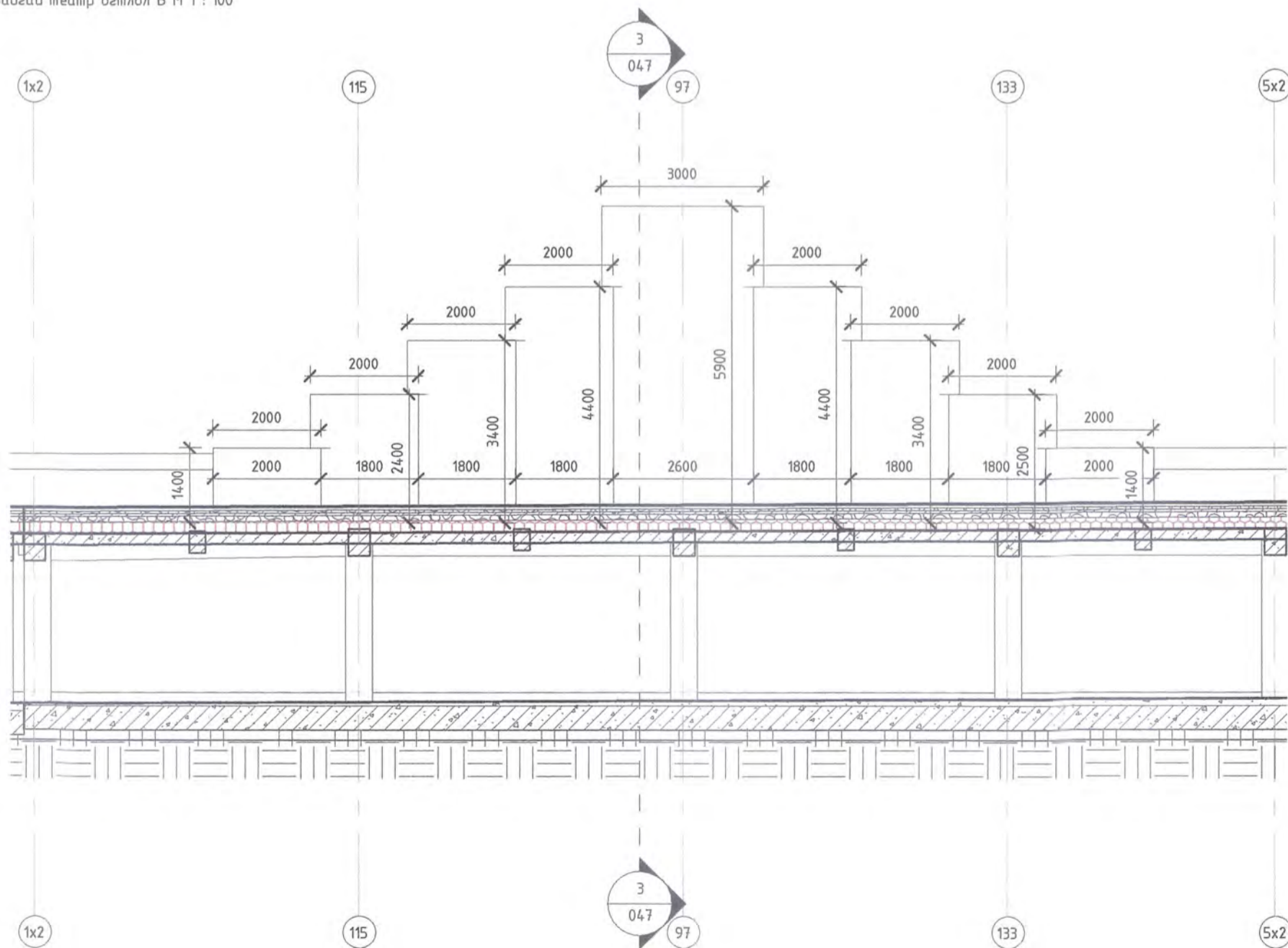
Задгай театр огтлол Б М 1 : 100
