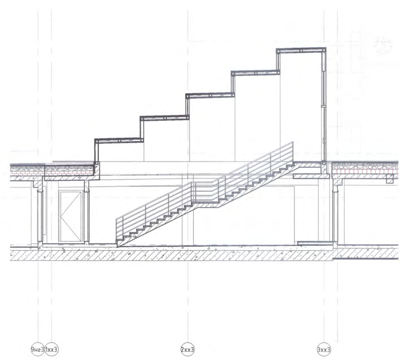
Орц 2-А М 1 : 100
