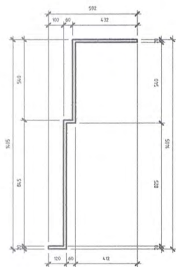
08_Ашиглалттай дээврийн парпетний хүрээ М: 1 : 25
