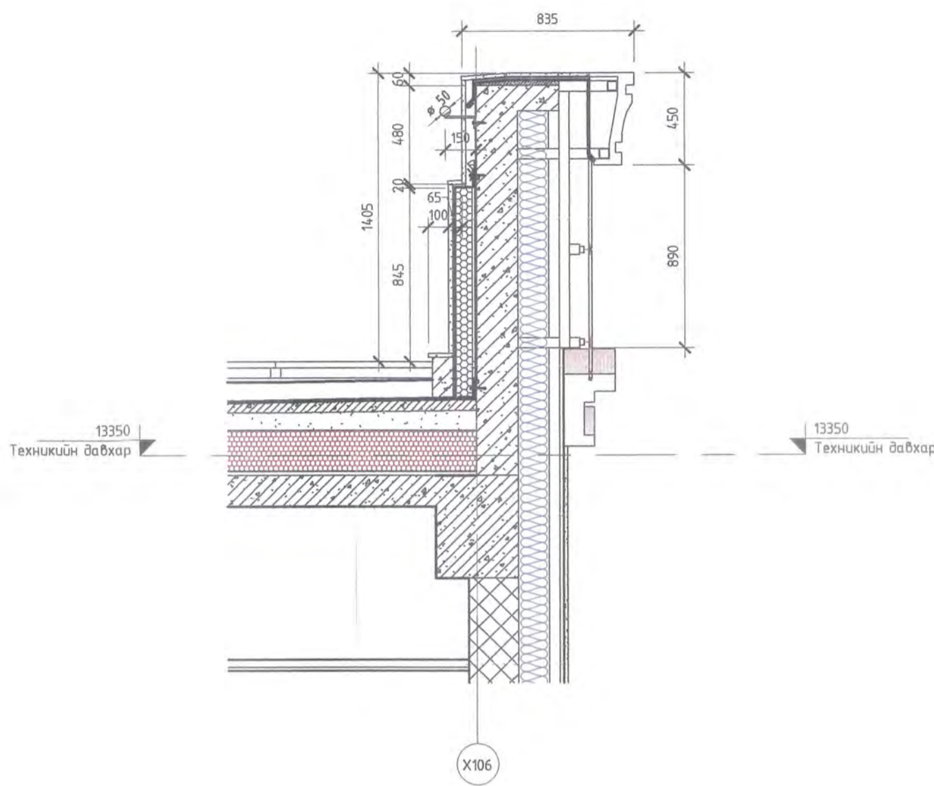
4 Section 2-2 - Callout 2 M: 1 : 25
