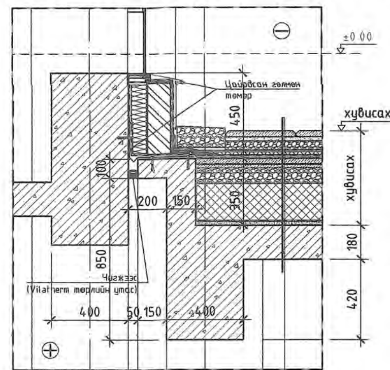
ХЭСЭГ ЛЭЛ - 11 M1:20
