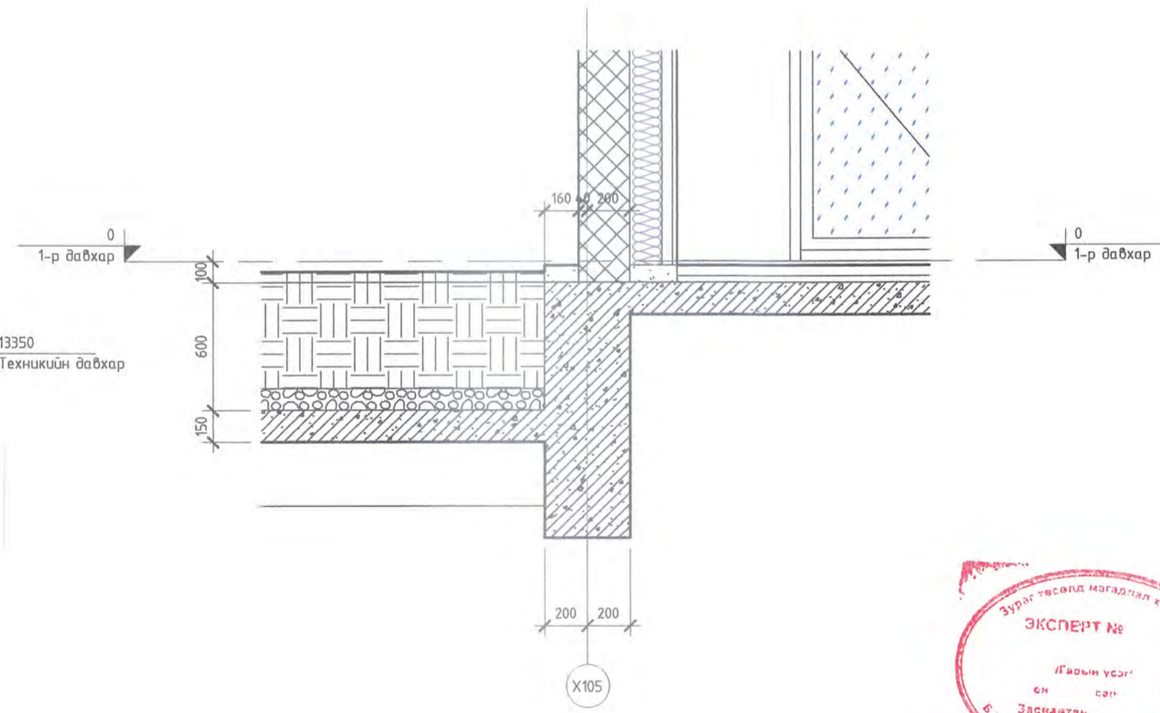
1 Section 1-1 - Callout 1 M: 1 : 25
