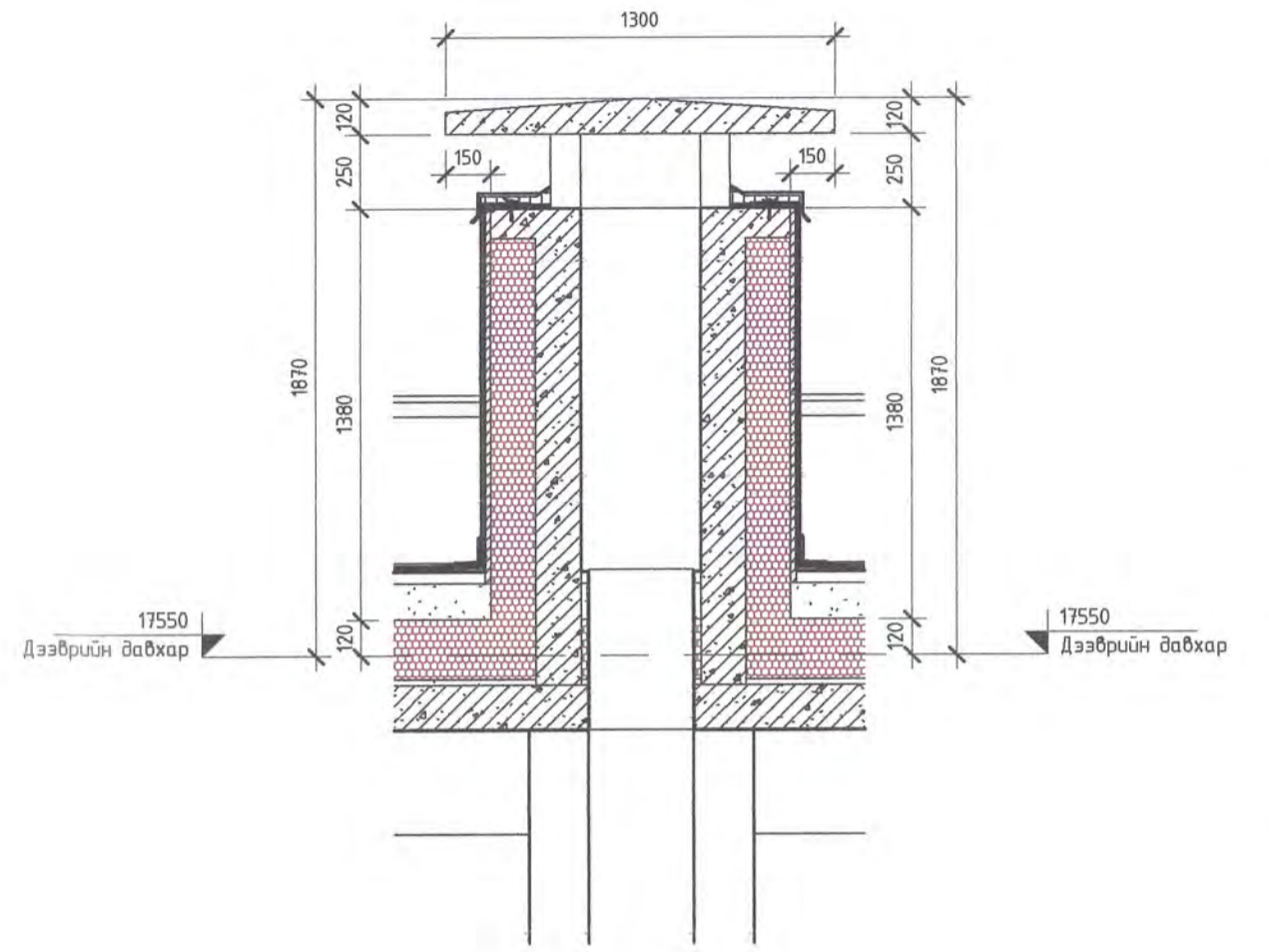
5 Section 5-5 - Callout 5 M: 1 : 25
