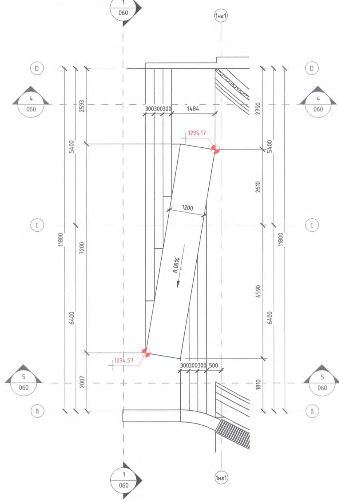
Тохжилтын шат А1 М1 : 75
