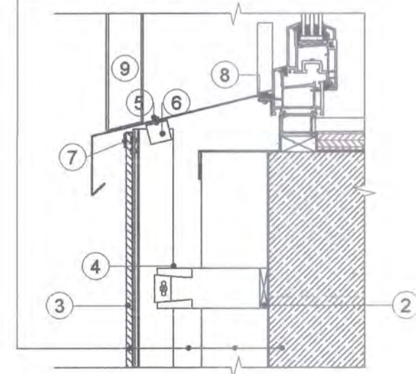
Метал хавтан агаарын үе Эрдэс хөвөн дулаалга ТЕХНОВЕНТ Барилгын үндсэн хийц
