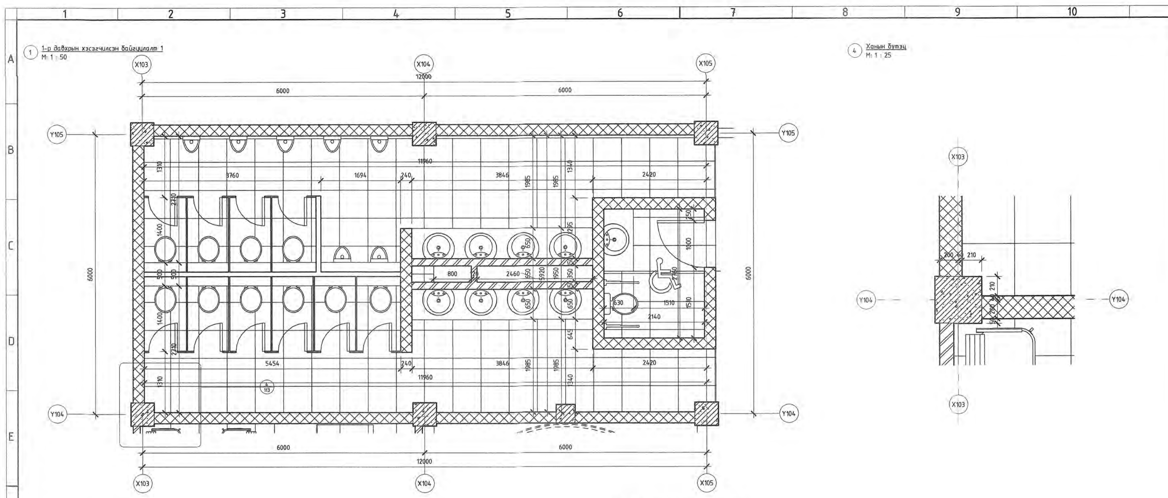
2-р давхрын хэсэгчилсэн байгуулалт 2 М: 1 : 50
