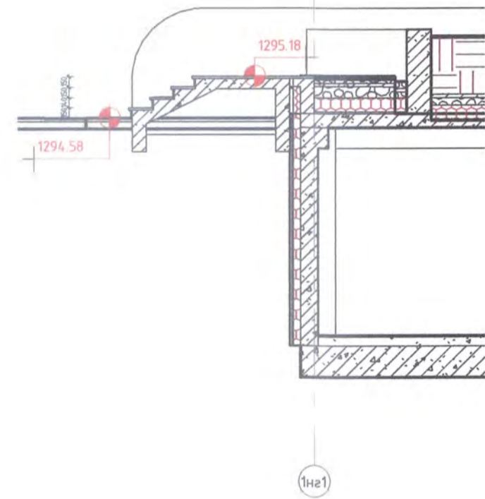
Огтлол А1-3 М1 : 75
