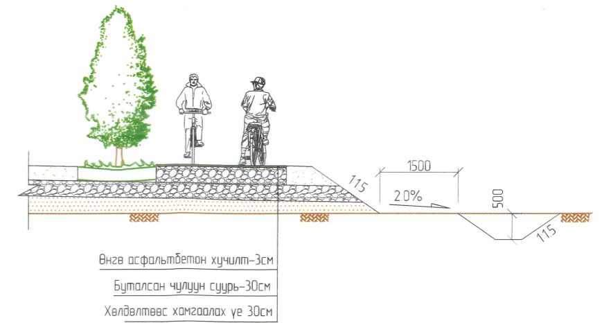
Дугуйн замын хучилтын хийц
