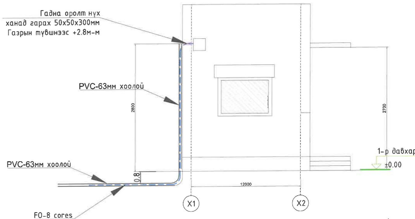
FO-8 cores
