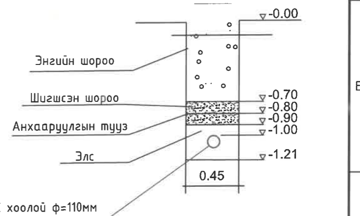
РВС ХООЛОЙТОЙ СУВАГЧЛАЛЫН ОГТЛОЛ А-А
