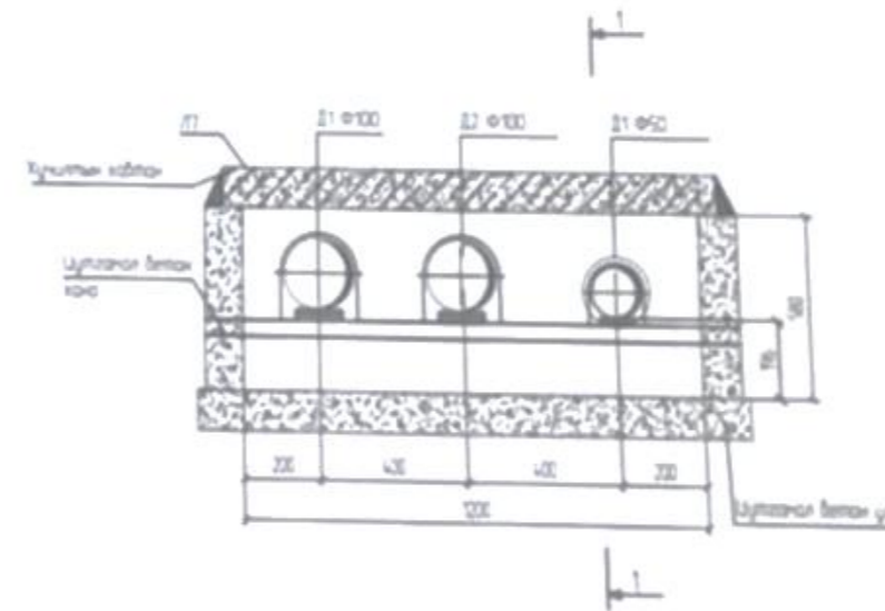
ҮЛ ХӨДЛӨХ ТУЛГУУР / ҮХТ-1/ М1:20
