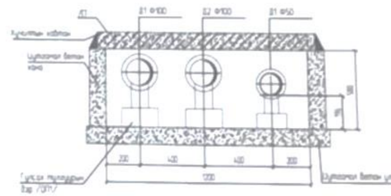
ҮЛ ХӨДЛӨХ ТУЛГУУР / ҮХТ-1/ М1:20
