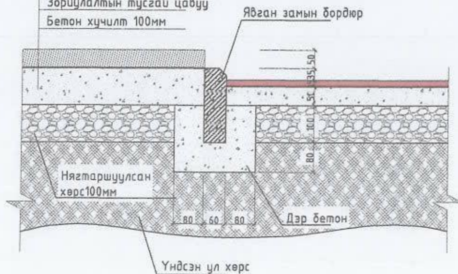
ОГТЛОЛ 1-1 М1:10
