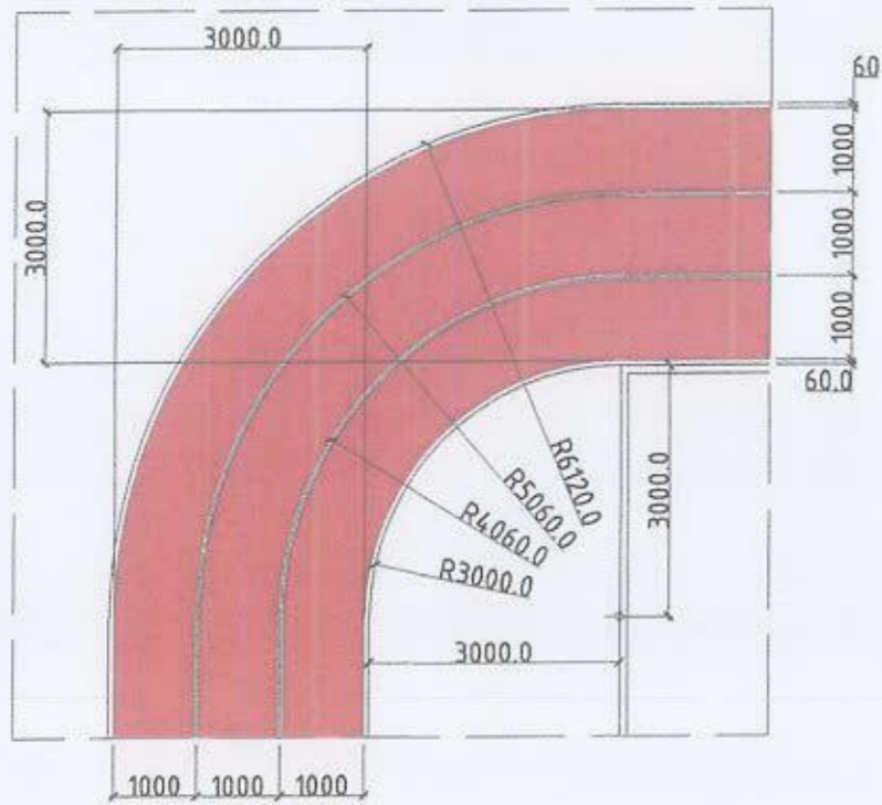
ХЭСЭГЛЭЛ М1:100
