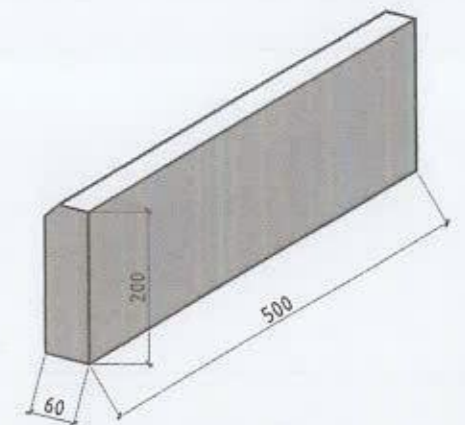
ЗАМЫН БОРДЮРЫН ЖИШЭЭ ЗУРАГ
