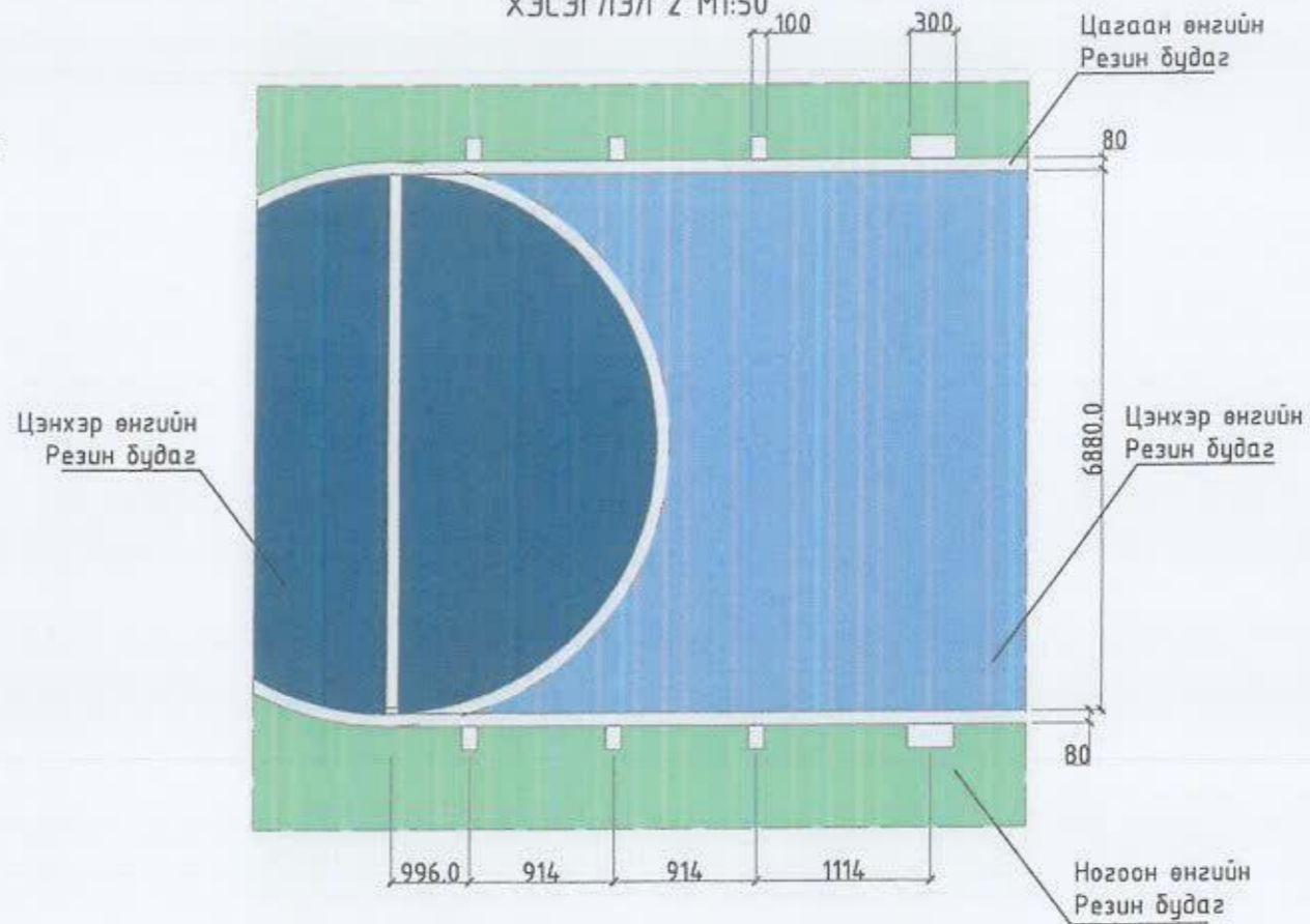
ХЭСЭГЛЭЛ 2 М1:50
