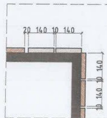
ХЭСЭГЛЭЛ 1 М1:12.5
