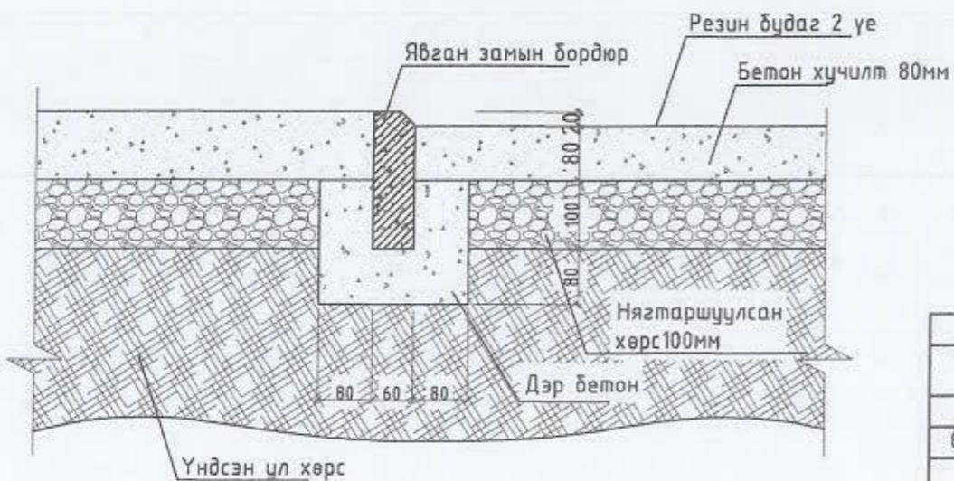
ОГТЛОЛ М1:10
