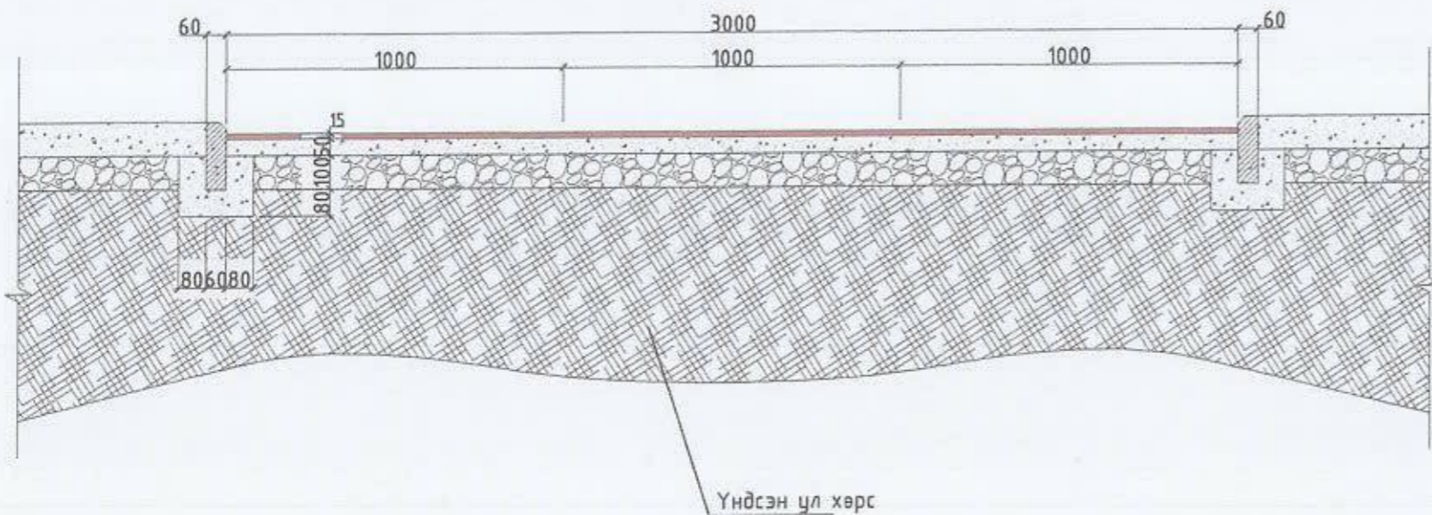
ОГТЛОЛ 1-1 М1:25
