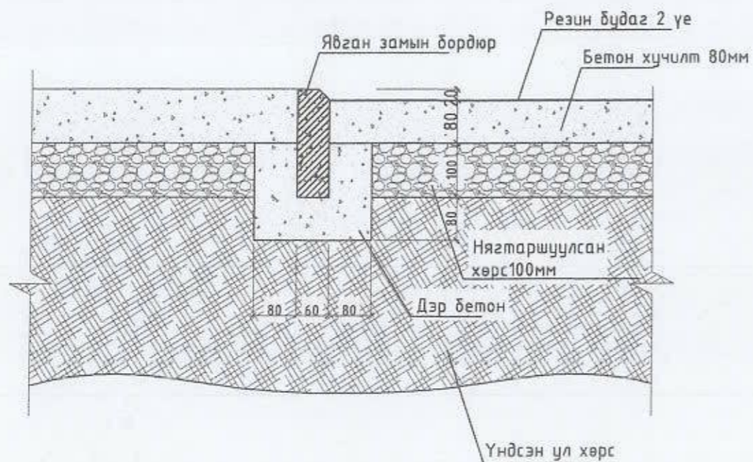
ОГТЛОЛ 1-1 М1:10
